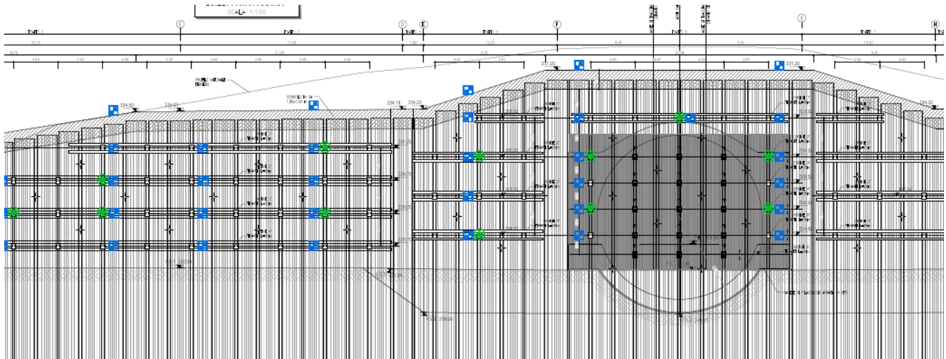
Figura 3-2. Stralcio del monitoraggio paratia: posizionamento delle mire ottiche (blu) e delle celle di carico toroidali (verdi)
