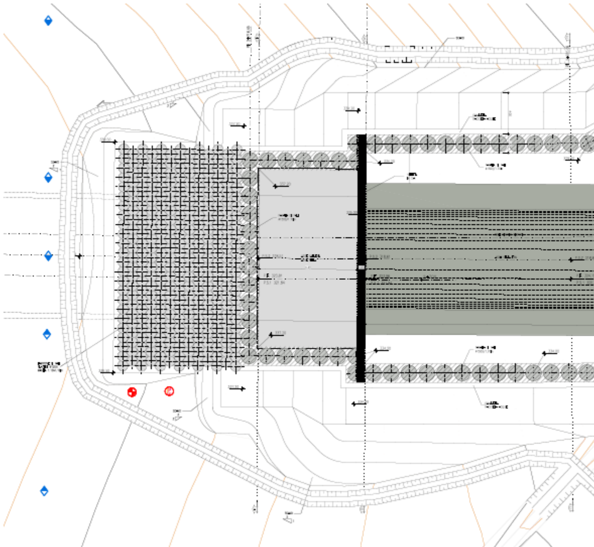
Figura 3-1 – Posizionamento capisaldi (in blu) e inclinometri e piezometri (in rosso)
