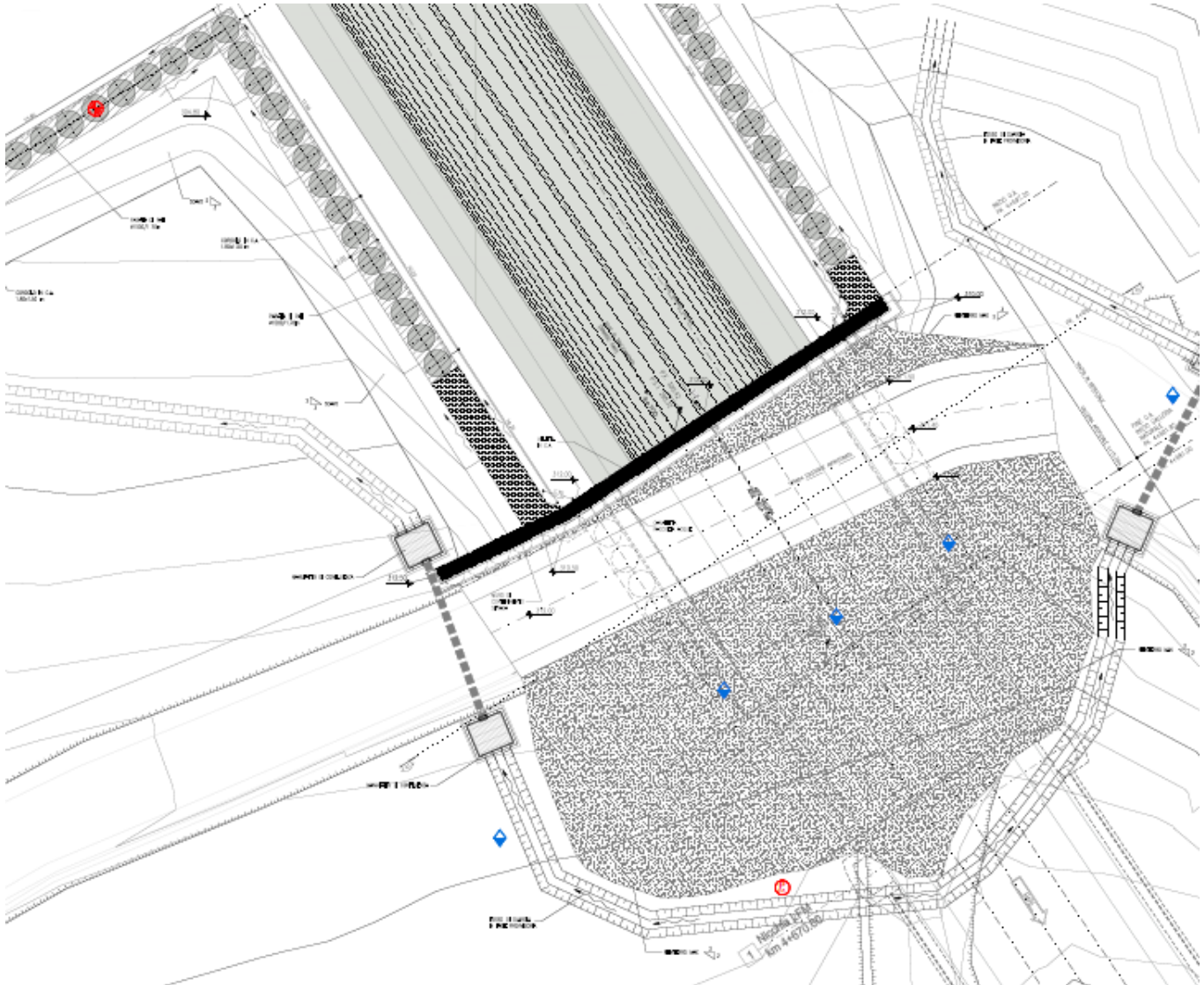
Figura 3-1 – Esempio di posizionamento di capisaldi (in blu), inclinometri e piezometri (in rosso)
