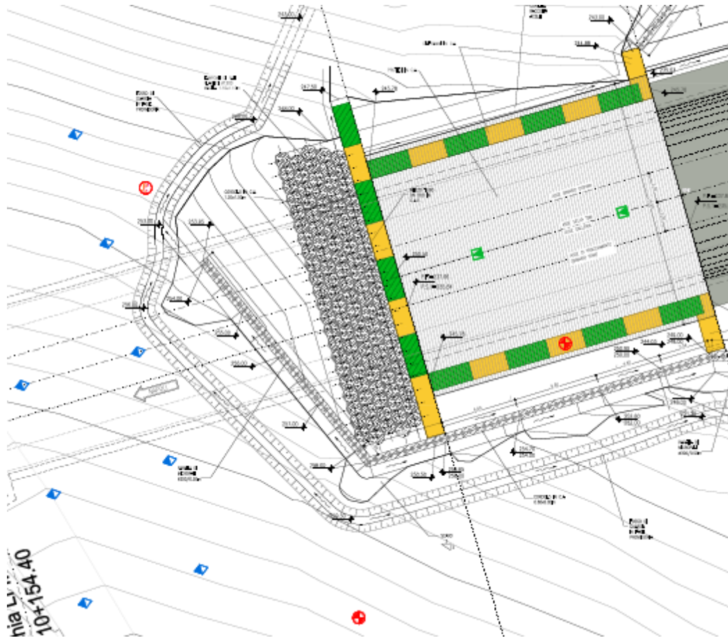
Figura 3-1 – Posizionamento capisaldi (in blu), inclinometri e piezometri (in rosso), barrette estensimetriche (in verde)
