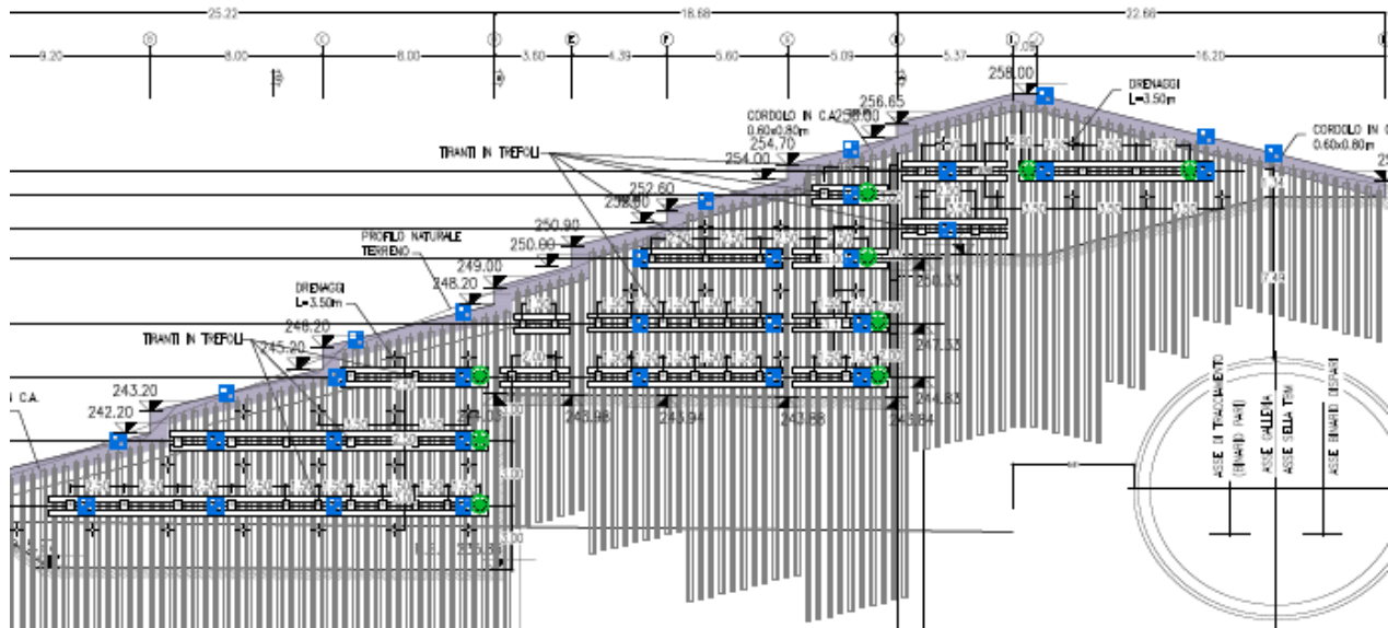
Figura 3-2. Monitoraggio paratia: posizionamento delle mire ottiche (blu) e delle celle di carico toroidali (verdi)
