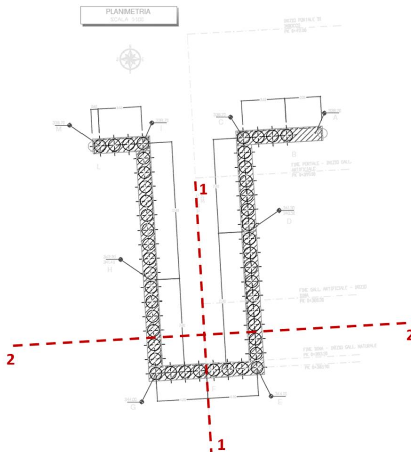
Figura 3-3. Sezioni di calcolo
