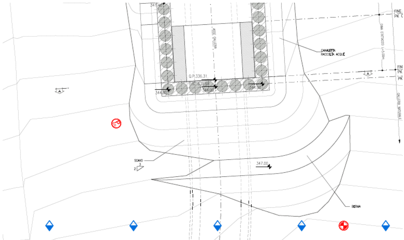
Figura 3-1 – Posizionamento capisaldi (in blu) e inclinometro e piezometro (in rosso)
