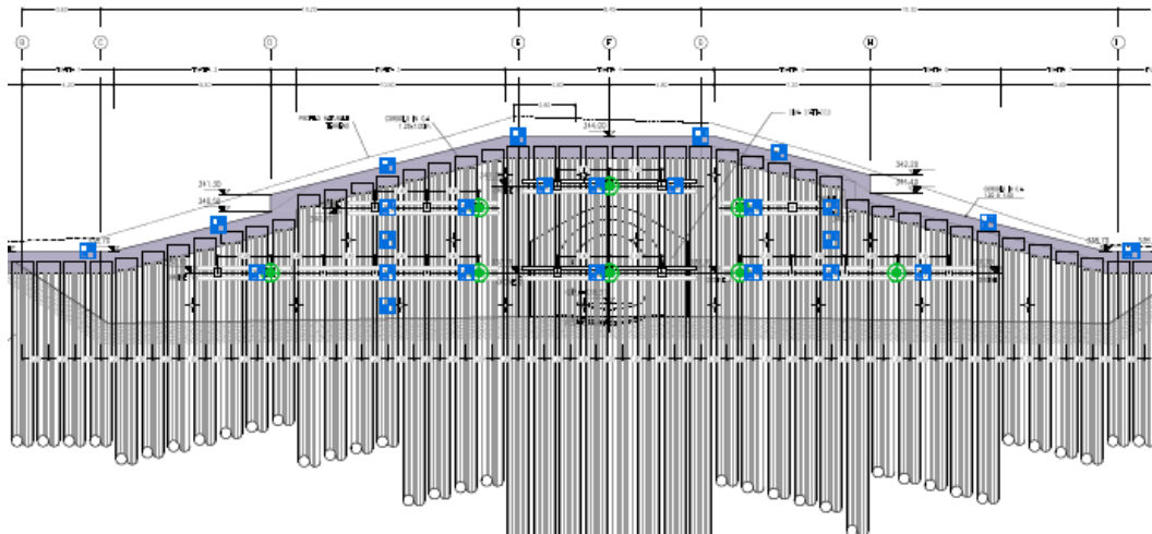
Figura 3-2. Monitoraggio paratia: posizionamento delle mire ottiche (blu) e delle celle di carico toroidali (verdi)
