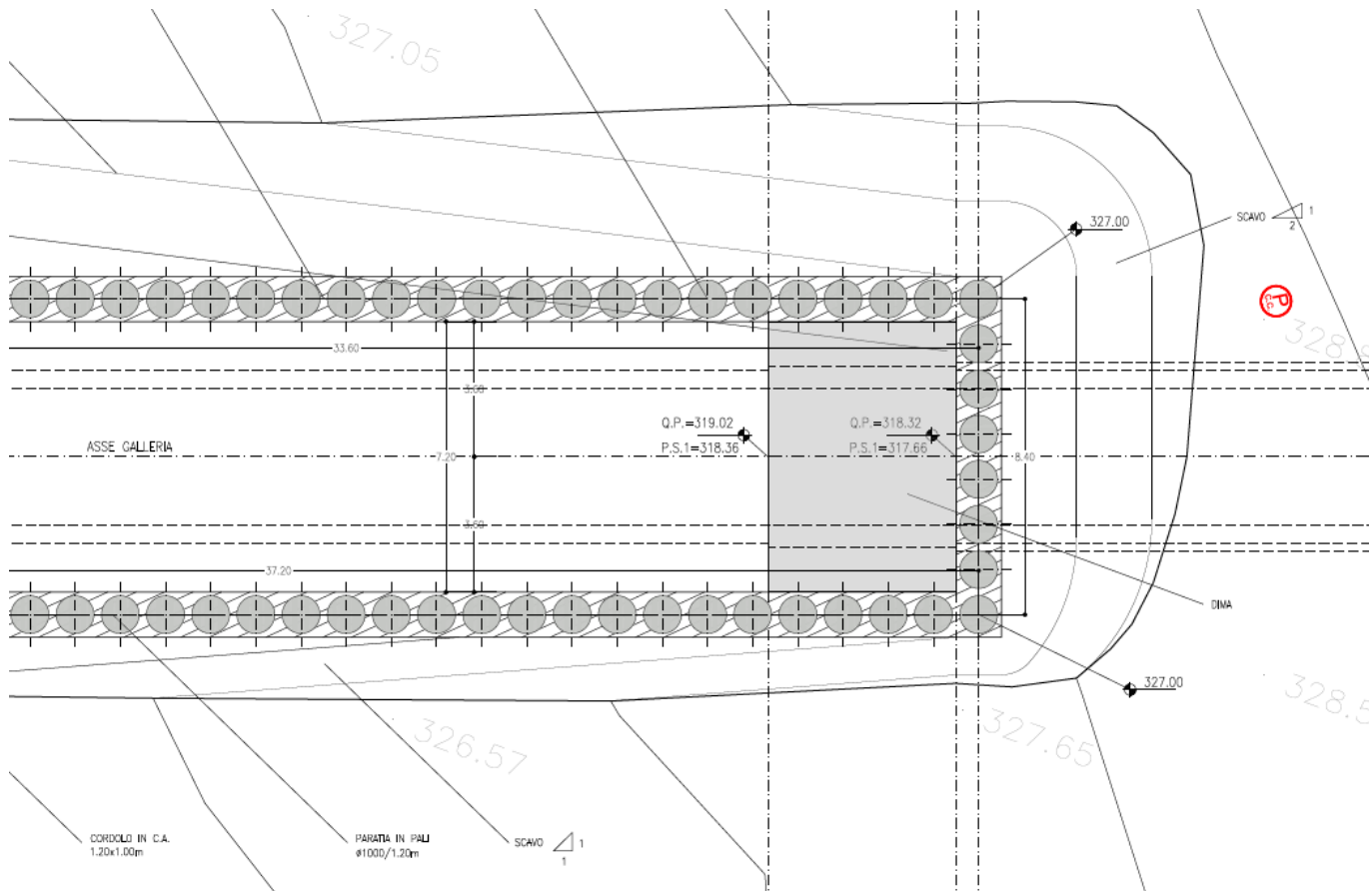
Figura 3-1. Posizionamento piezometro (in rosso)
