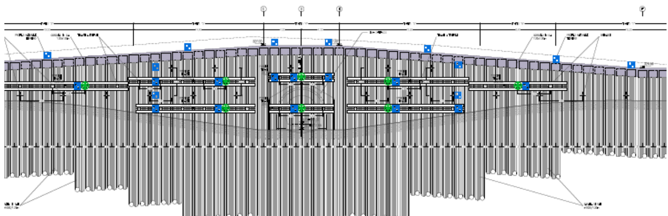
Figura 3-2. Monitoraggio paratia: posizionamento delle mire ottiche (blu) e delle celle di carico toroidali (verdi)
