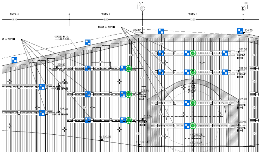
Figura 3-2. Monitoraggio paratia: posizionamento delle mire ottiche (blu) e delle celle di carico toroidali (verdi)
