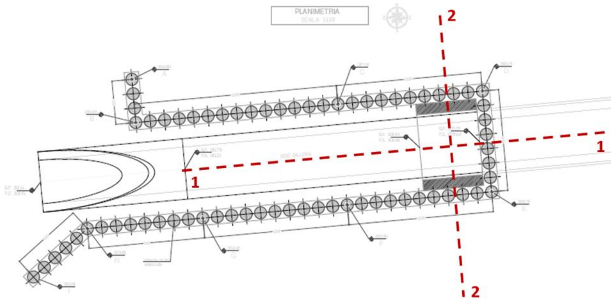
Figura 3-3. Sezioni di calcolo
