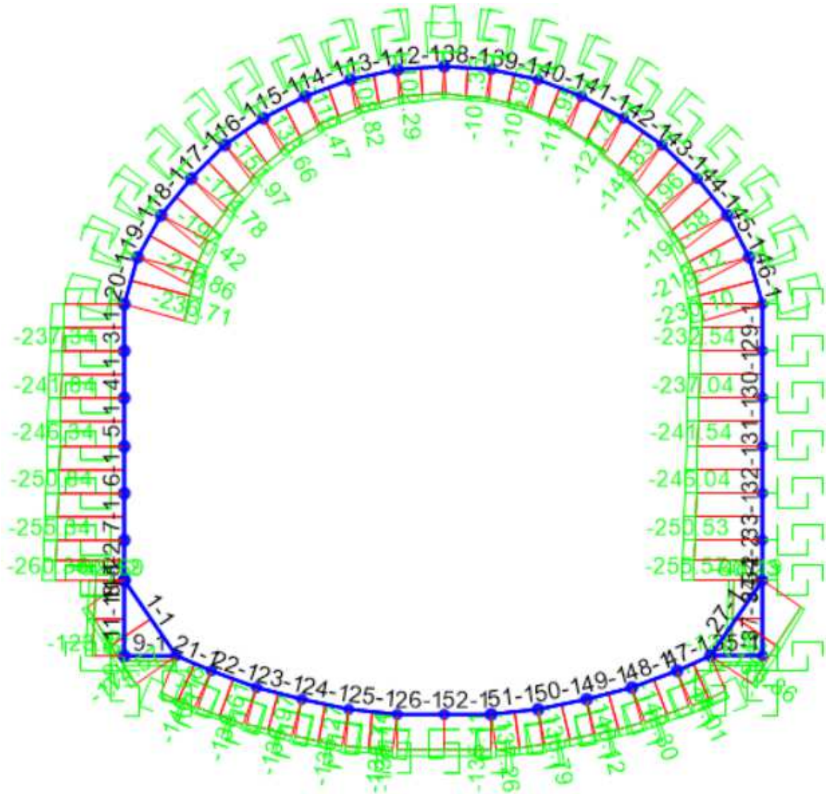
Figura 63 – Diagramma di involuppo dell'azione assiale (INVILUPPO SLE-F)
