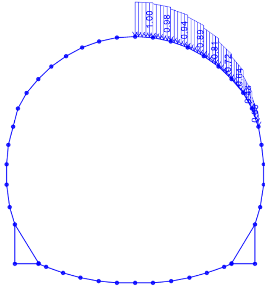
Figura 9 – Carico variabile Q_{d,dx} applicato in copertura sul lato destro
