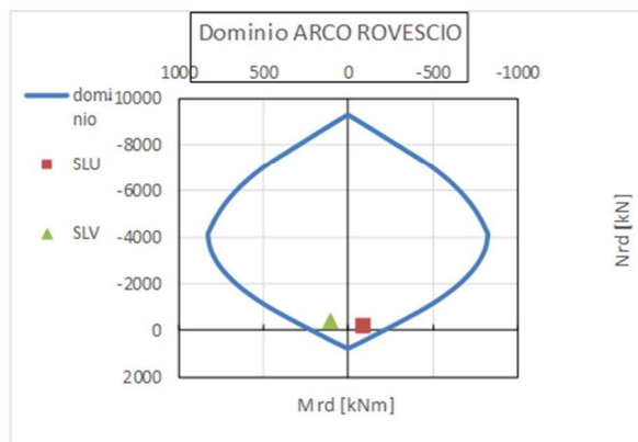
Figura 52 – Domini M-N – SLU
