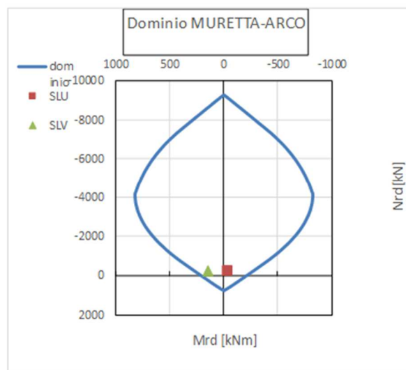
Figura 45 – Domini M-N – SLU
