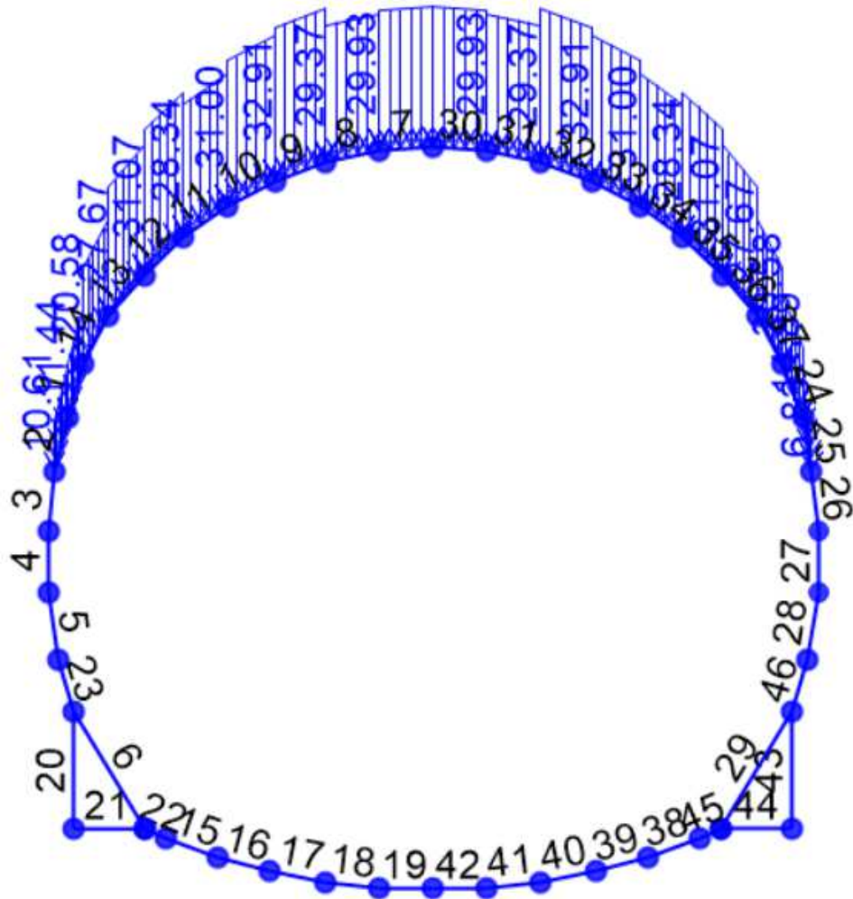
Figura 14 – Carico applicato spinta sismica verticale
