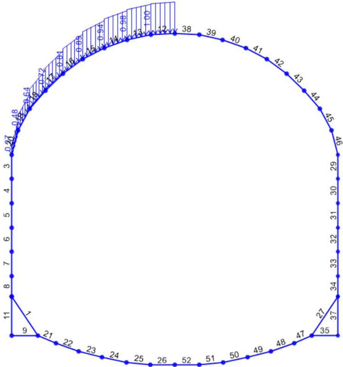
Figura 20 – Carico variabile Q_{d\_sx} applicato in copertura sul lato sinistro
