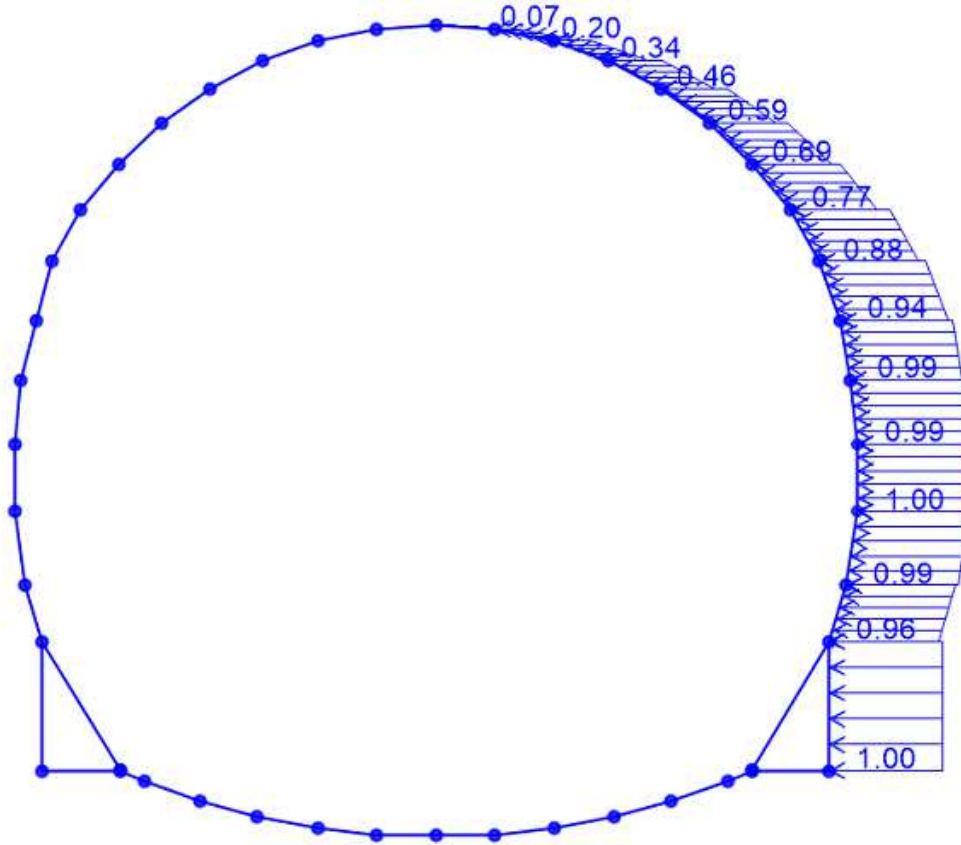
Figura 11 – Sovraccarico laterale SQ.dx sul lato destro, dovuto al carico variabile in copertura (20 kN/m * k 0-dx )
