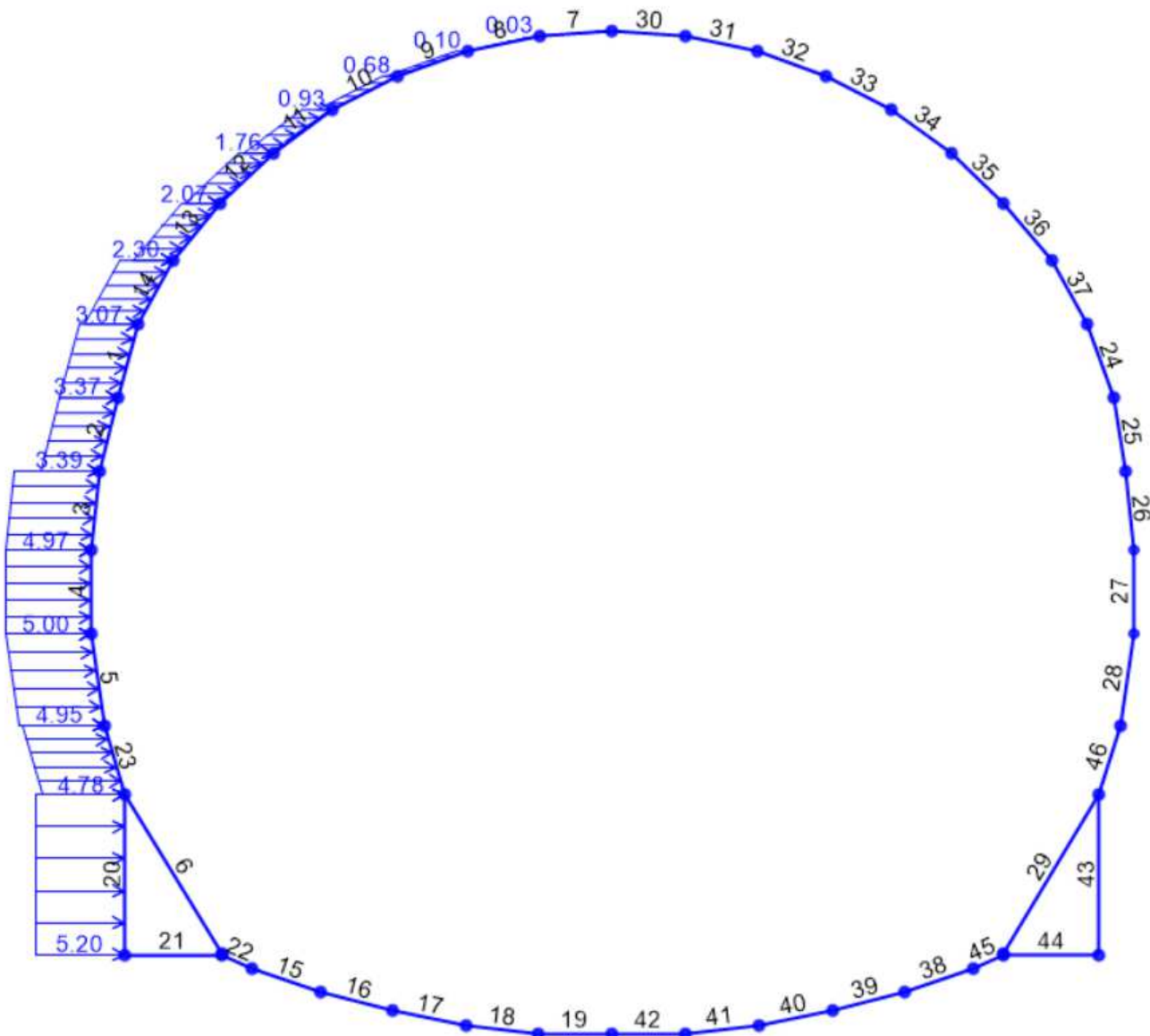
Figura 30 – Carico dovuto alla spinta orizzontale sinistra SP.sx ( K_{osn} * \gamma_{rit} * H_{rit} )
