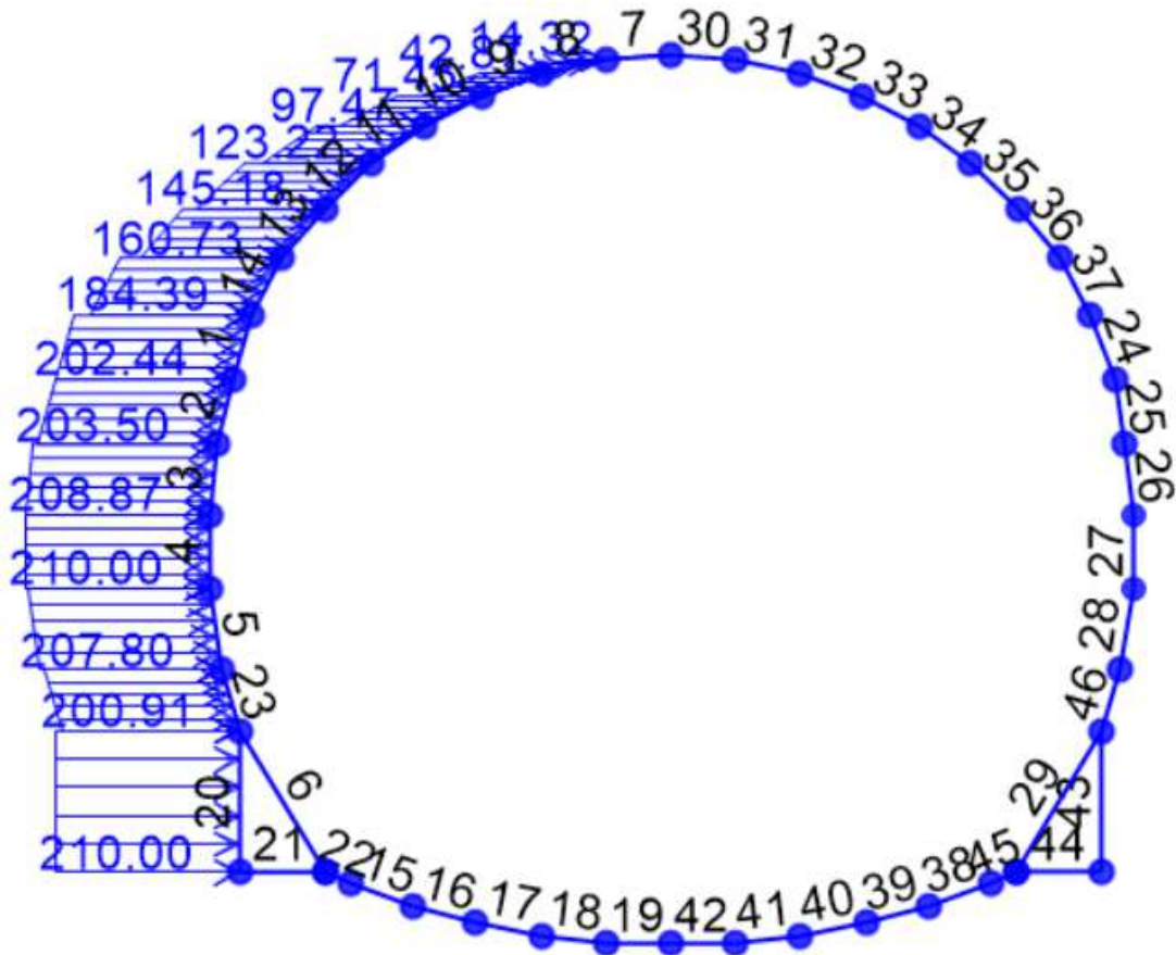
Figura 12 – Carico applicato: spinta sismica orizzontale lato sinistro
