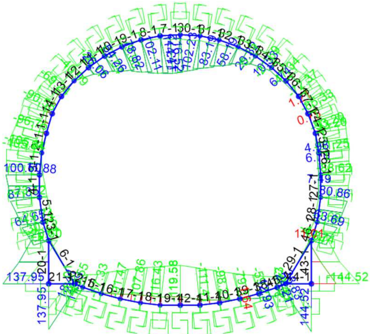
Figura 39 – Diagramma di involuppo del Momento flettente (condizioni statiche SLU)
