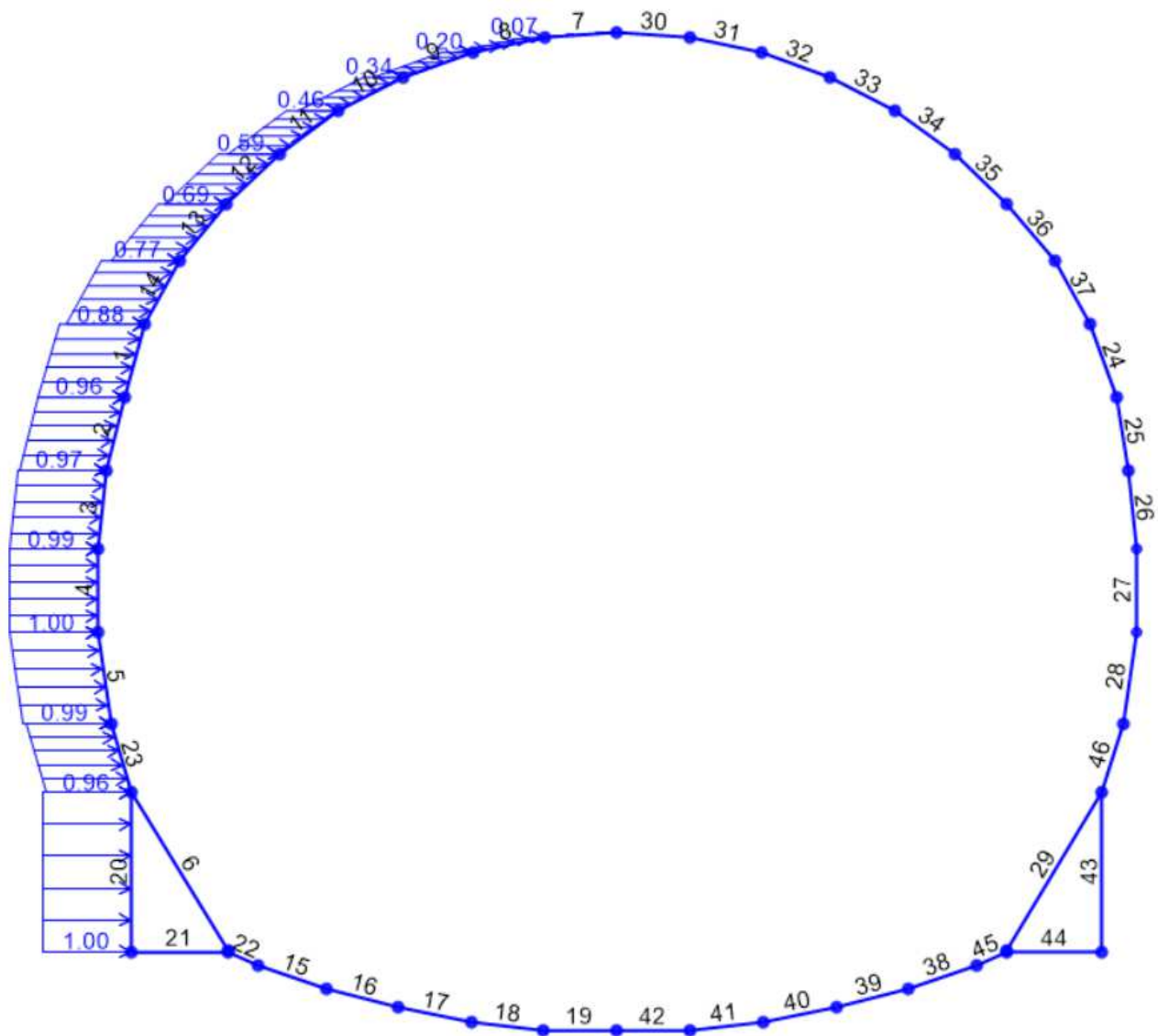
Figura 34 - Sovraccarico laterale SQ.sx sul lato sinistro, dovuto al carico variabile in copertura ( 20 \text{ kN/m} \cdot k_{0-sn} )
