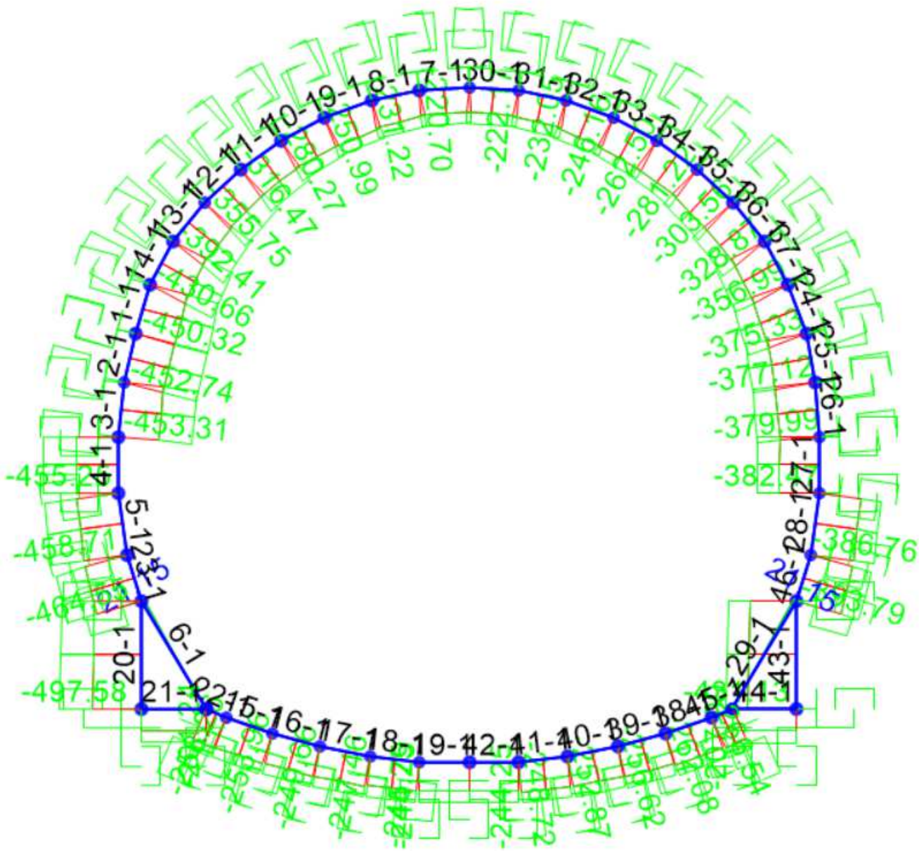
Figura 41 – Diagramma di involuppo dell'Azione assiale (condizioni statiche SLU)
