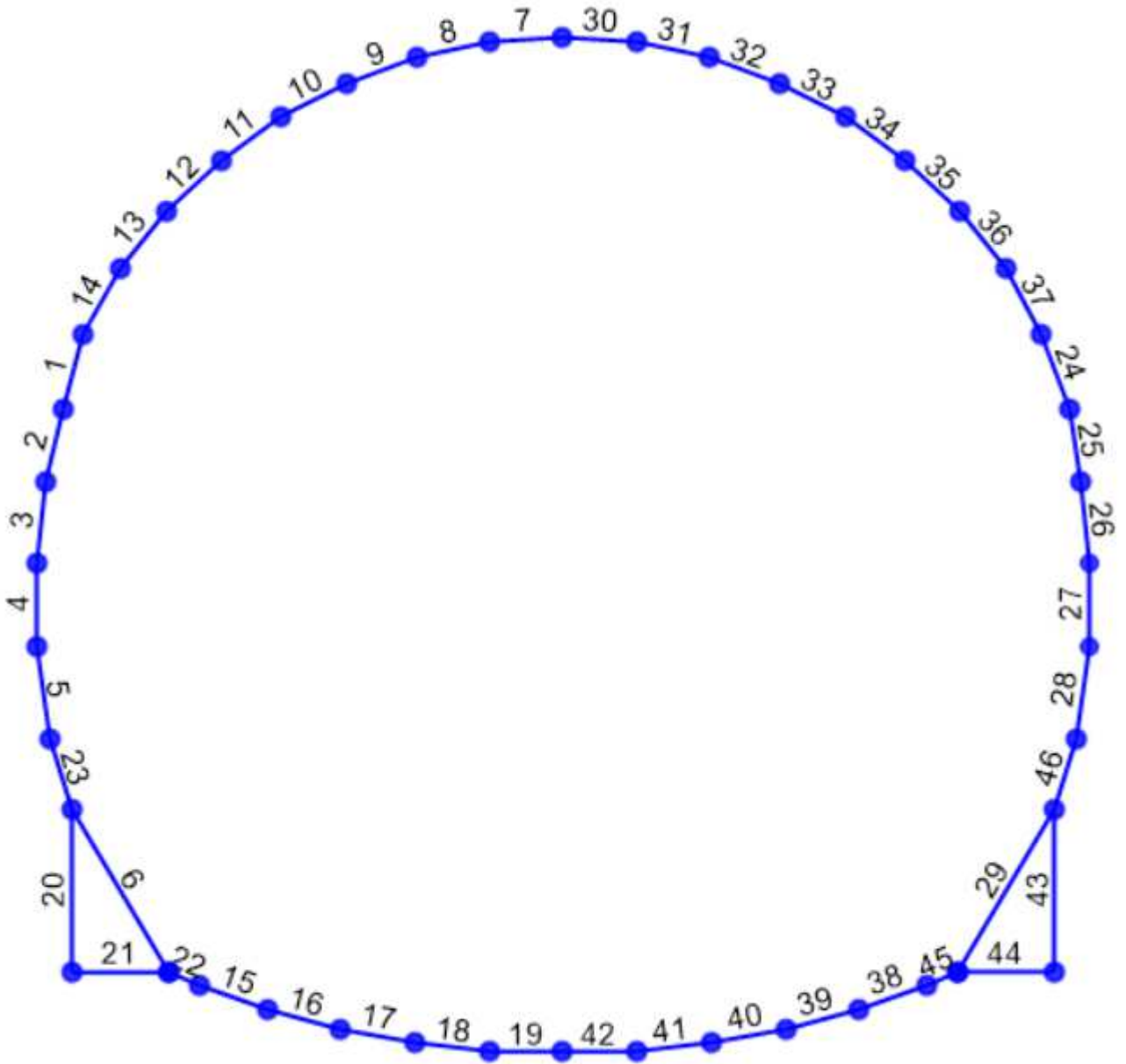
Figura 27 – Numerazione nodi e numerazione elementi beam
