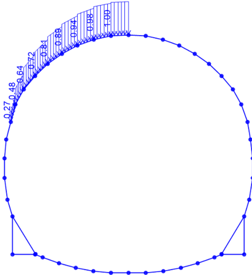
Figura 8 – Carico variabile Q_d sx applicato in copertura sul lato sinistro
