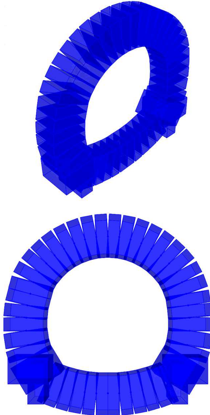
Figura 4 – Modello strutturale con evidenziati gli spessori degli elementi beam
