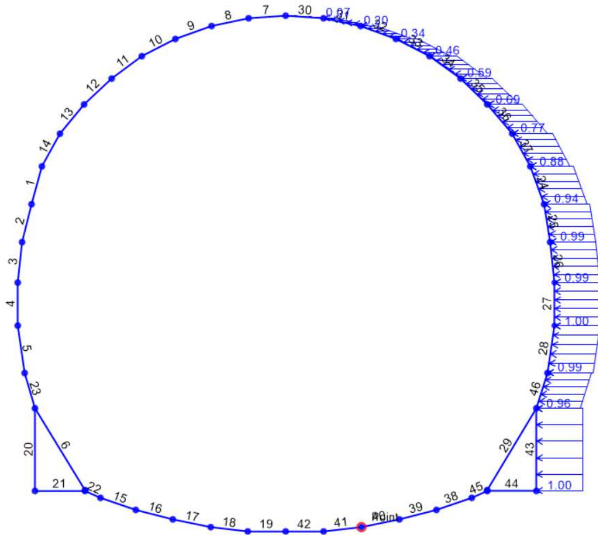
Figura 35 – Sovraccarico laterale SQ.dx sul lato destro, dovuto al carico variabile in copertura ( 20 \text{ kN/m} \cdot k_{0-dx} )
