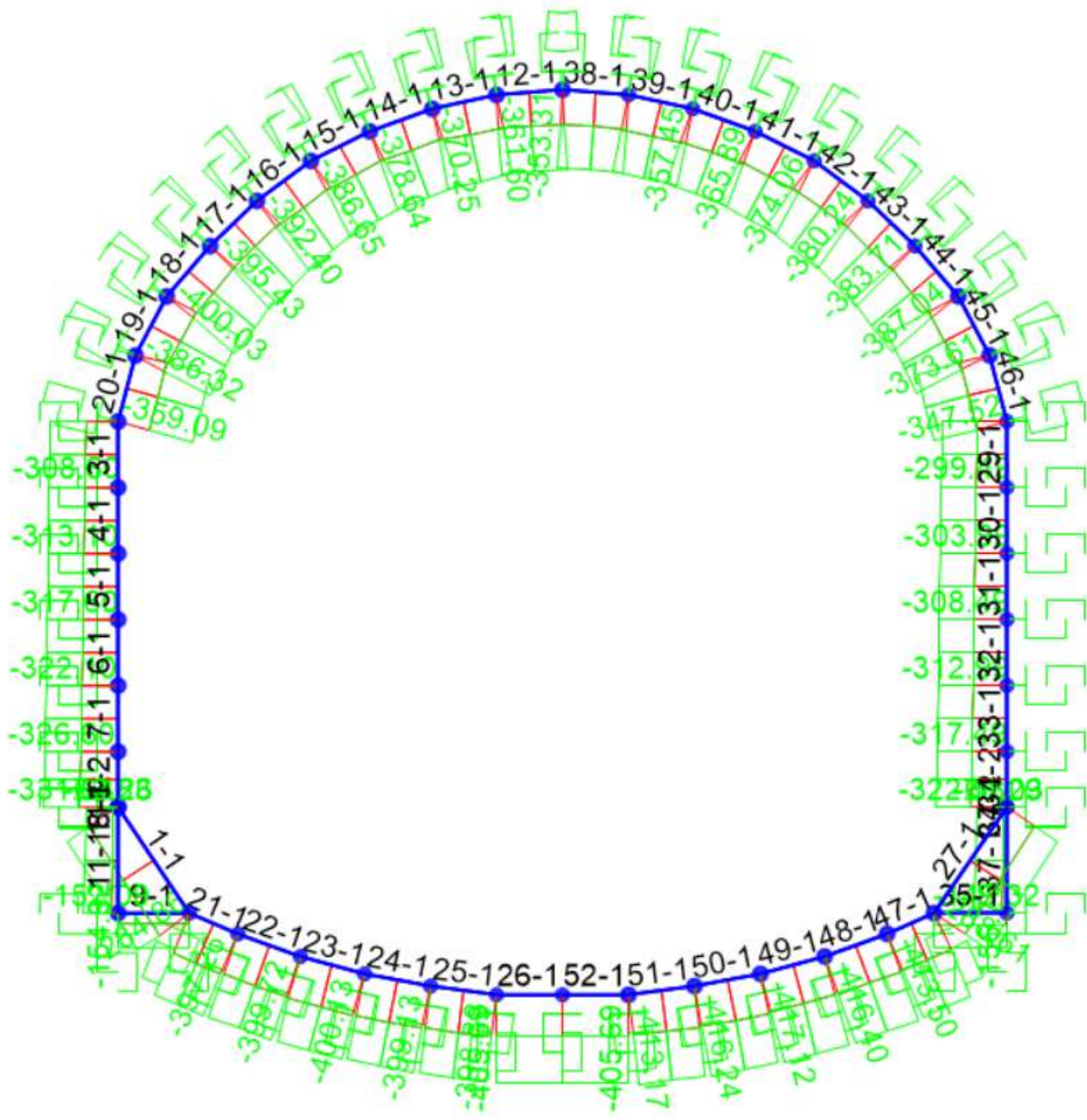
Figura 51 – Diagramma di involuppo dell'azione assiale (condizioni sismiche SLV)
