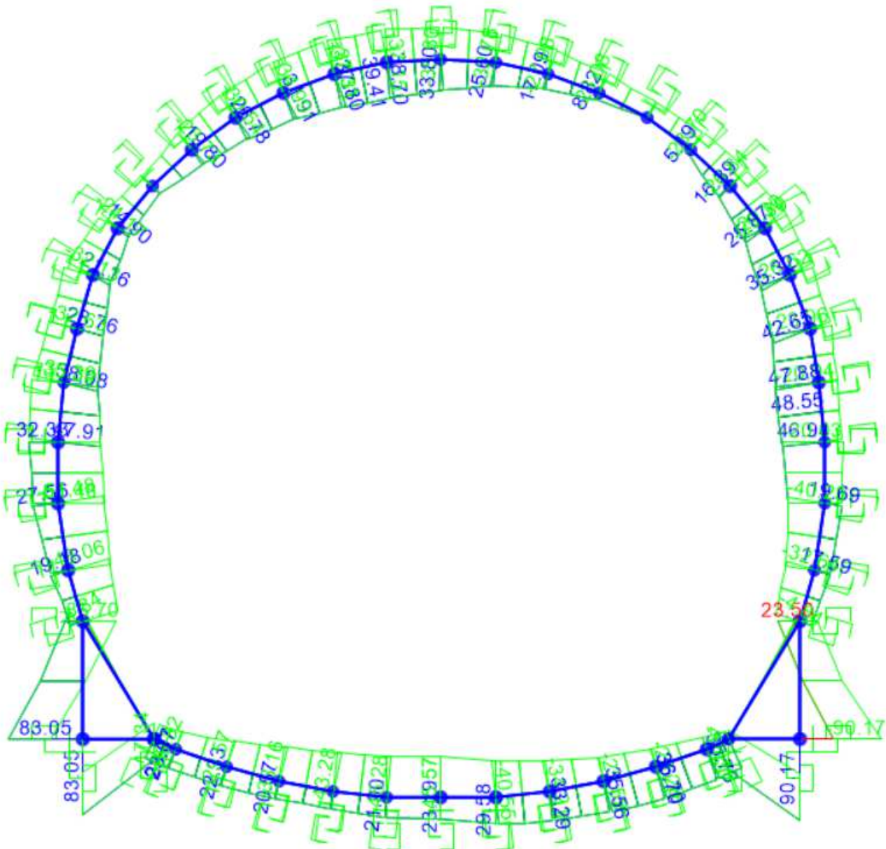
Figura 53 – Diagramma di involuppo del Momento flettente (condizioni statiche SLU)
