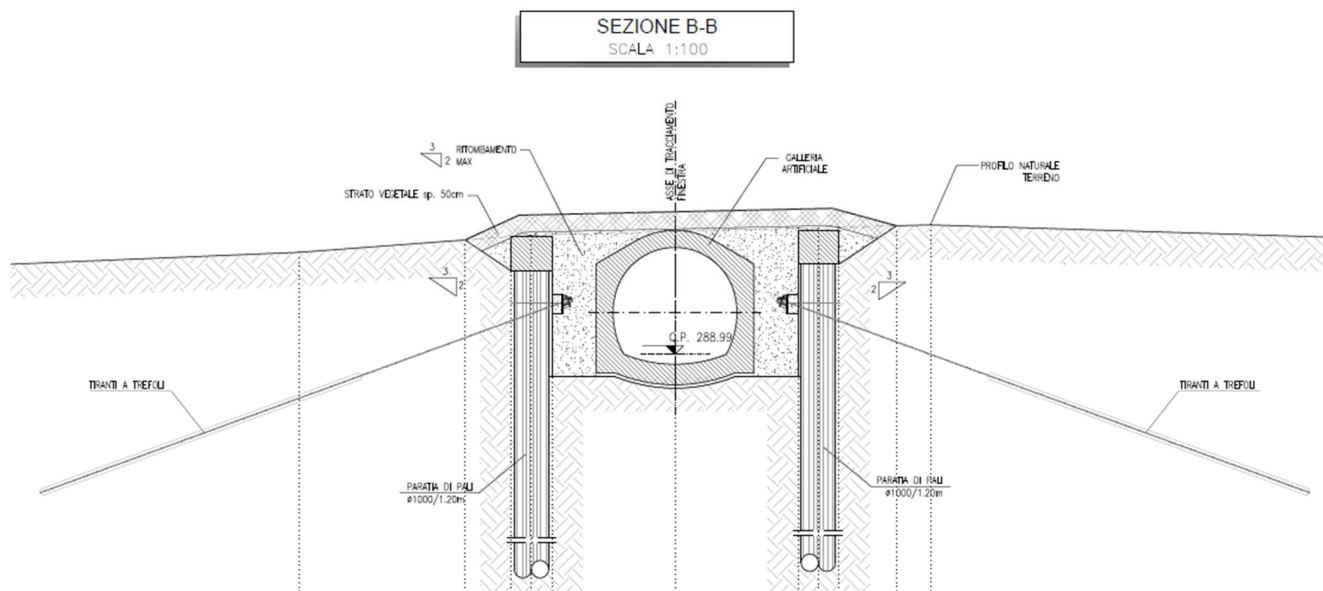
Figura 2– Sezione con le relative altezze di ritombamento
