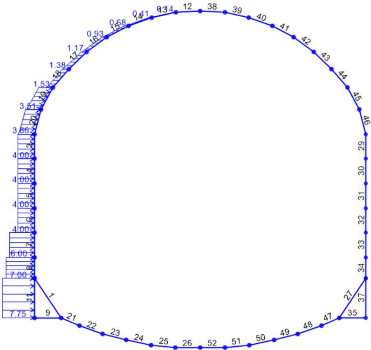
Figura 18 – Carico dovuto alla spinta orizzontale sinistra SP.sx (K_{osn} \cdot \gamma_{rit} \cdot H_{rit})
