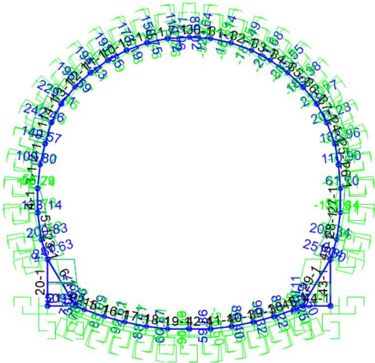
Figura 43 – Diagramma di involuppo del Taglio (condizioni sismiche SLV)
