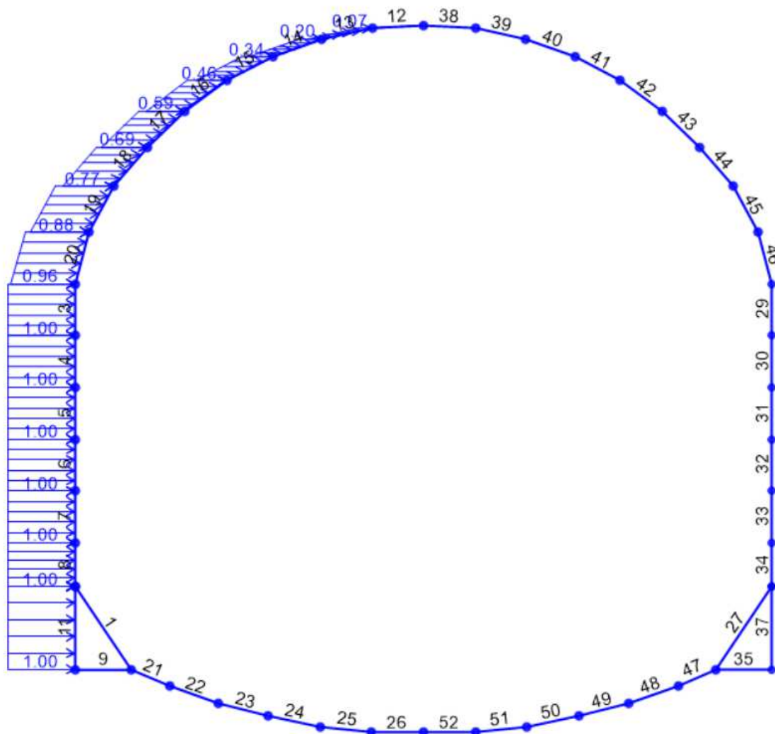
Figura 22 – Sovraccarico laterale SQ.sx sul lato sinistro, dovuto al carico variabile in copertura ( 20 \text{ kN/m} \cdot k_{0\text{-sn}} )
