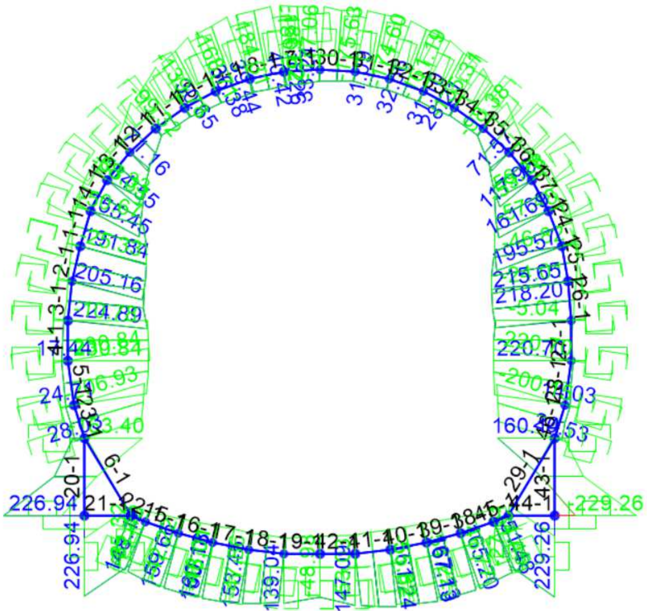
Figura 42 – Diagramma di involuppo del Momento flettente (condizioni sismiche SLV)
