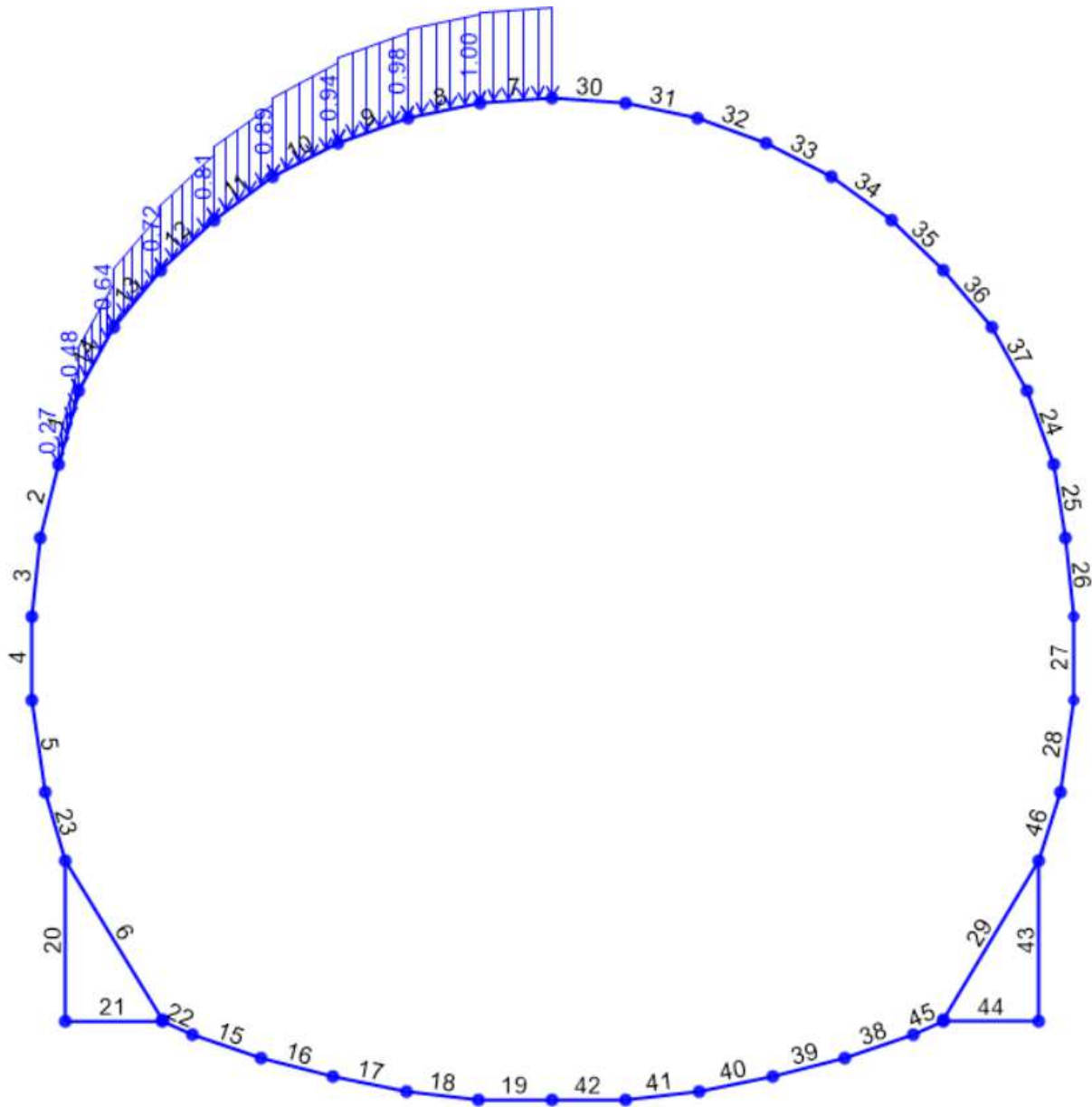
Figura 32 – Carico variabile Q_{d\_sx} applicato in copertura sul lato sinistro
