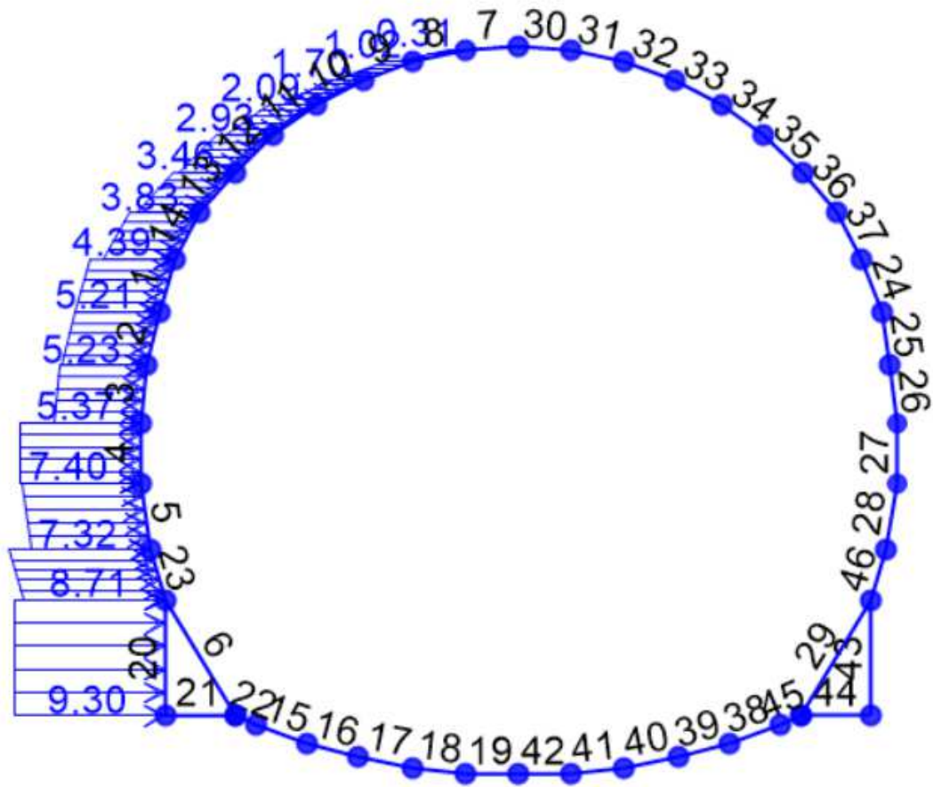
Figura 6 – Carico dovuto alla spinta orizzontale sinistra SP.sx ( K_{osn} \cdot \gamma_{rit} \cdot H_{rit} )
