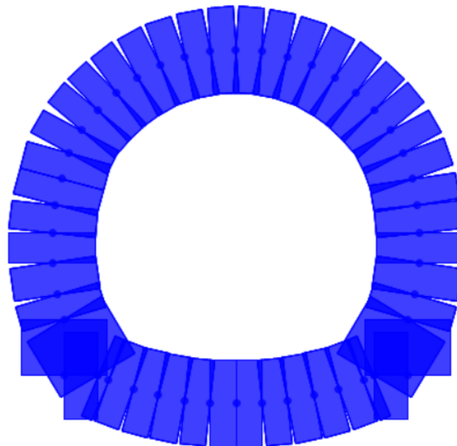
Figura 28 – Modello strutturale con evidenziati gli spessori degli elementi beam
