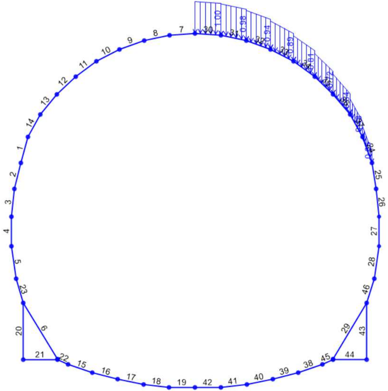
Figura 33 – Carico variabile Q_{d,dx} applicato in copertura sul lato destro
