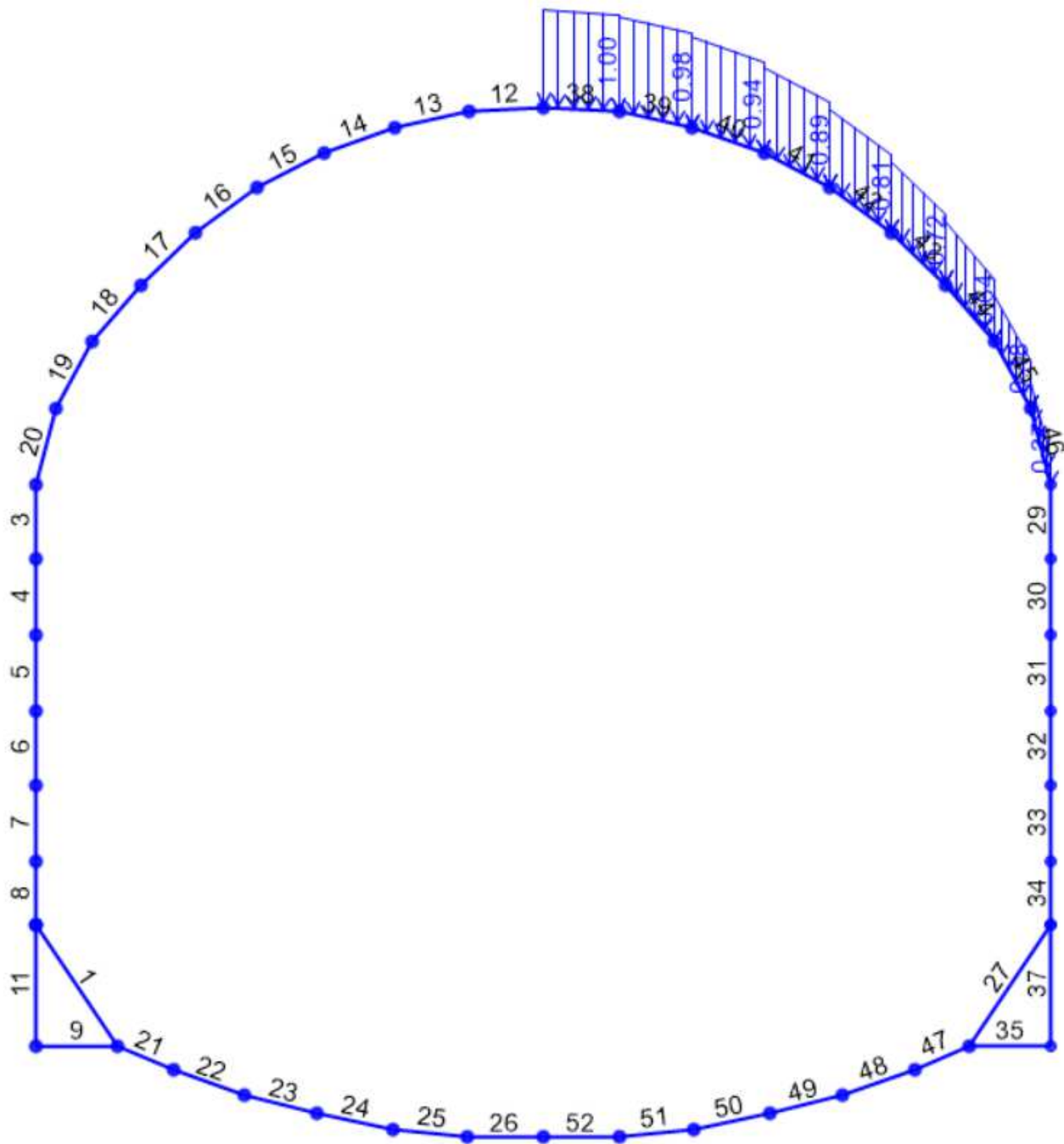
Figura 21 – Carico variabile Q_{d\_dx} applicato in copertura sul lato destro
