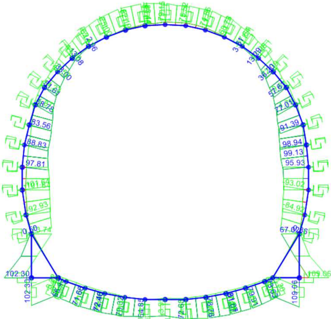
Figura 56 – Diagramma di involuppo del Momento flettente (condizioni sismiche SLV)
