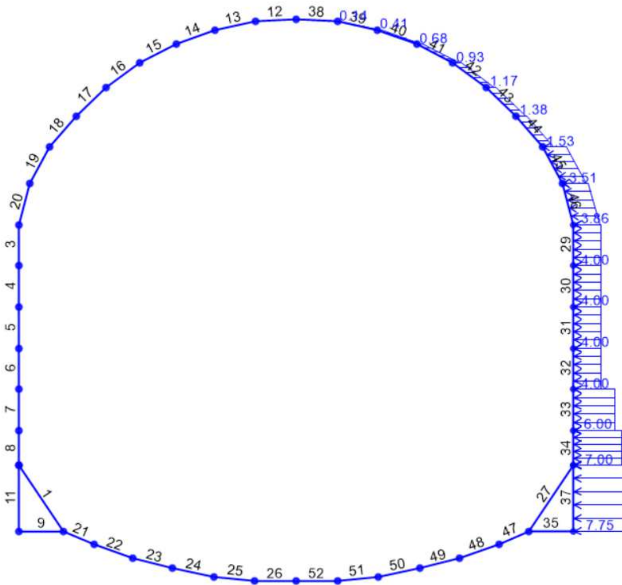
Figura 19 – Carico dovuto alla spinta orizzontale destra SP.dx ( K_{odx} * \gamma_{rit} * H_{rit} )
