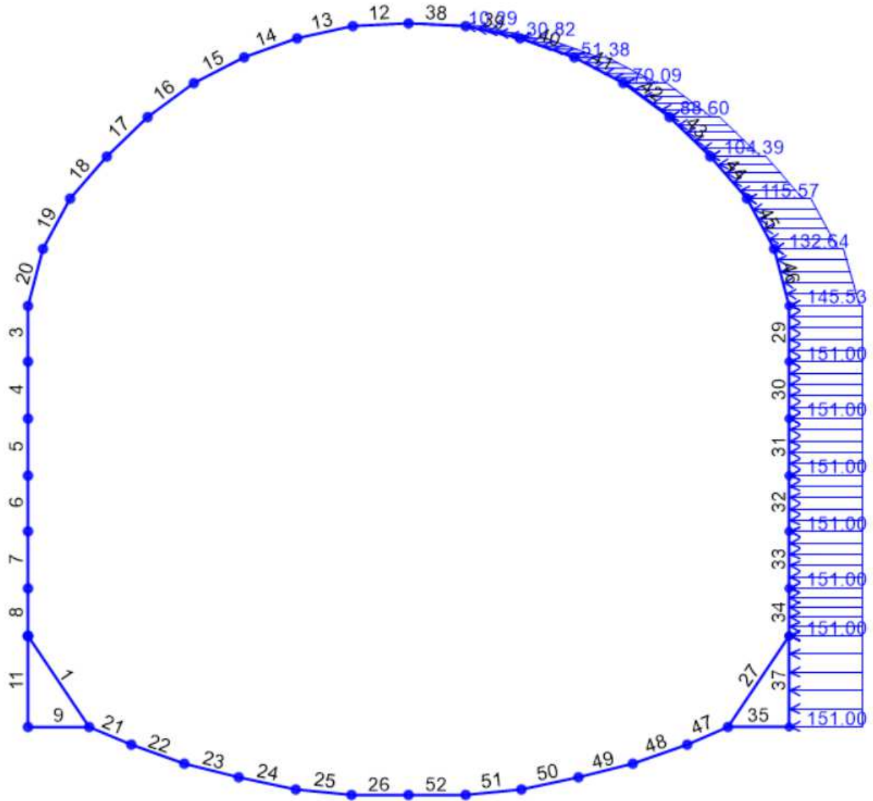
Figura 25 – Carico applicato: spinta sismica orizzontale lato destro
