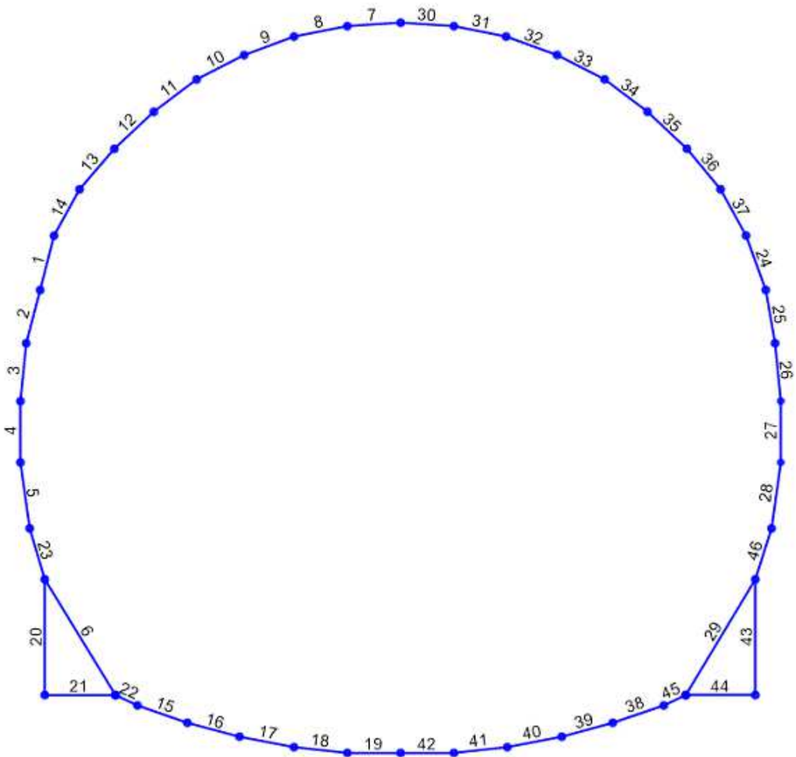
Figura 3 – Numerazione elementi beam
