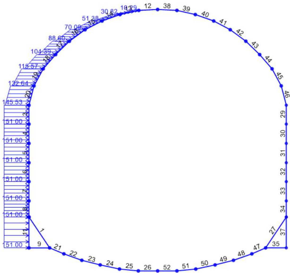
Figura 24 – Carico applicato: spinta sismica orizzontale lato sinistro
