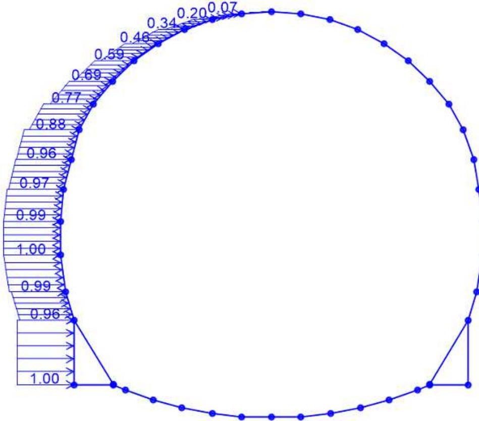
Figura 10 – Sovraccarico laterale SQ.sx sul lato sinistro, dovuto al carico variabile in copertura (20 kN/m * k 0-sn )
