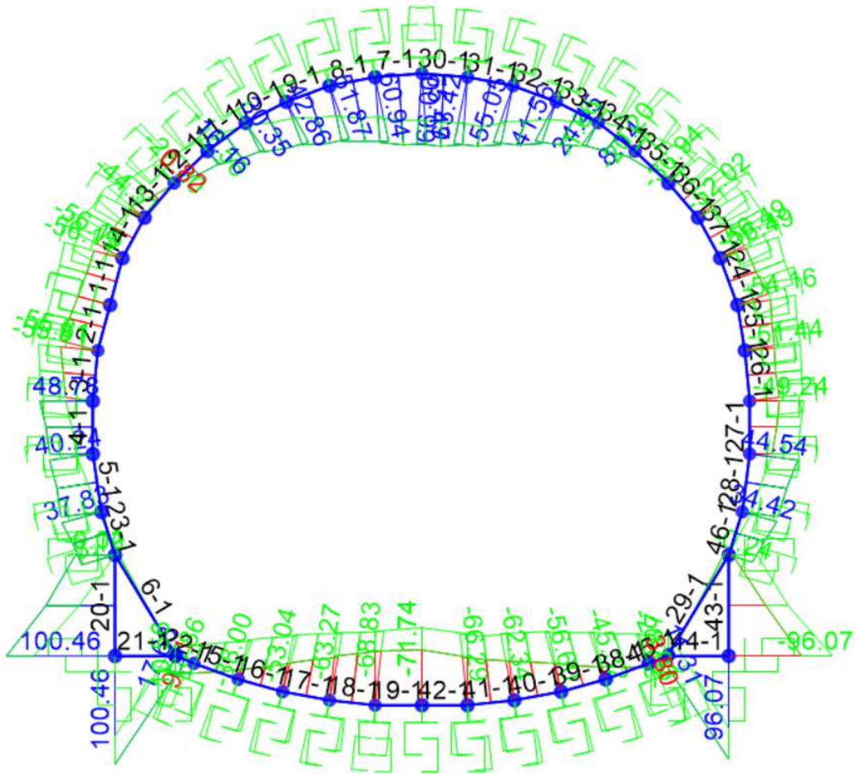
Figura 60 – Diagramma di involuppo del Momento flettente (INVILUPPO SLE-F)
