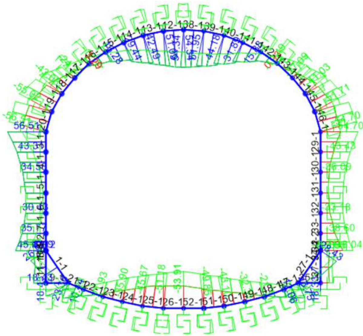
Figura 62 – Diagramma di involuppo del Momento flettente (INVILUPPO SLE-F)
