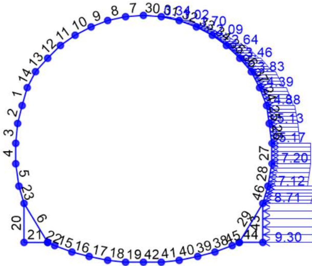
Figura 7 – Carico dovuto alla spinta orizzontale destra SP.dx ( K_{odx} * \gamma_{rit} * H_{rit} )
