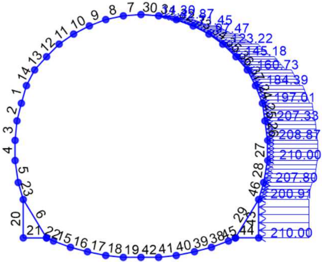
Figura 13 – Carico applicato: spinta sismica orizzontale lato destro
