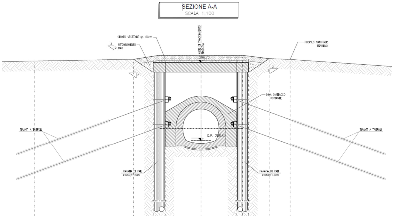
Figura 1 – Sezione con le relative altezze di ritombamento
