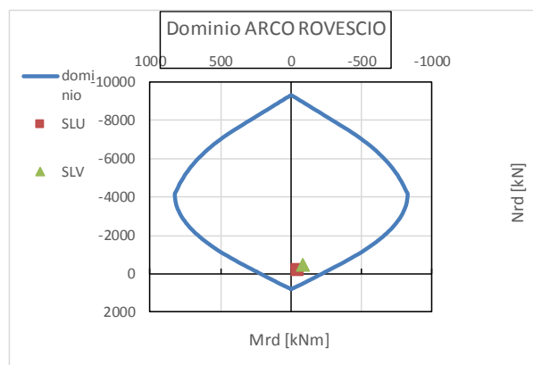
Figura 59 – Domini M-N – SLU
