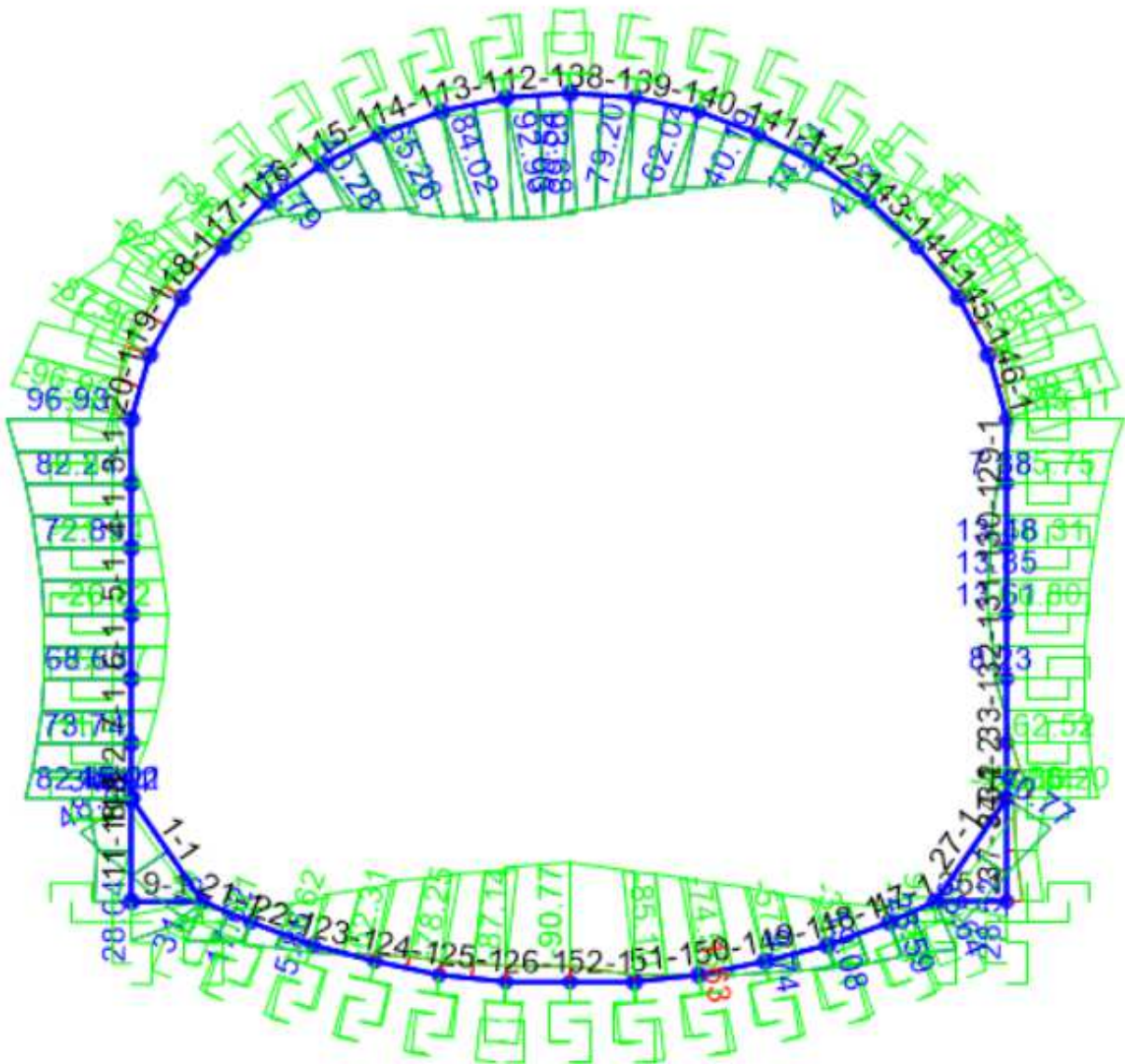
Figura 46 – Diagramma di involuppo del Momento flettente (condizioni statiche SLU)
