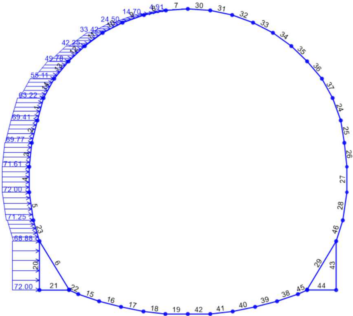
Figura 36 – Carico applicato: spinta sismica orizzontale lato sinistro
