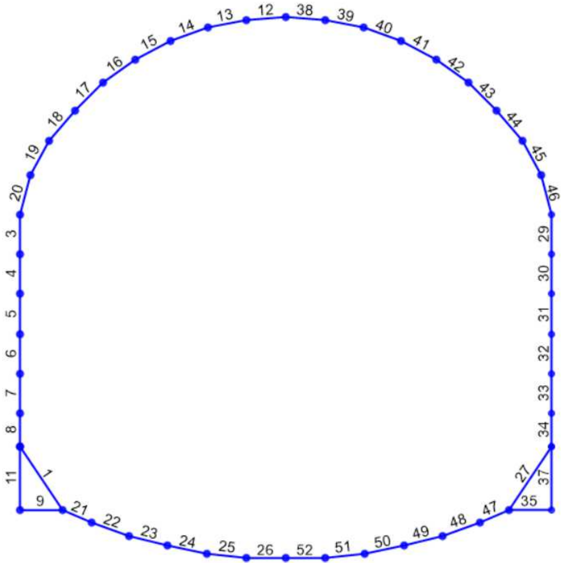
Figura 15 – Numerazione elementi beam
