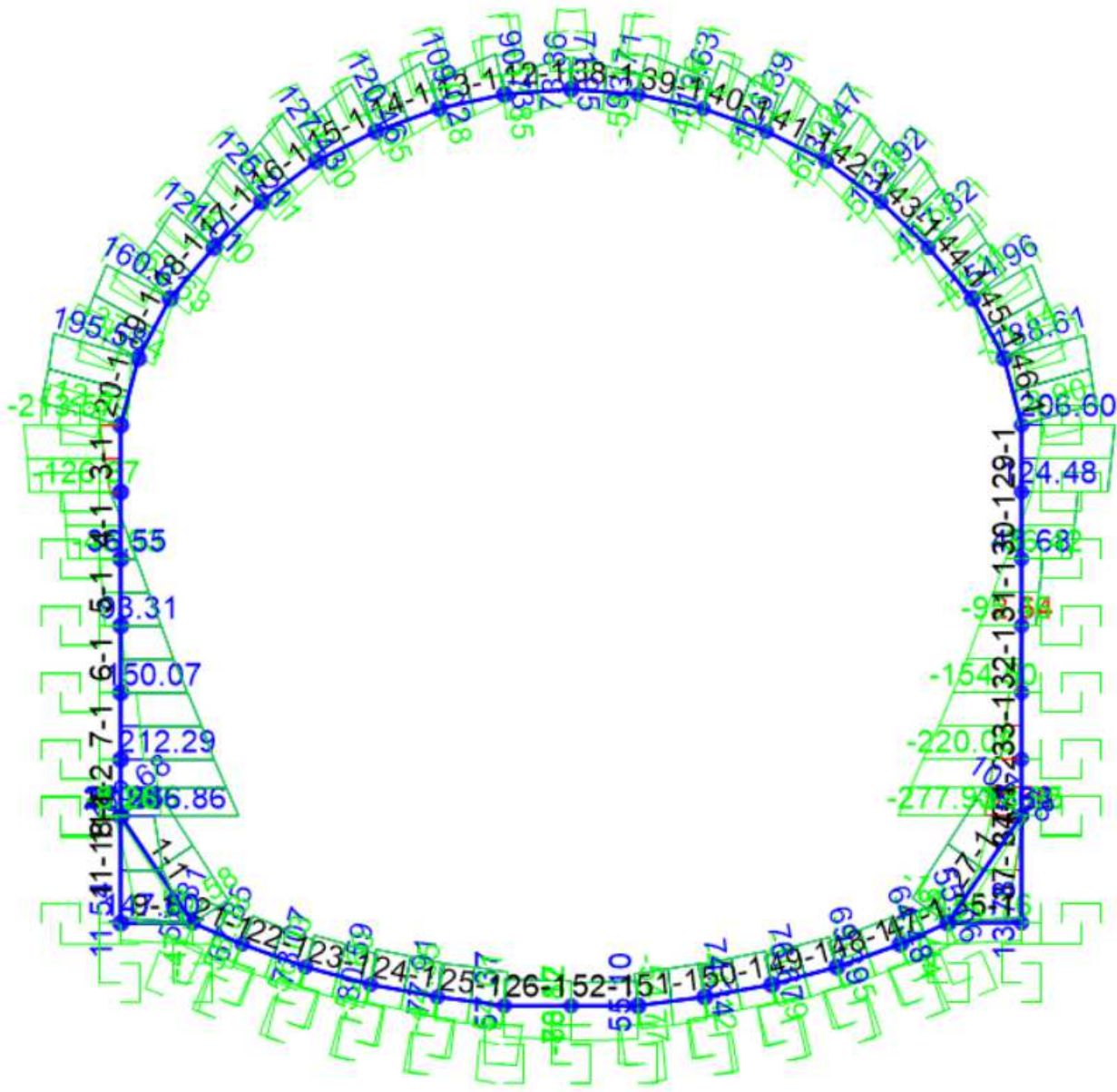
Figura 50 – Diagramma di involuppo del Taglio (condizioni sismiche SLV)
