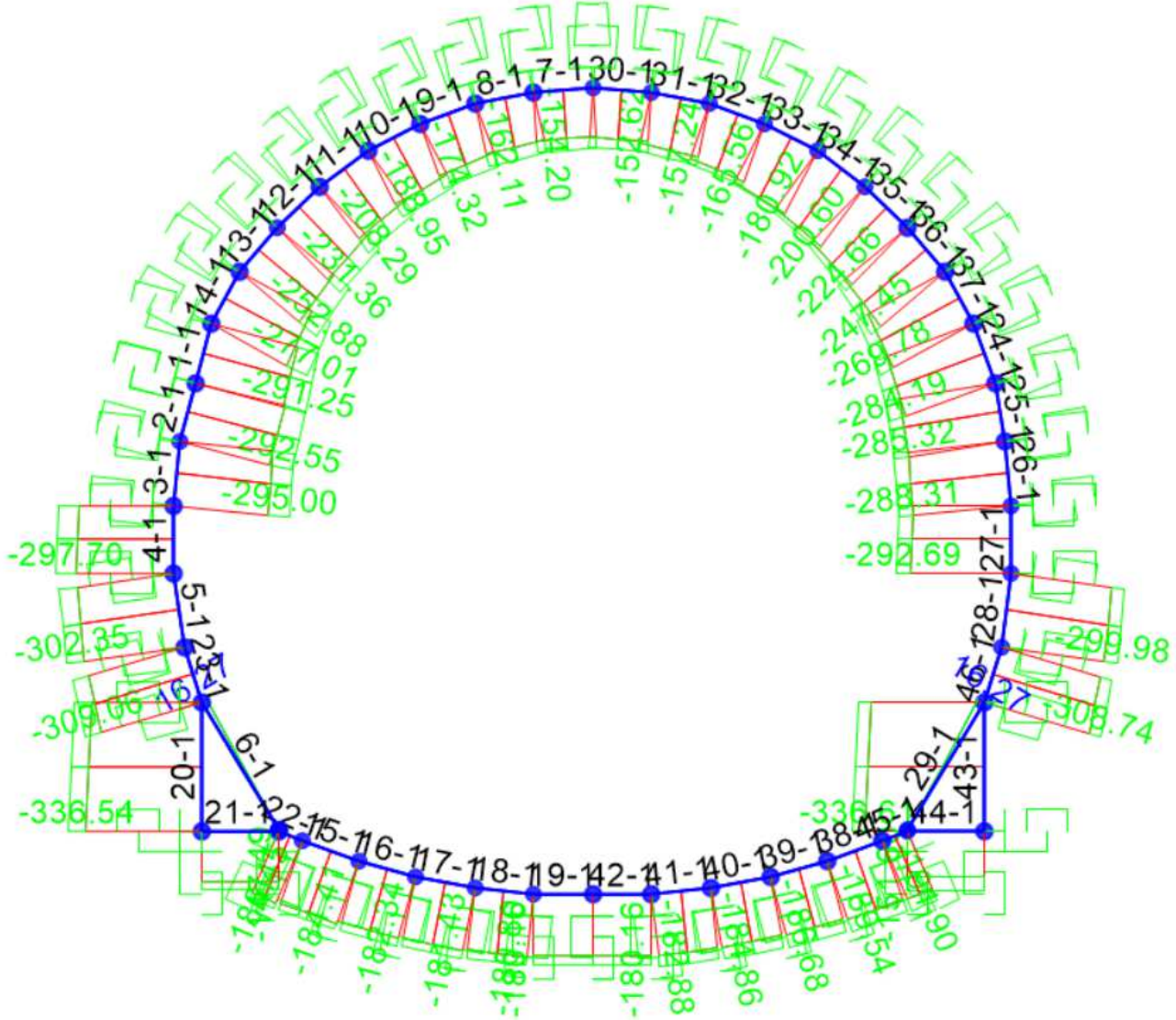
Figura 61 – Diagramma di involuppo dell’Azione assiale (INVILUPPO SLE-F)
