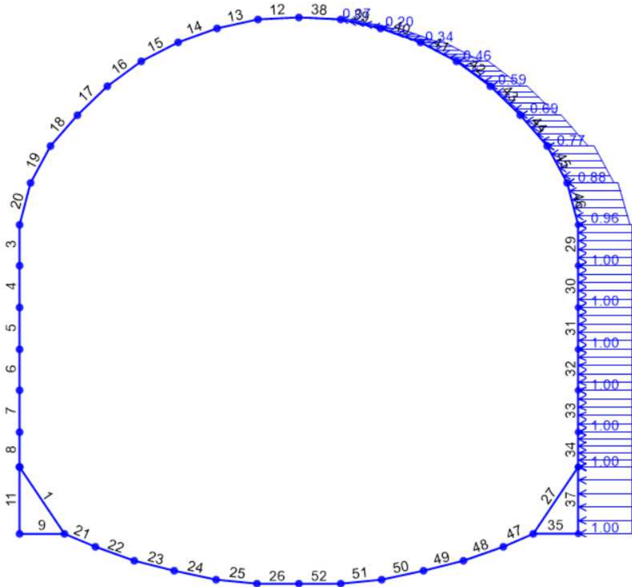
Figura 23 – Sovraccarico laterale SQ.dx sul lato destro, dovuto al carico variabile in copertura (20 kN/m * k 0-dx )
