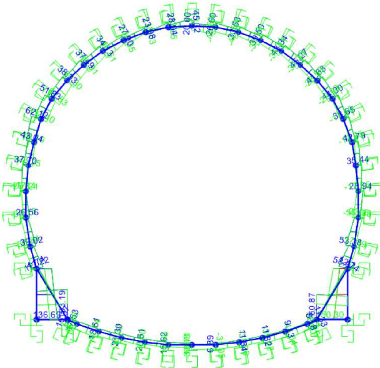
Figura 54 – Diagramma di involuppo del Taglio (condizioni statiche SLU)
