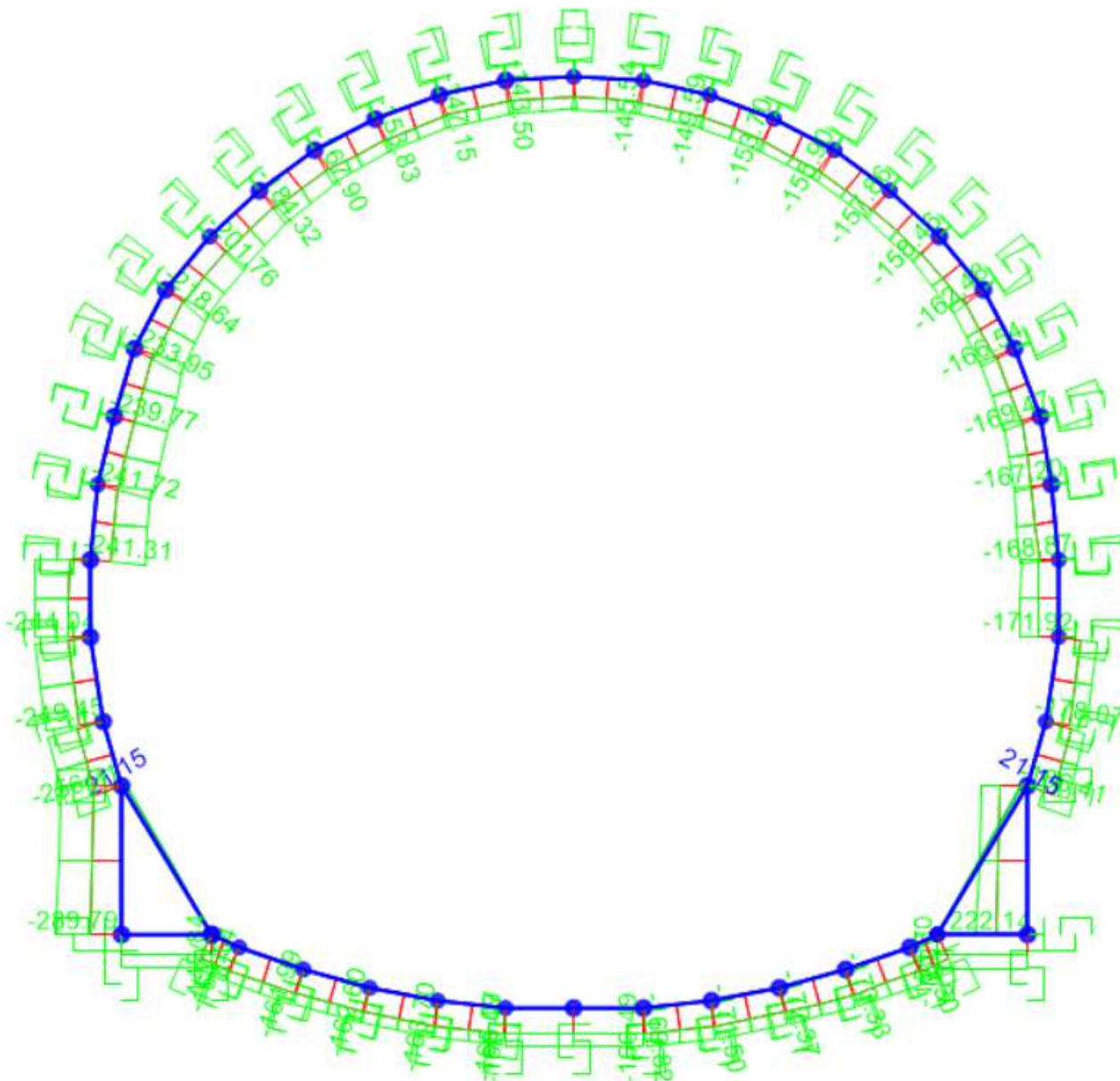
Figura 55 – Diagramma di involuppo dell'Azion assiale (condizioni statiche SLU)
