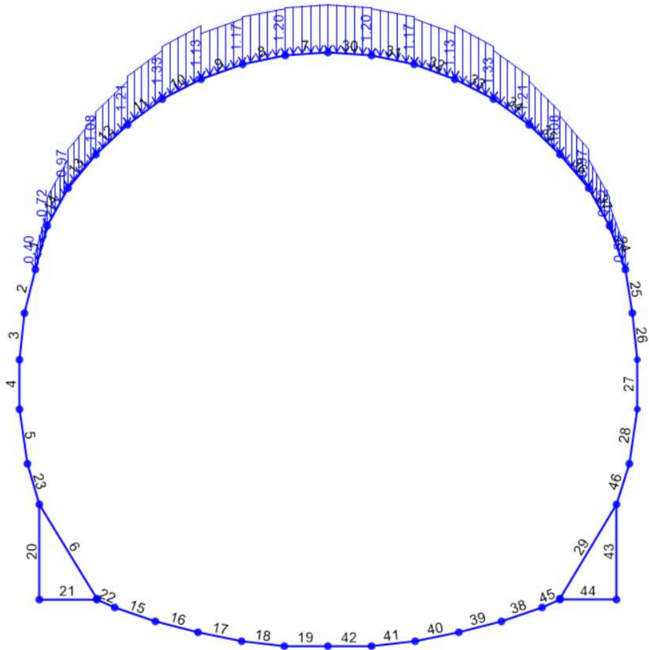
Figura 29 – Carico di ricoprimento P_{cop} (\gamma_{rit} * H_{rit})
