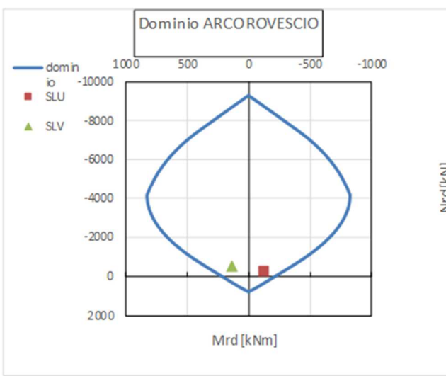
Figura 45 – Domini M-N – SLU
