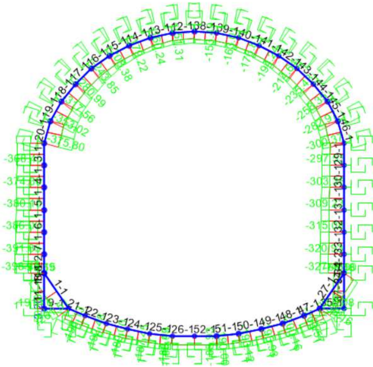
Figura 48 – Diagramma di involuppo dell'Azione assiale (condizioni statiche SLU)
