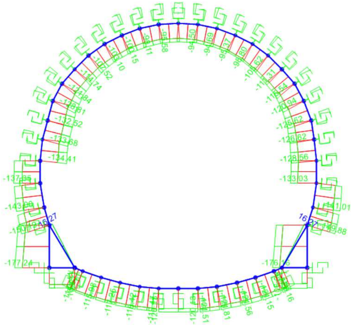
Figura 65 – Diagramma di involuppo dell'azione assiale (INVILUPPO SLE-F)
