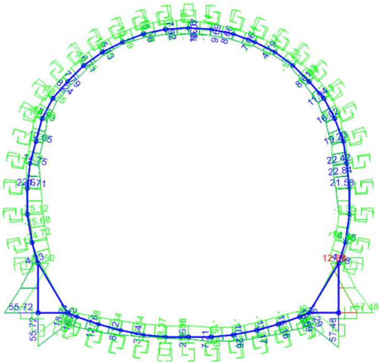
Figura 64 – Diagramma di involuppo del Momento flettente (INVILUPPO SLE-F)
