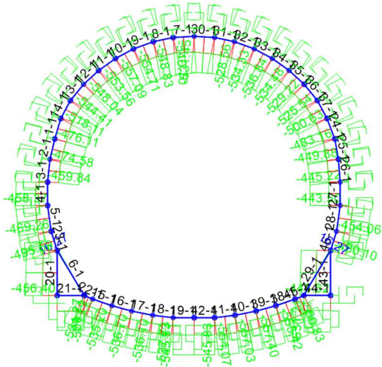
Figura 44 – Diagramma di involuppo dell'azione assiale (condizioni sismiche SLV)
