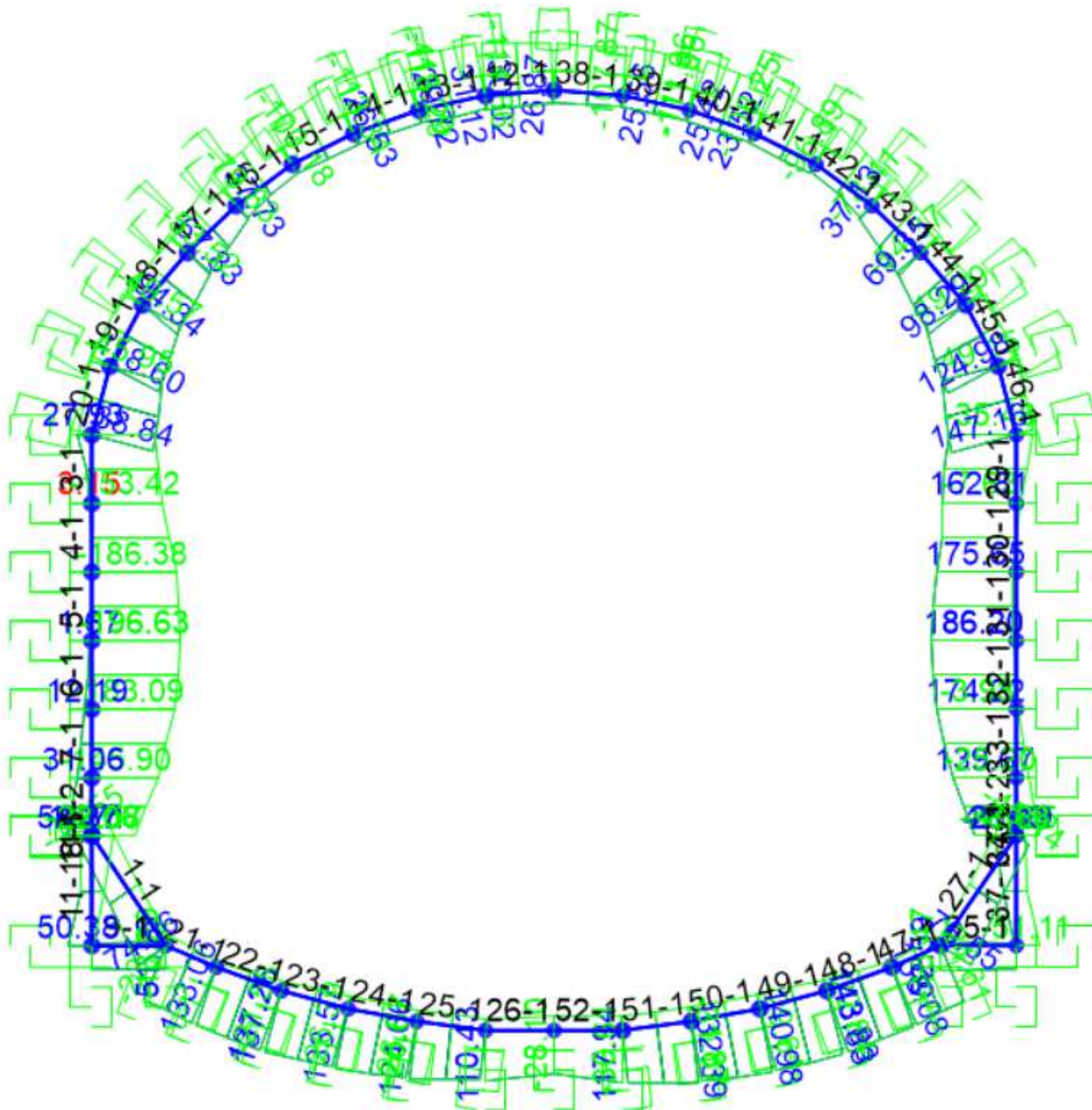
Figura 49 – Diagramma di involuppo del Momento flettente (condizioni sismiche SLV)
