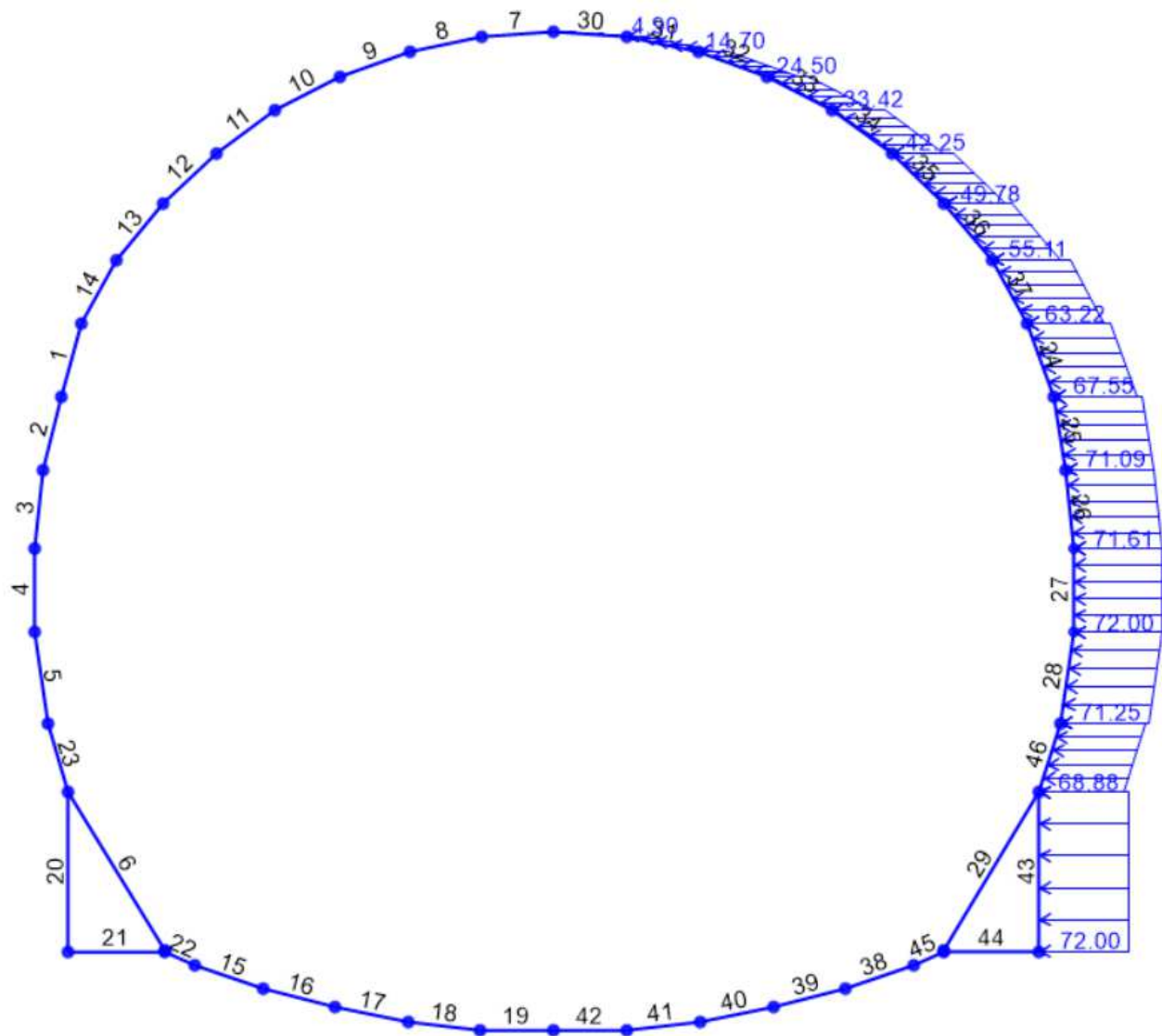
Figura 37 – Carico applicato: spinta sismica orizzontale lato destro
