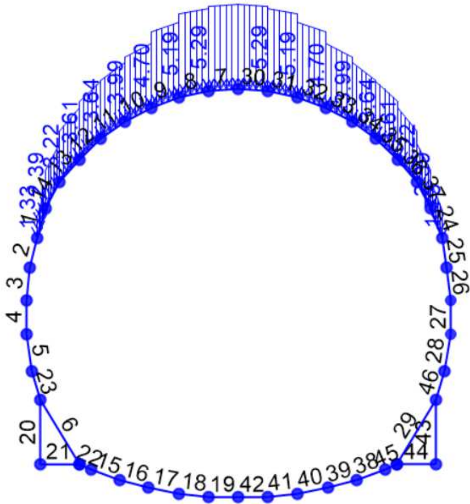
Figura 5 – Carico di ricoprimento P_{cop} ( \gamma_{rit} \cdot H_{rit} )
