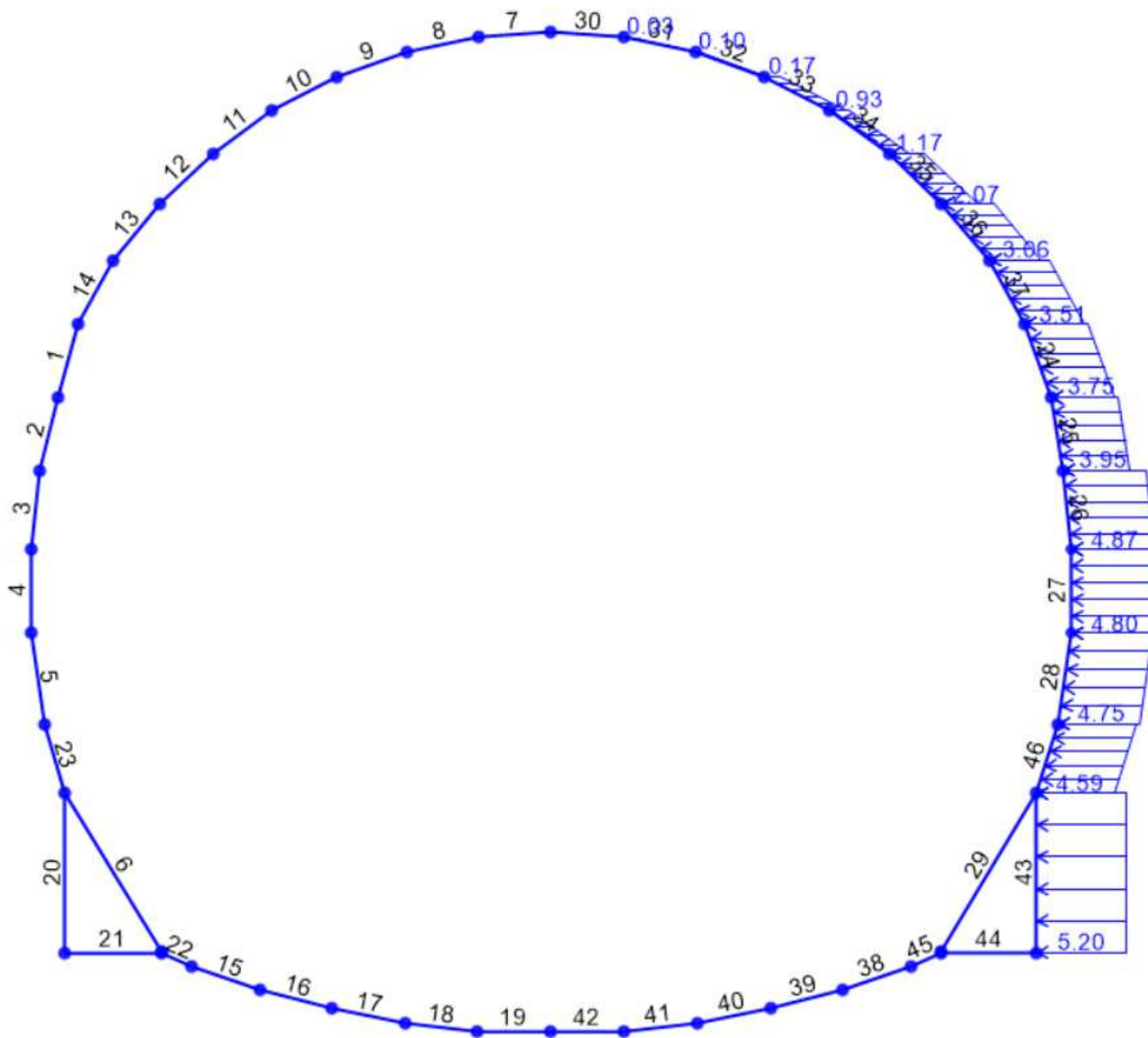
Figura 31 – Carico dovuto alla spinta orizzontale destra SP.dx (K_{odx} * \gamma_{rit} * H_{rit})
