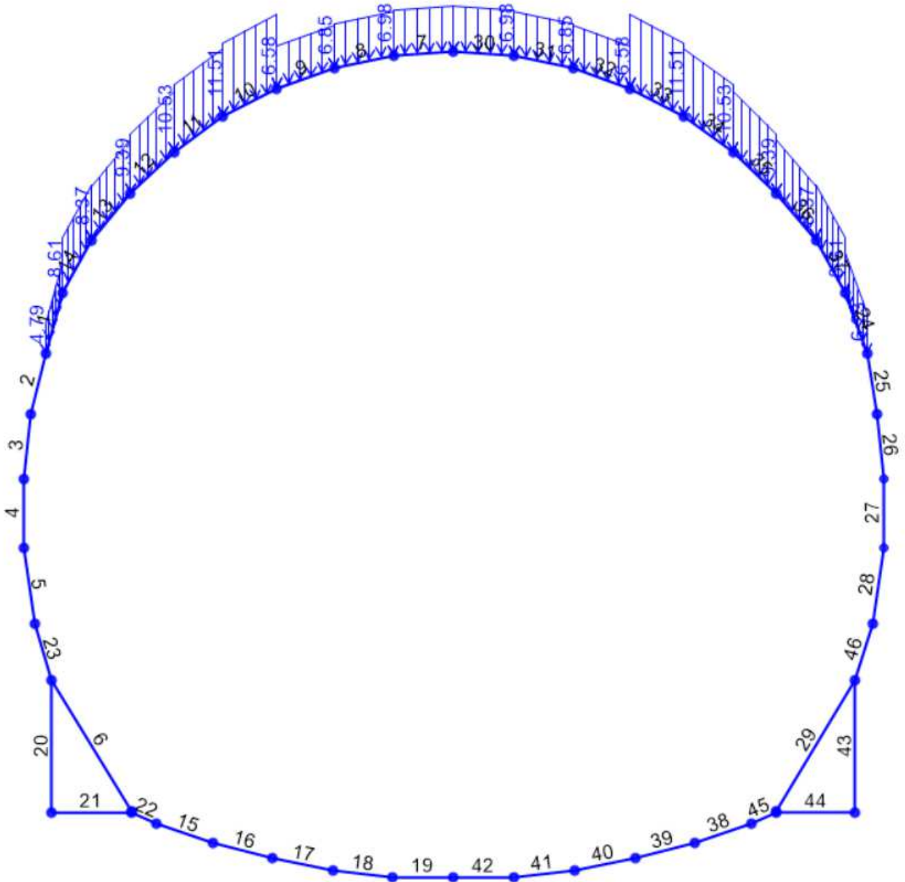
Figura 38– Carico applicato spinta sismica verticale
