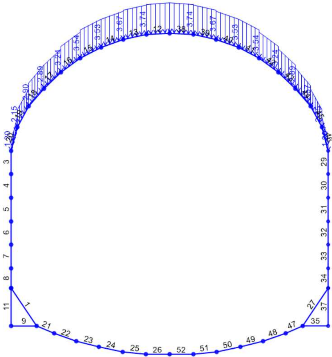
Figura 17 – Carico di ricoprimento P_{cop} (\gamma_{rit} * H_{rit})
