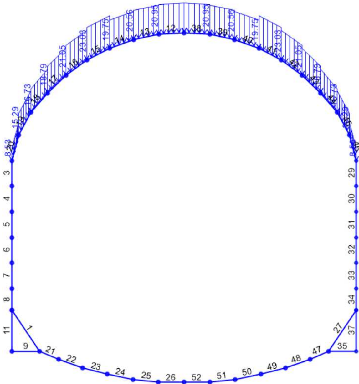
Figura 26 – Carico applicato spinta sismica verticale
