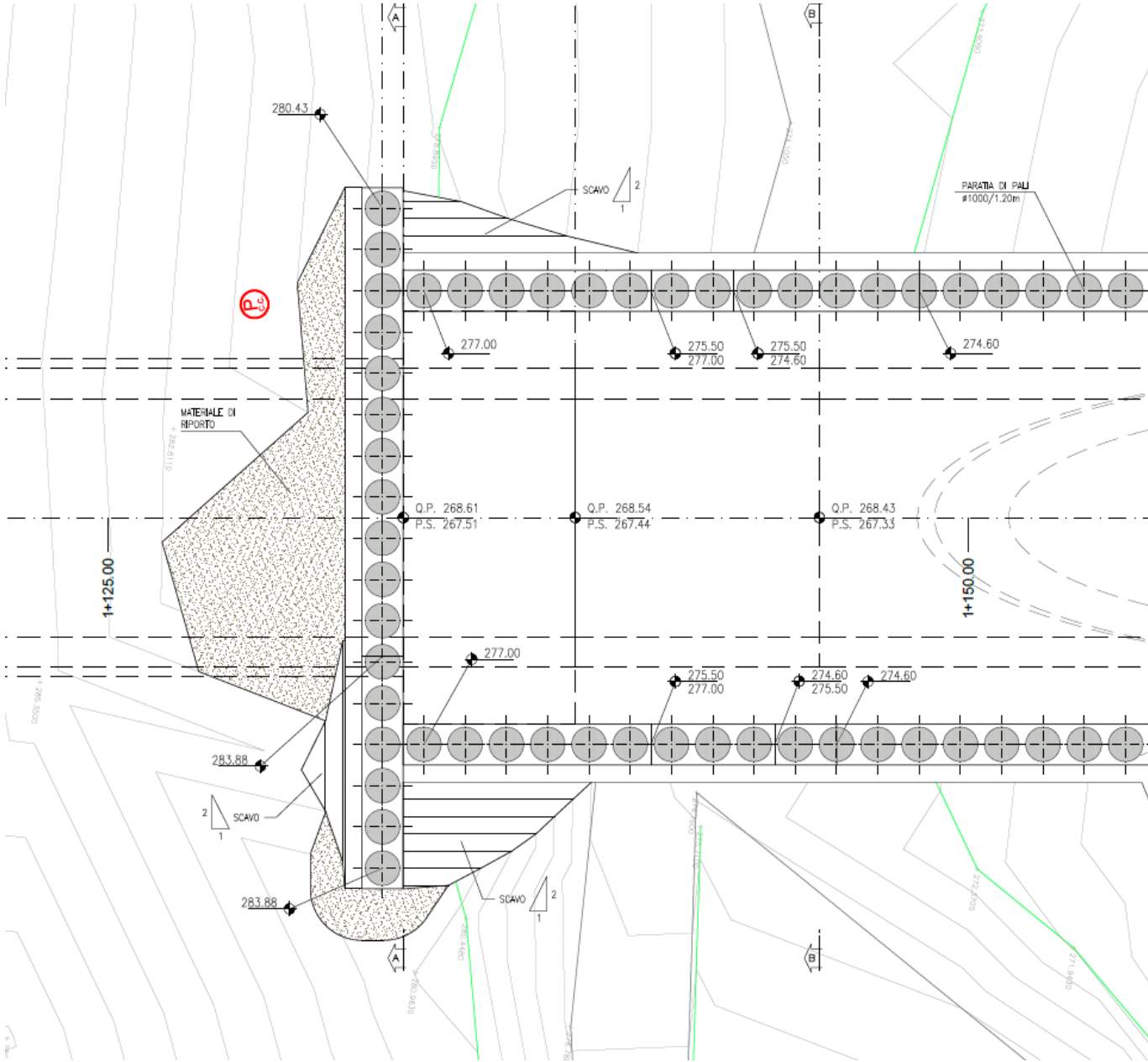
Figura 3-1 – Posizionamento piezometro (in rosso)
