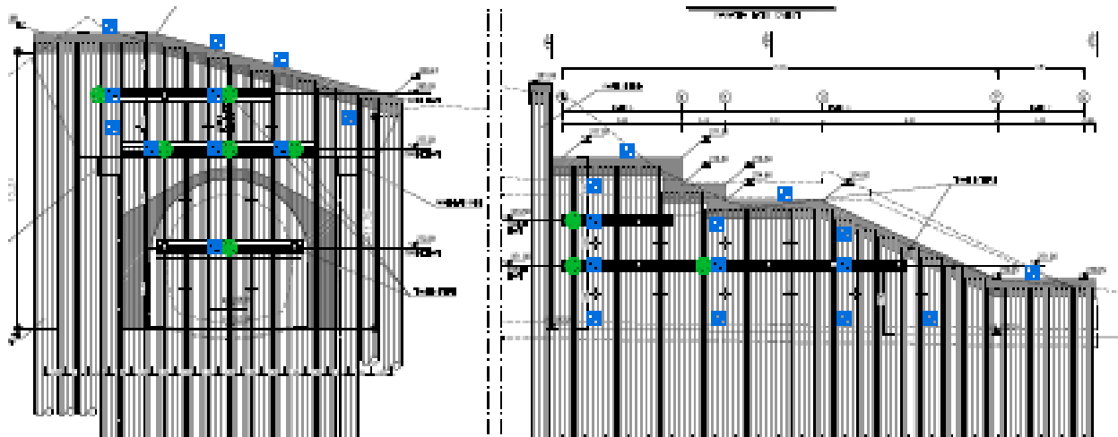
Figura 3-2. Monitoraggio paratia: posizionamento delle mire ottiche (blu) e delle celle di carico toroidali (verdi)
