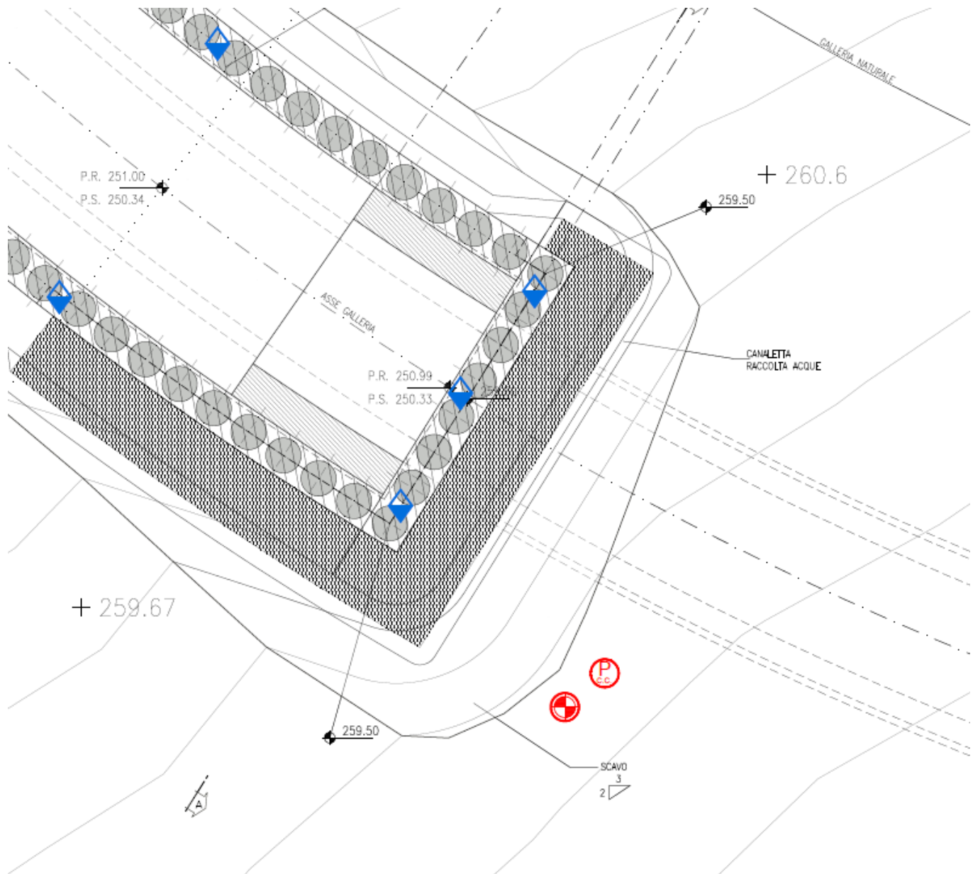
Figura 3-1 – Posizionamento di inclinometri e piezometri (in rosso) e capisaldi/mire topografiche
