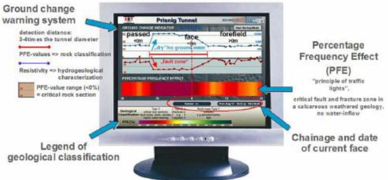
Figura 5 – Esempio di risultati riportati dal metodo BEAM relativamente ad una zona interessata dalla presenza di una faglia senza acqua.
