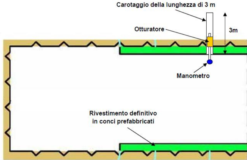
Figura 3 – Schema illustrativo dei carotaggi eseguiti attraverso il rivestimento definitivo
