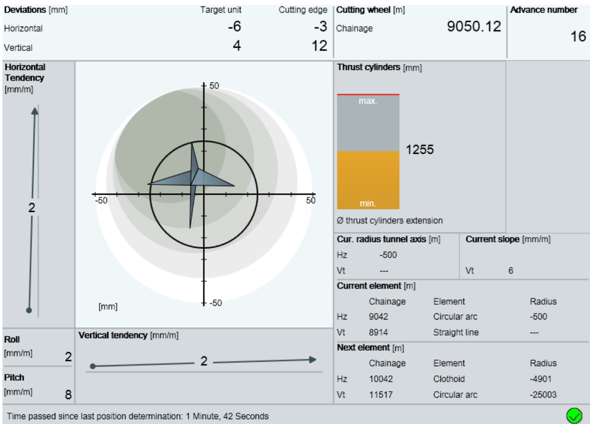
Figura 1 – Esempio di monitoraggio del sistema di guida
