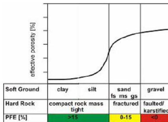
Figura 4 – Relazione fra la polarizzazione indotta (PFE) e la porosità efficace per una classificazione geologica.
