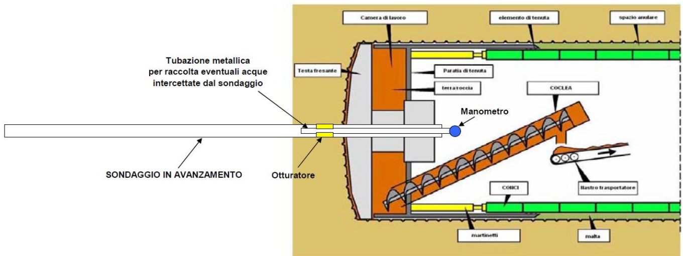
Figura 2 – Schema sondaggio in avanzamento e del sistema per la misura sia dell'eventuale acqua drenata e della pressione ("preventer").
