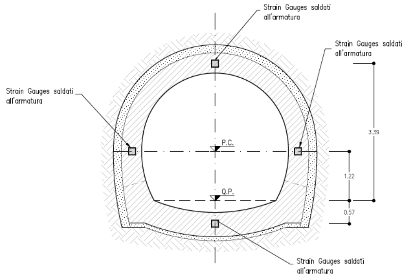
Figure 4-3. Esempio di monitoraggio rivestimento definitivo – misura dello stato tenso-deformativo
