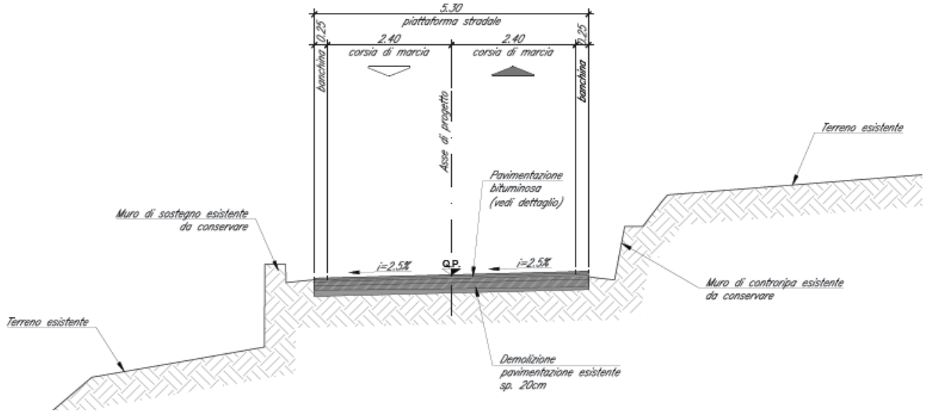
Figura 5.1.3 – Planimetria NV12-Asse A2
