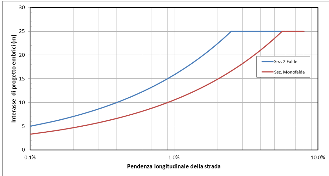
Figura 5.1: interasse massimo di scarico con embrice in rilevato.
