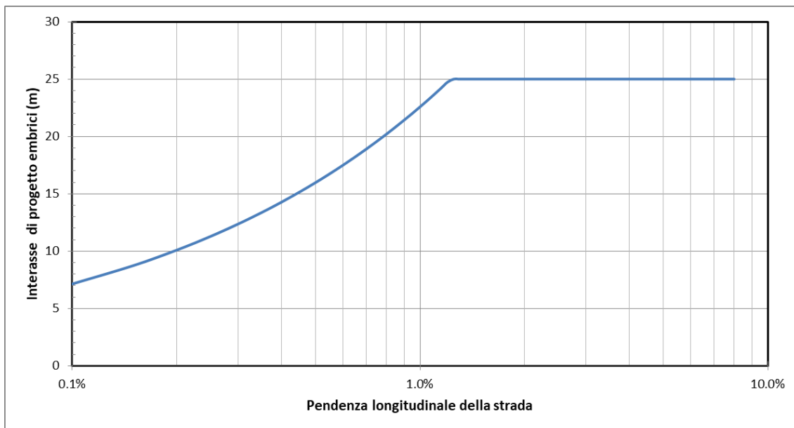
Figura 3: interasse massimo di scarico con embrice in rilevato.
