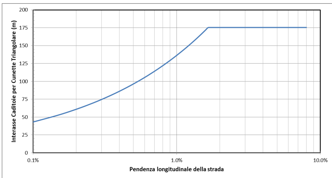
Figura 4: Interasse massimo per le caditoie di scrico delle cunette trinagolari
