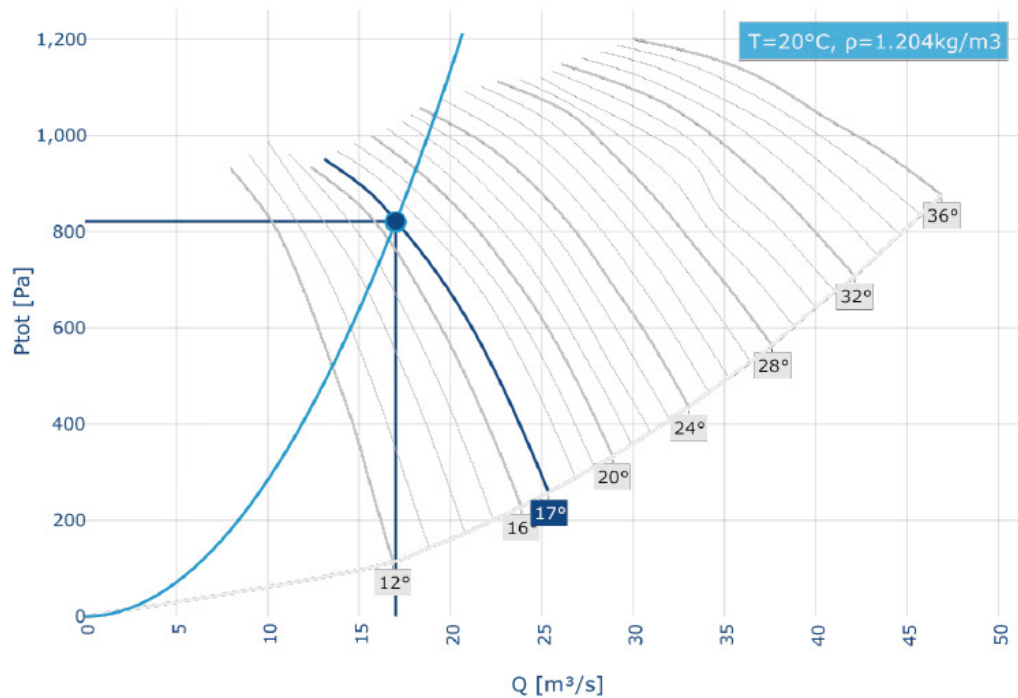
Figura 5 – Curva caratteristica del ventilatore VC
