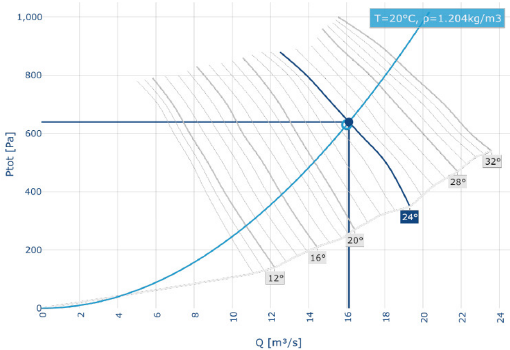
Figura 4 – Curva caratteristica dei ventilatori VF1/VF2
