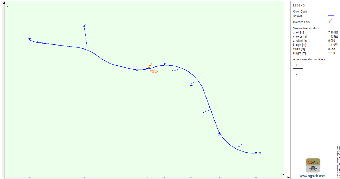
Figura A1-1 - Modello dispersore complessivo
