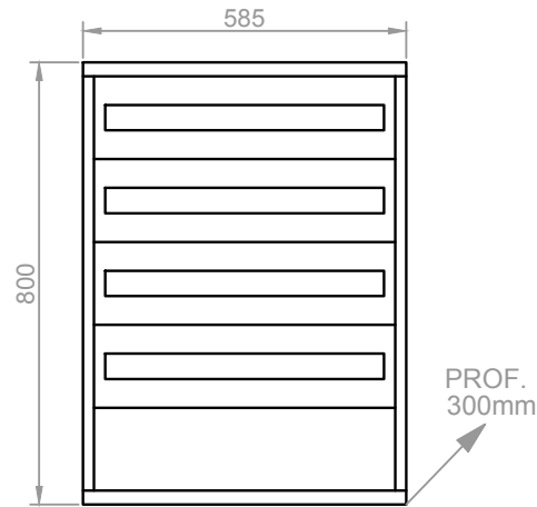
VISTA FRONTALE QUADRO INTERNO
