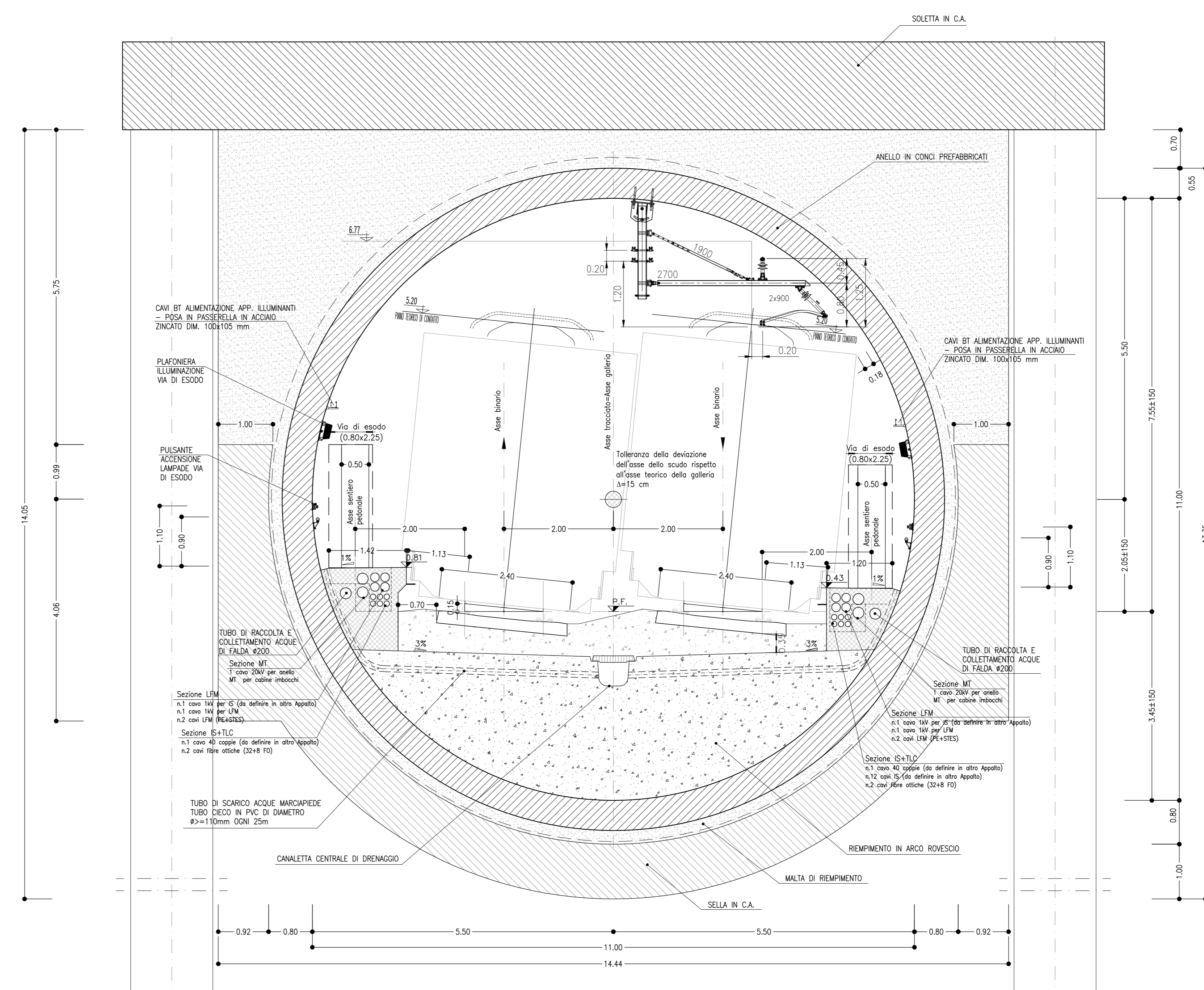
SEZIONE CONCIO SOTTO SOLETTONE SCALA 1:50
