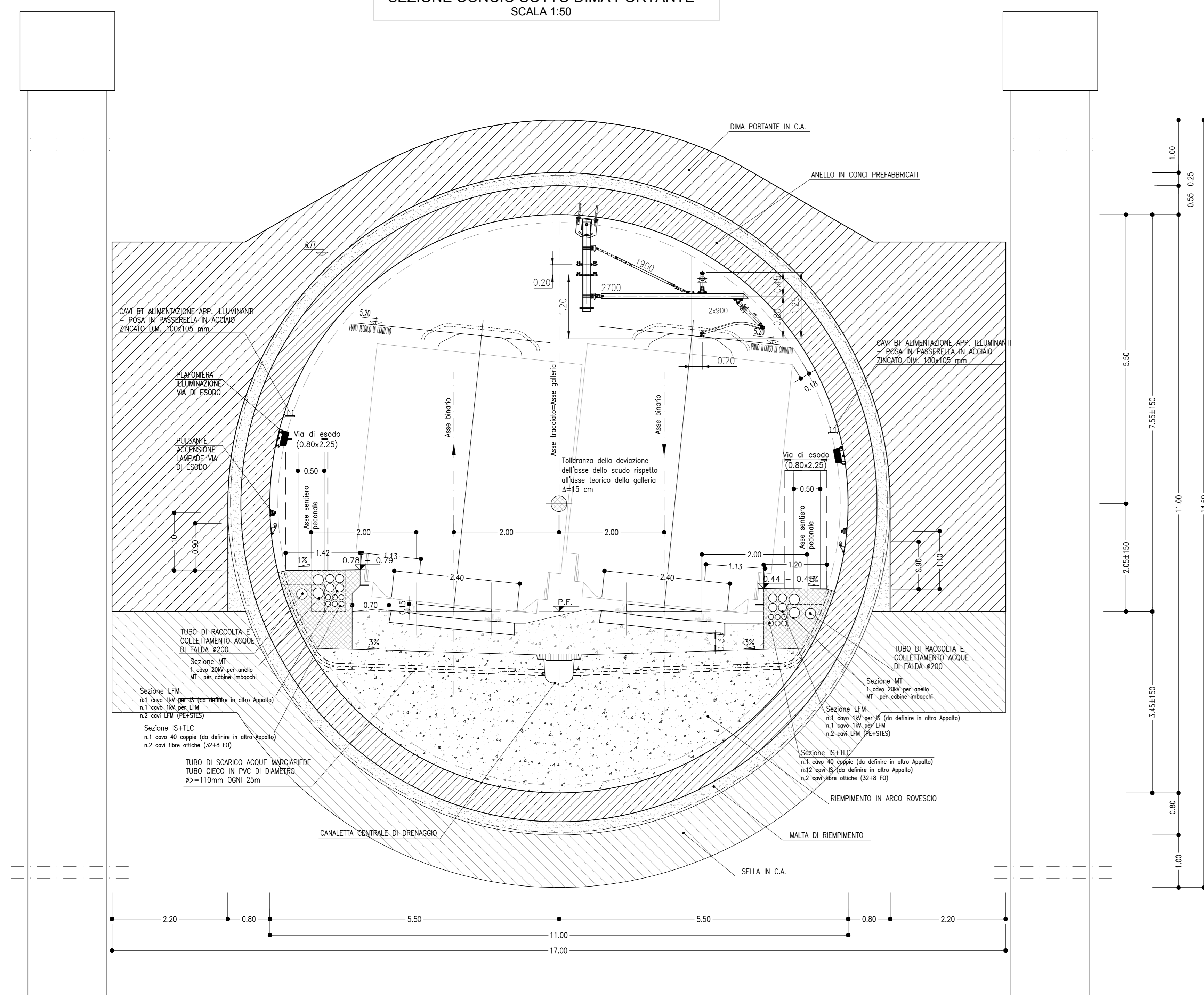
SEZIONE CONCIO SOTTO DIMA PORTANTE SCALA 1:50
