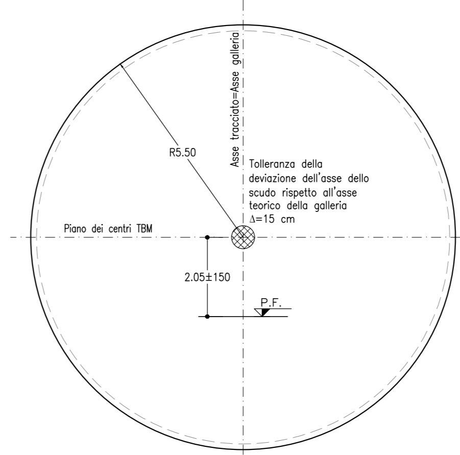
CARATTERISTICHE GEOMETRICHE SCALA 1:100
