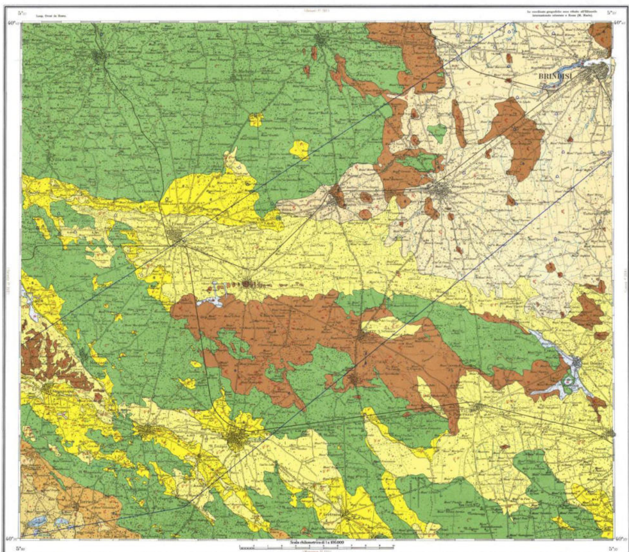
Foglio n° 203 della Carta D'Italia Scala 1:100.000 "BRINDISI" - Ubicazione dell'area indagata
