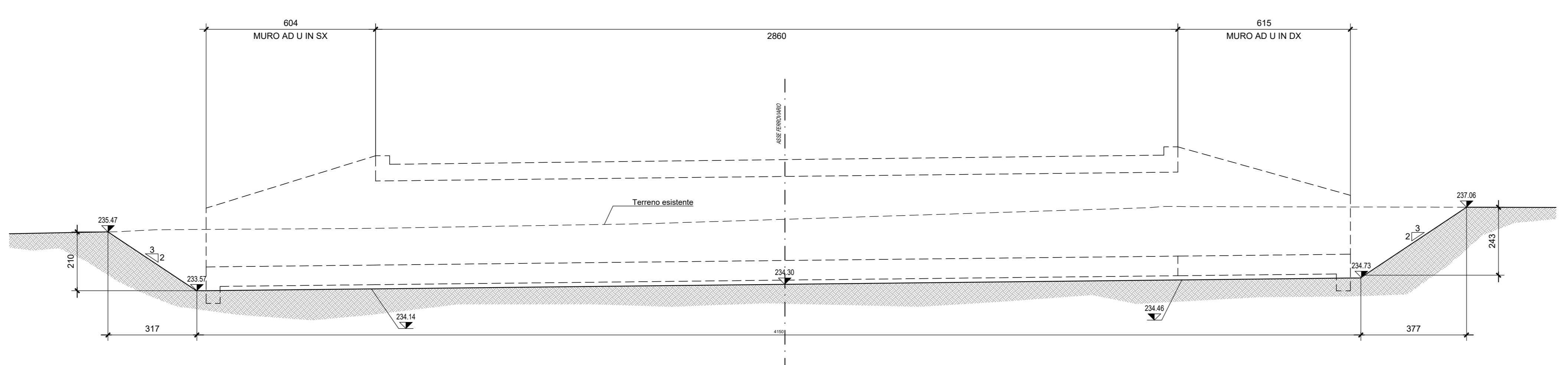
SEZIONE SCAVO A-A - SCALA 1:100
