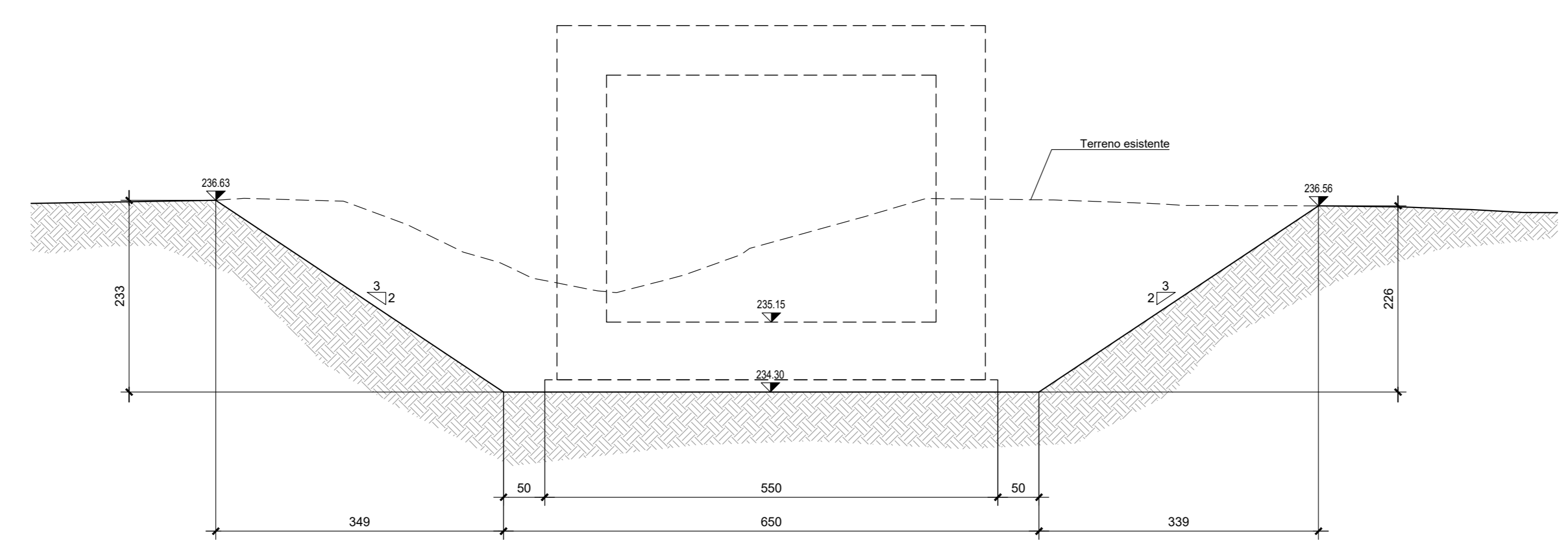
SEZIONE SCAVO B-B - SCALA 1:50
