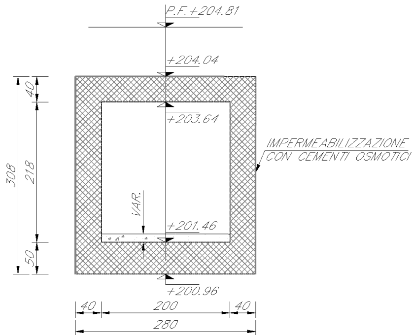
Figura 3 – Sezione trasversale C-C
