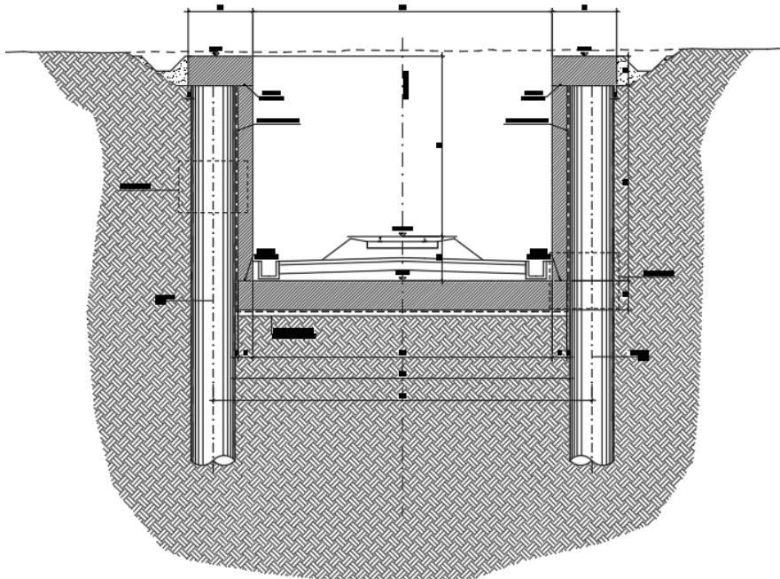
Fig. 2 – Sezione trasversale dell'opera TR10
