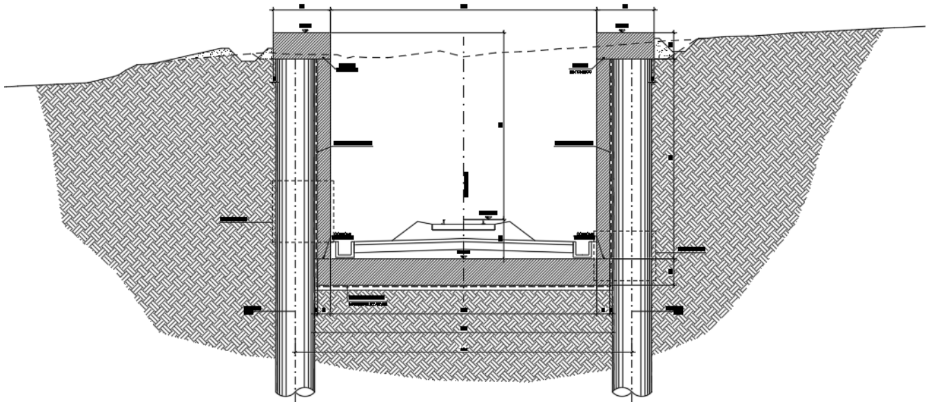
Fig. 1 – Sezione trasversale dell'opera TR09
