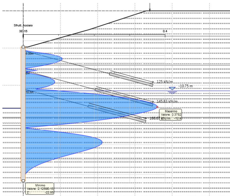
SLE – Tasso di sfruttamento acciaio
