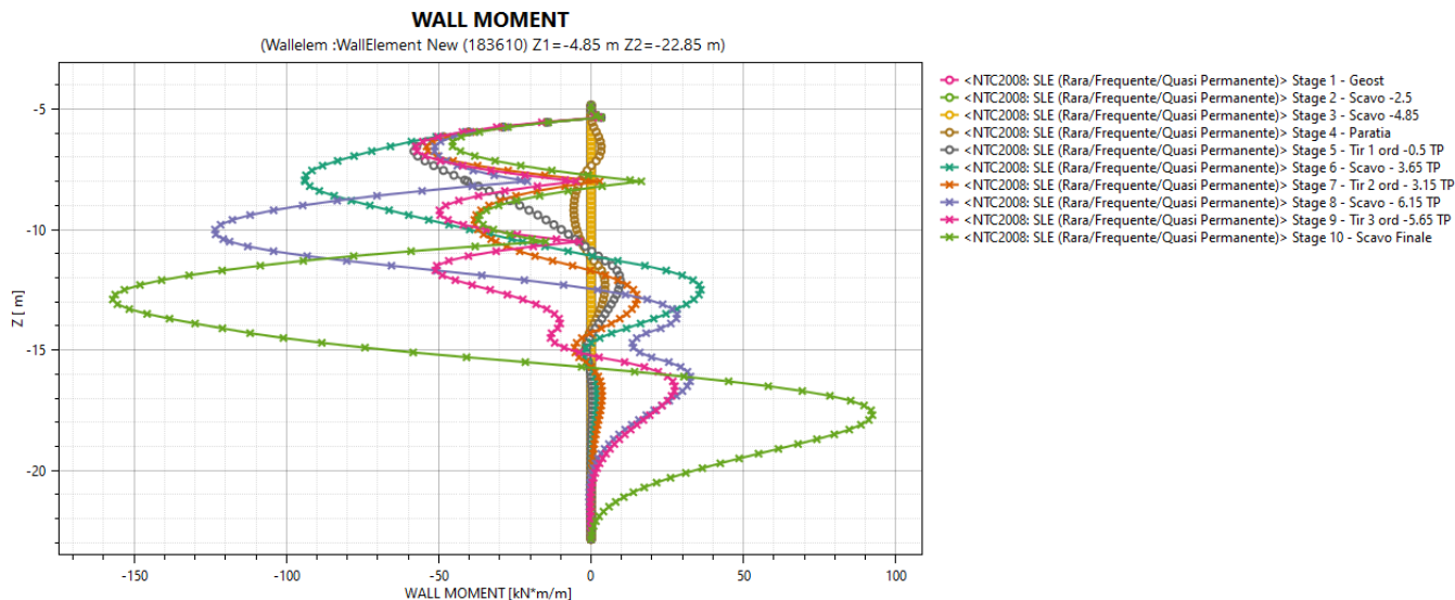
Momento flettente – SLE
