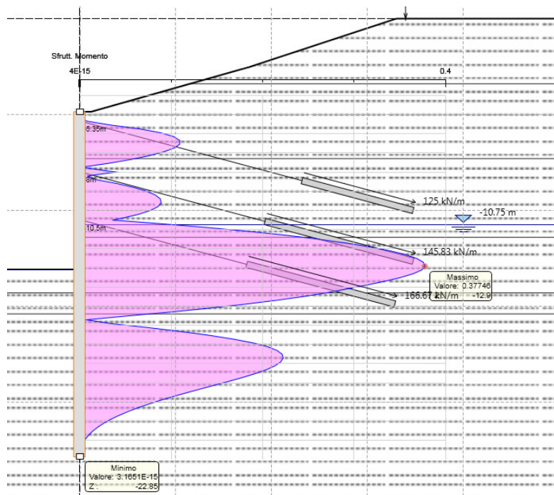
SLU – Tasso di sfruttamento a flessione
