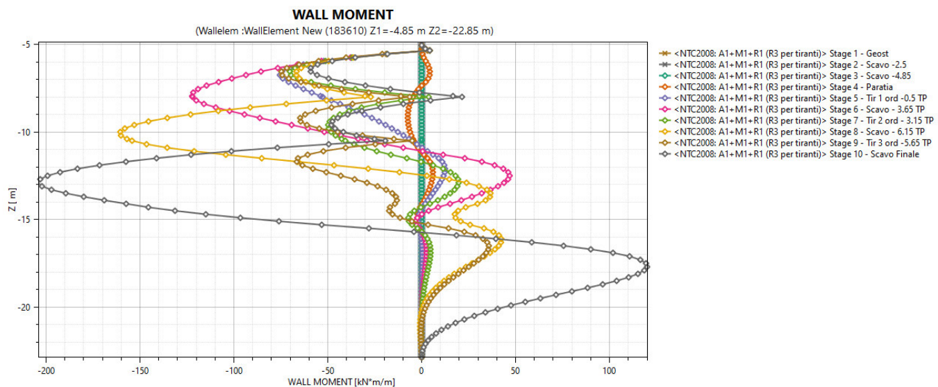
Momento flettente – A1-M1-R1
