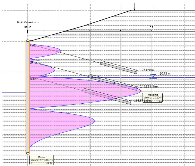
SLE – Tasso di sfruttamento calcestruzzo
