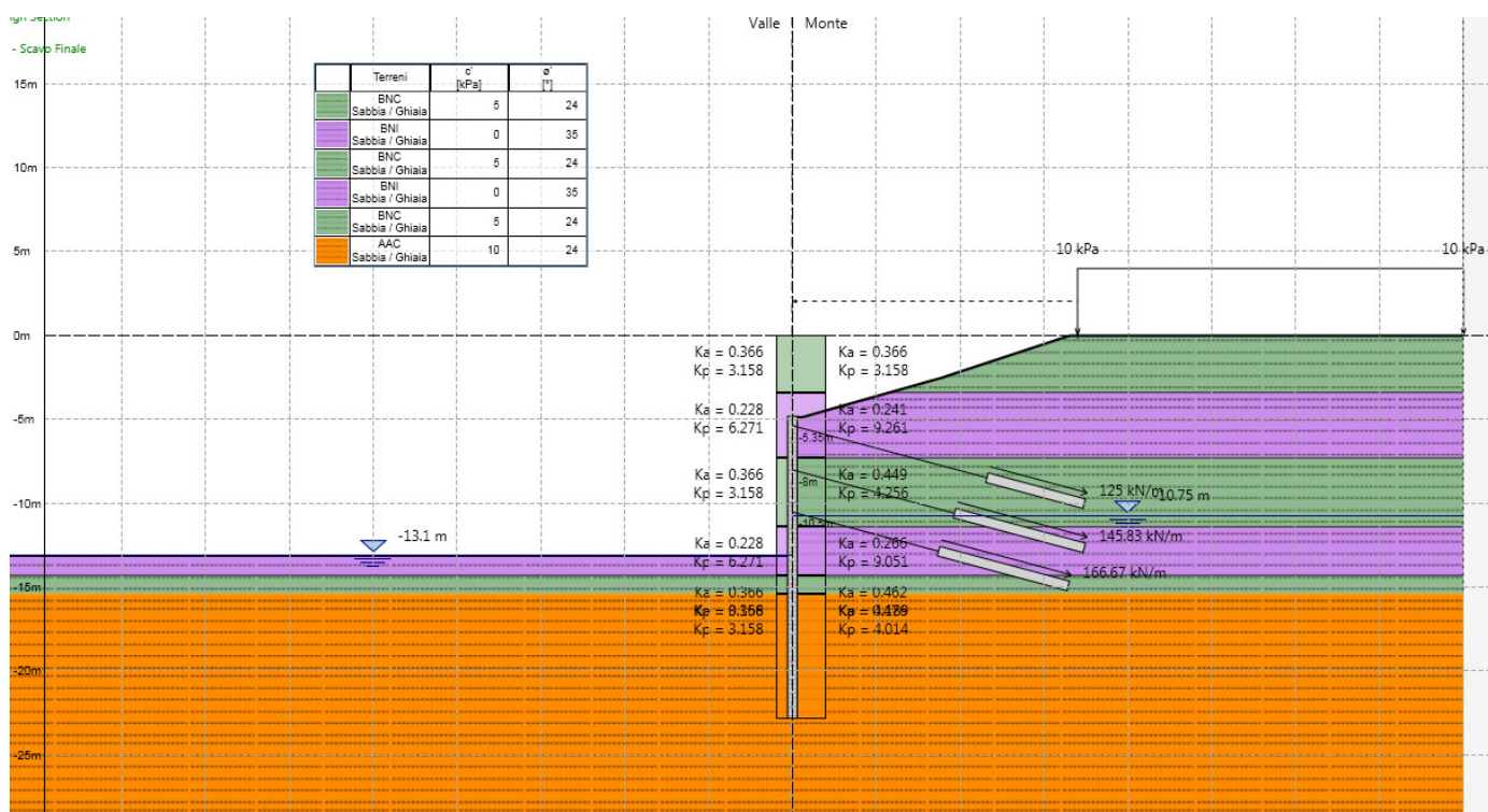
Modello Paratia (Fase finale)
