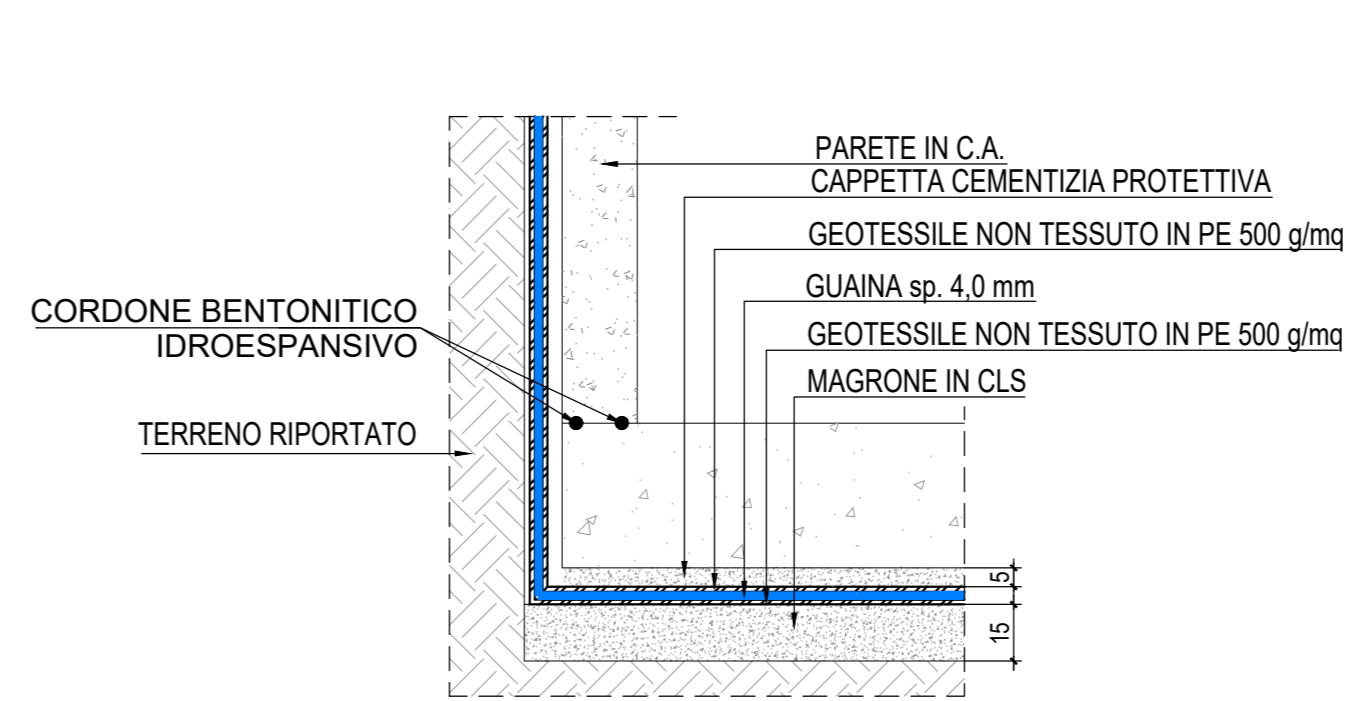
PARTICOLARE "3"-Scala 1:20 Impermeabilizzazione raccordo orizzontale verticale
