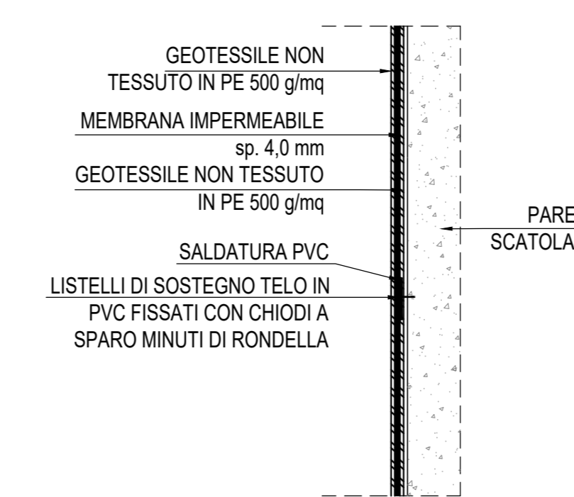
PARTICOLARE "2"-Scala 1:20 Impermeabilizzazione parete verticale
