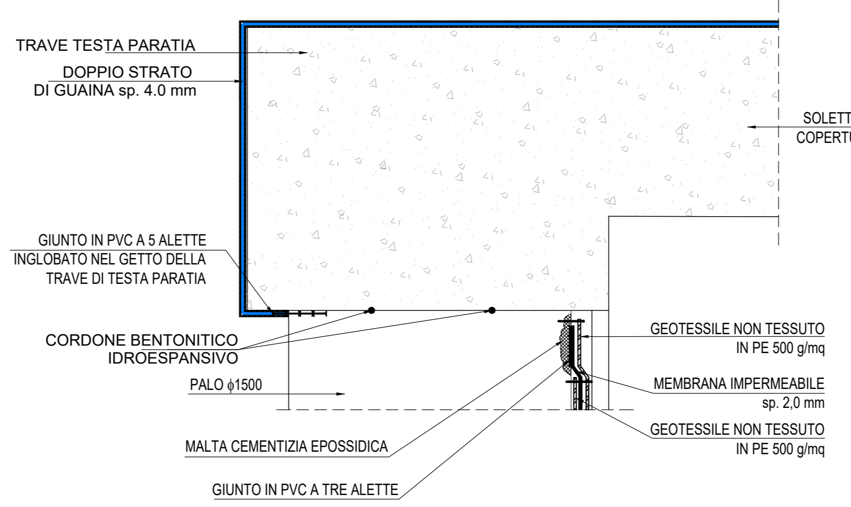
PARTICOLARE "2"-Scala 1:20 Impermeabilizzazione parete verticale
