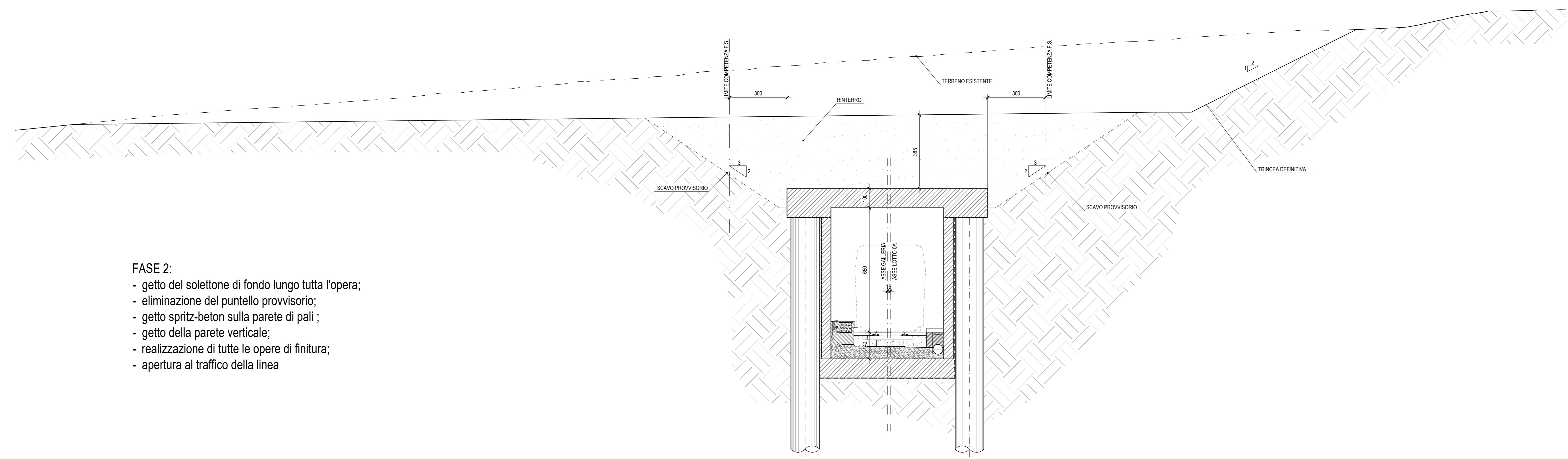
SEZIONE A-A Scala 1:100
