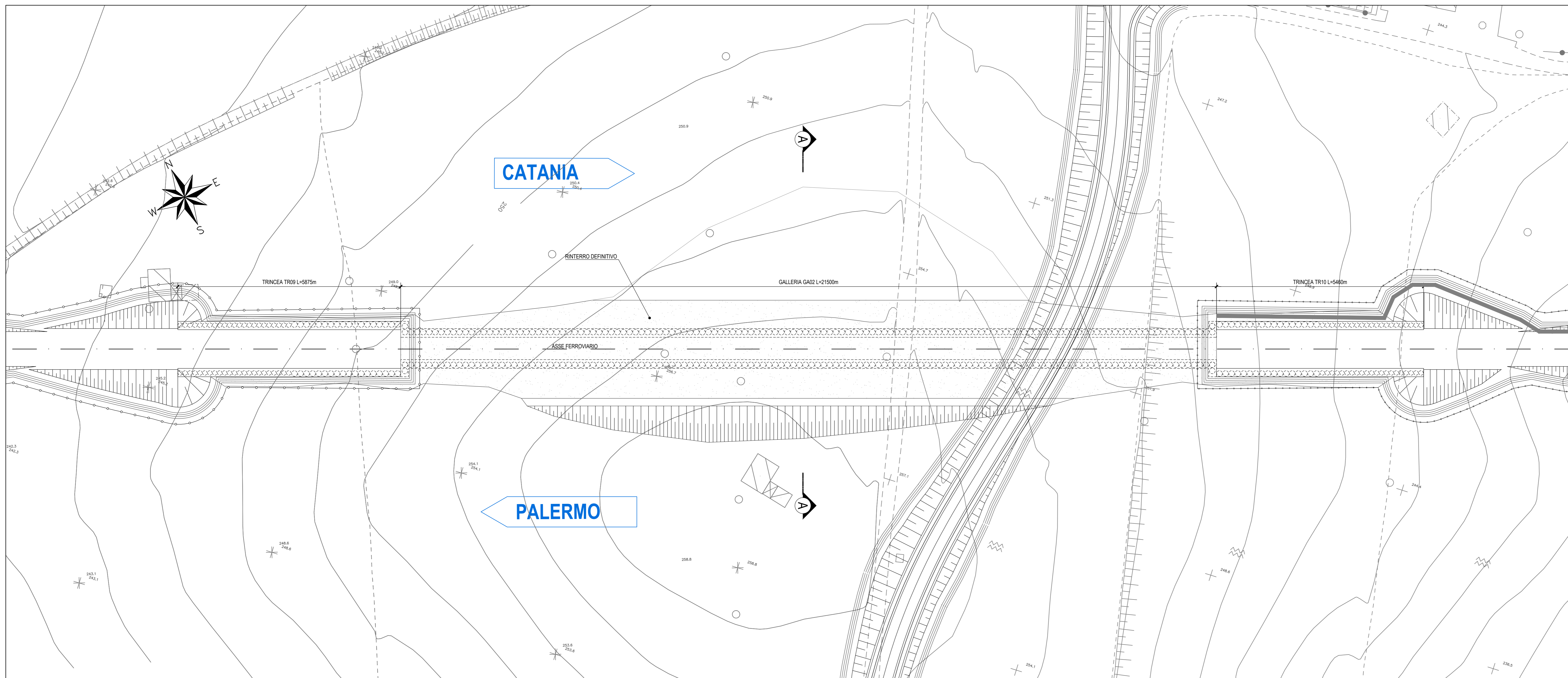
PLANIMETRIA RINTERRO - Scala 1:500
