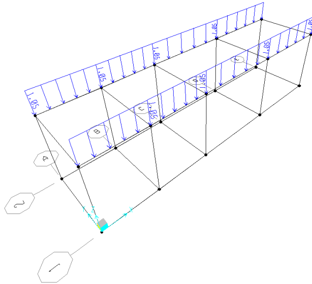
QH1 – Accidentali (Manutenzione)
