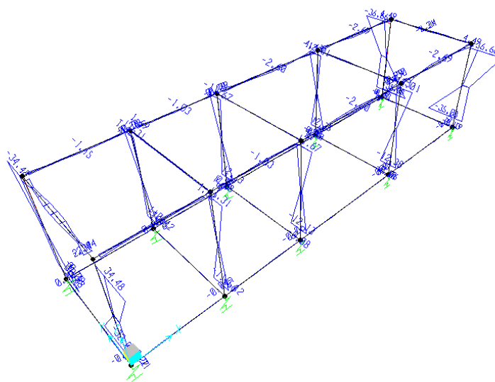
Momento M2 - Involuppo SLU
