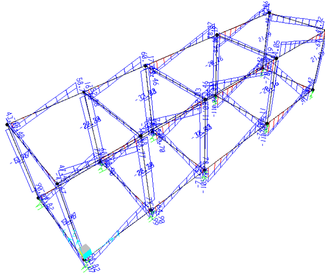
Taglio V2 - Involuppo SLV
