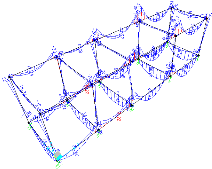
Momento M3 - Involuppo SLER
