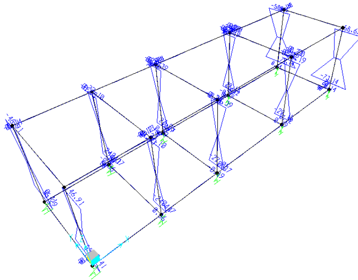
Momento M2 - Involuppo SLV
