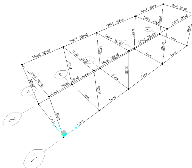
Figura 2: tipologia aste
