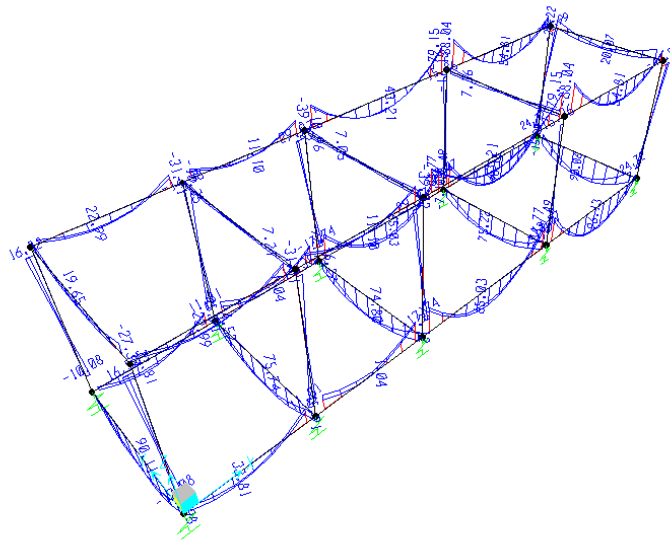
Momento M3 - Involuppo SLU
