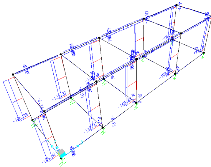
Sforzo Normale N - Involuppo SLV
