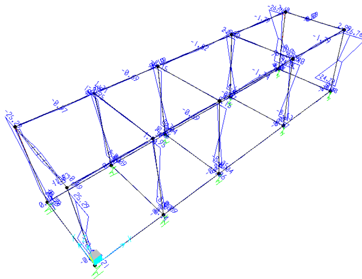
Momento M2 - Involuppo SLER
