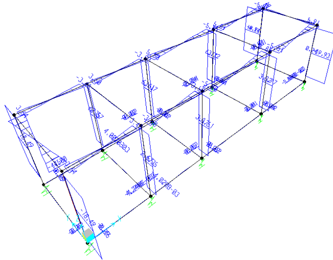
Taglio V3 - Involuppo SLU
