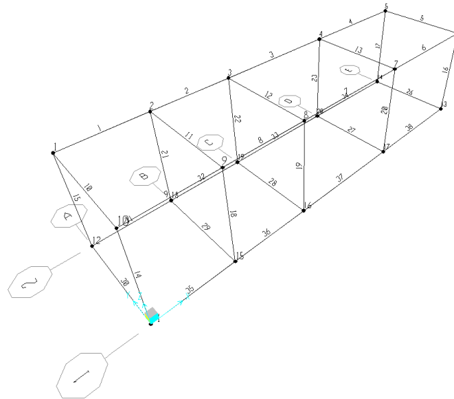
Figura 3: numerazione aste e nodi
