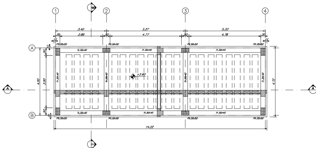
CARPENTERIA COPERTURA SCALA 1:50
