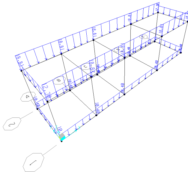
G2 – Permanenti non strutturali
