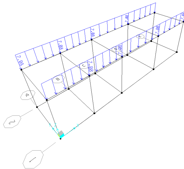
G1 – Peso solaio
