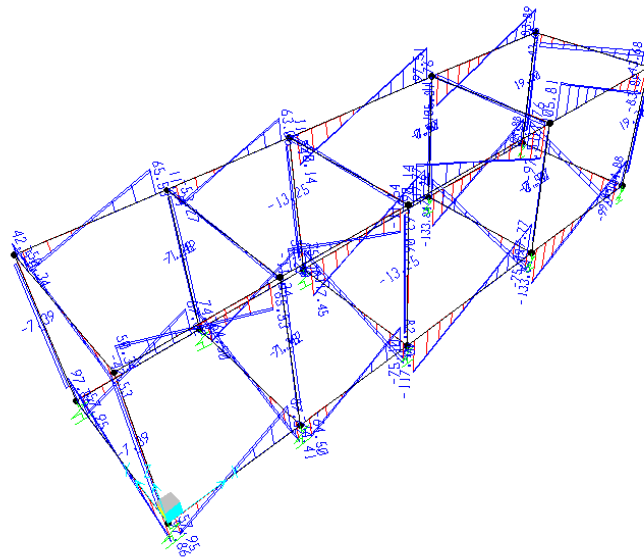
Taglio V2 - Involuppo SLU
