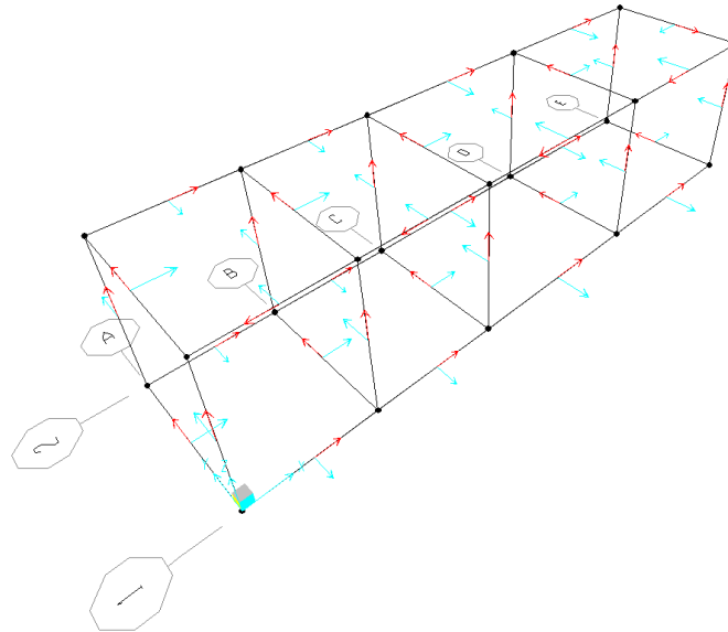
Figura 1: assi locali
