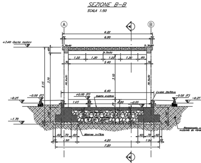
Figura 1-4. Sezione B
