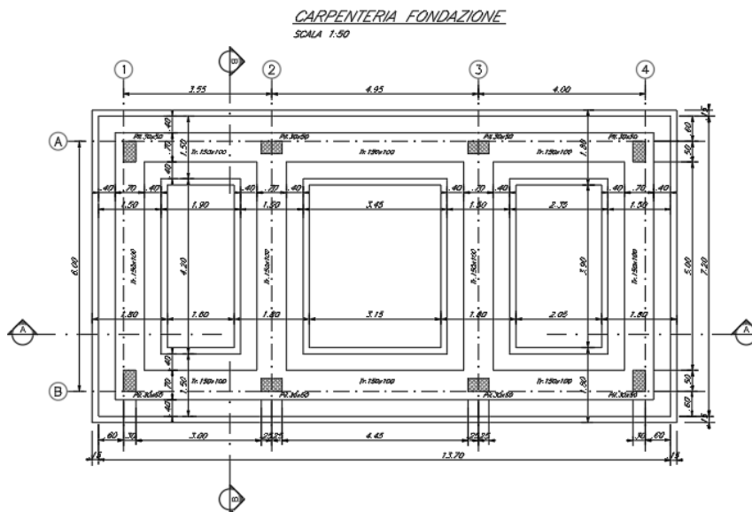
Figura 1-1. Carpenteria fondazioni.
