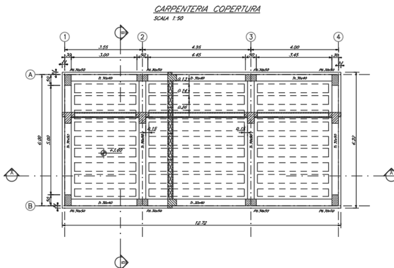
Figura 1-2. Carpenteria copertura.
