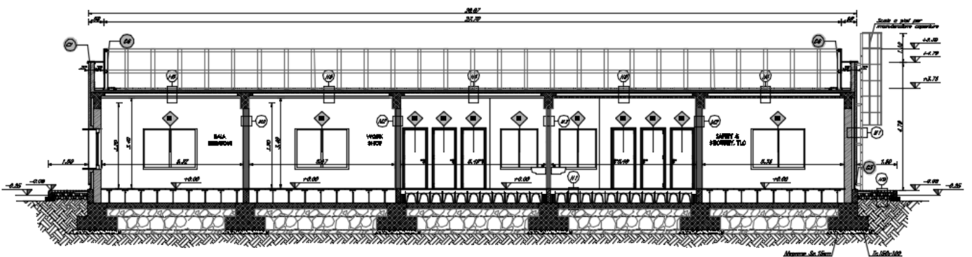
Figura 1-2. Sezione A
