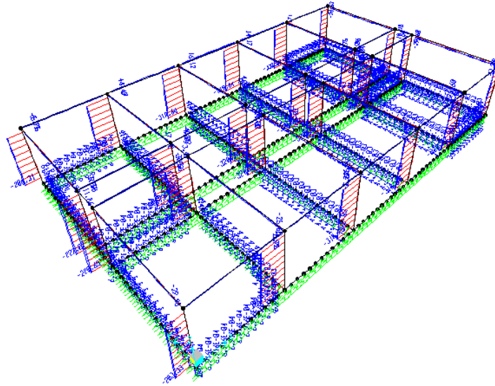
Sforzo Normale N - Involuppo SLU
