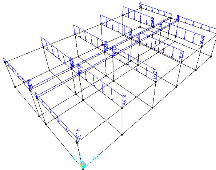
G1 – Peso solaio
