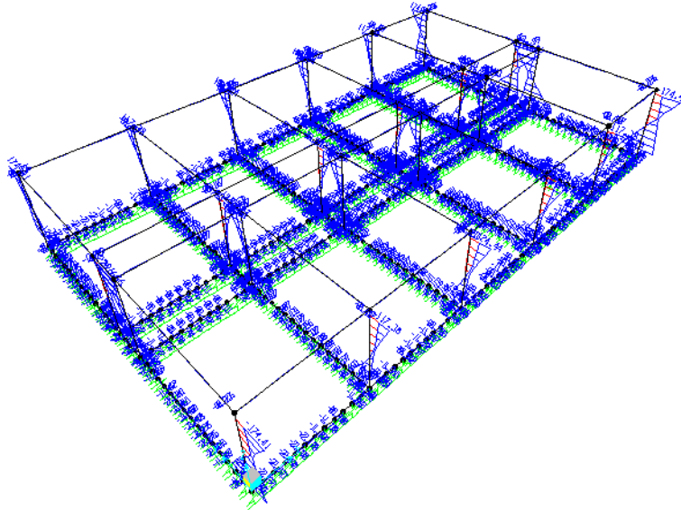
Momento M2 - Involuppo SLV
