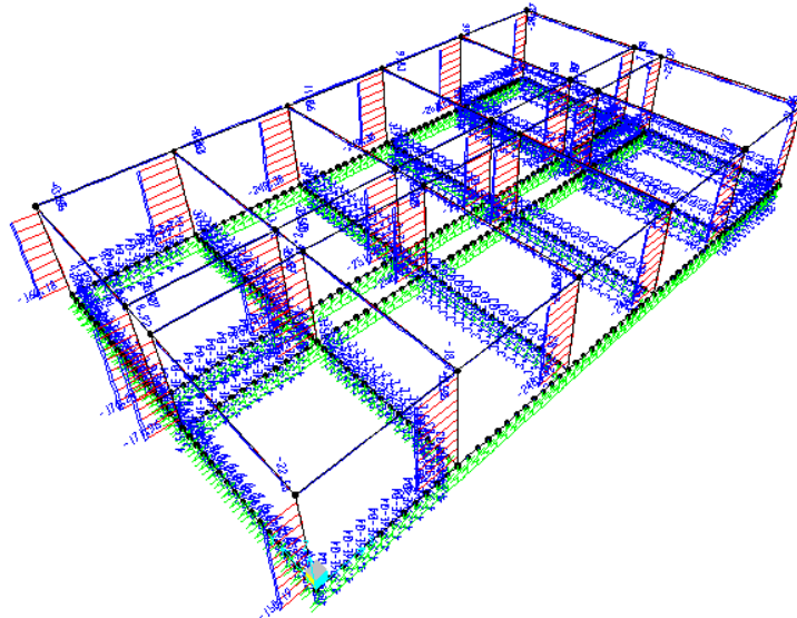
Sforzo Normale N - Involuppo SLER
