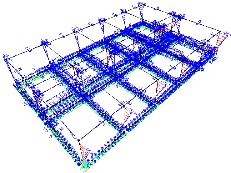
Momento M3 - Involuppo SLU
