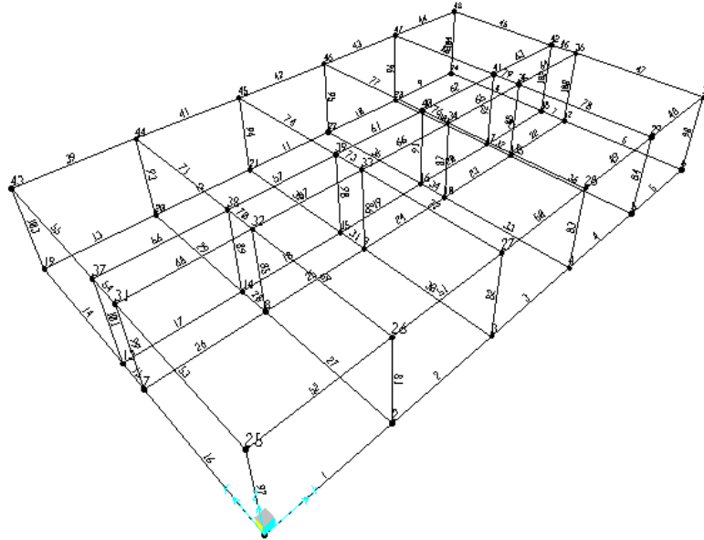
Figura 6: numerazione aste e nodi
