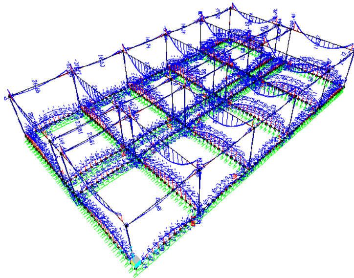
Momento M3 - Involuppo SLU
