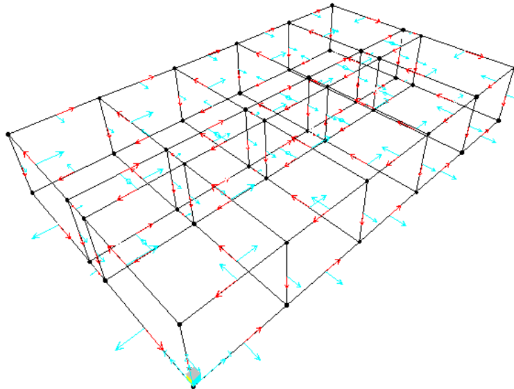
Figura 4: assi locali
