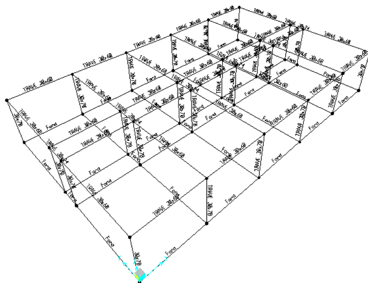
Figura 5: tipologia aste
