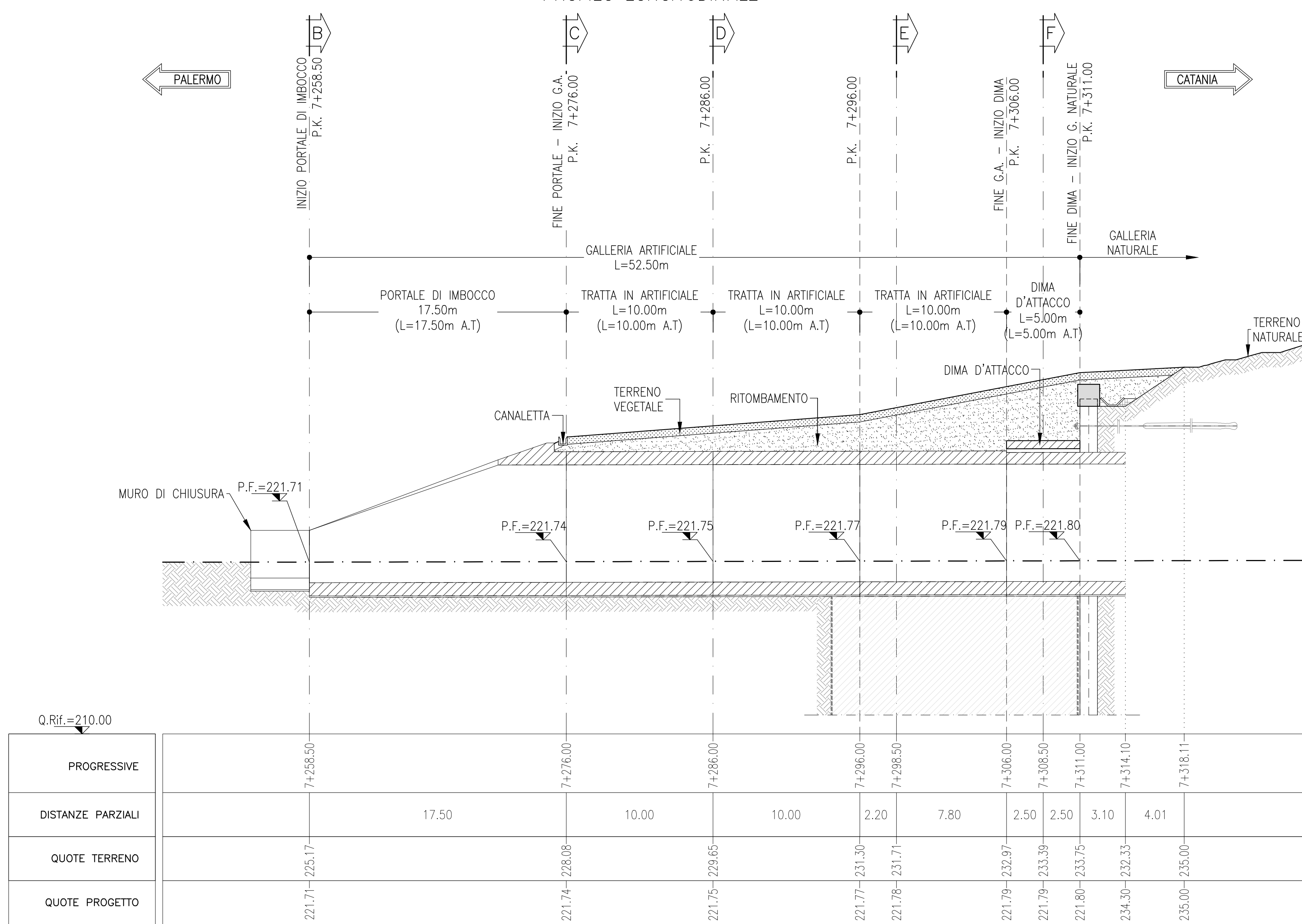
SEZIONE A-A SCALA 1:200 PROFILO LONGITUDINALE
