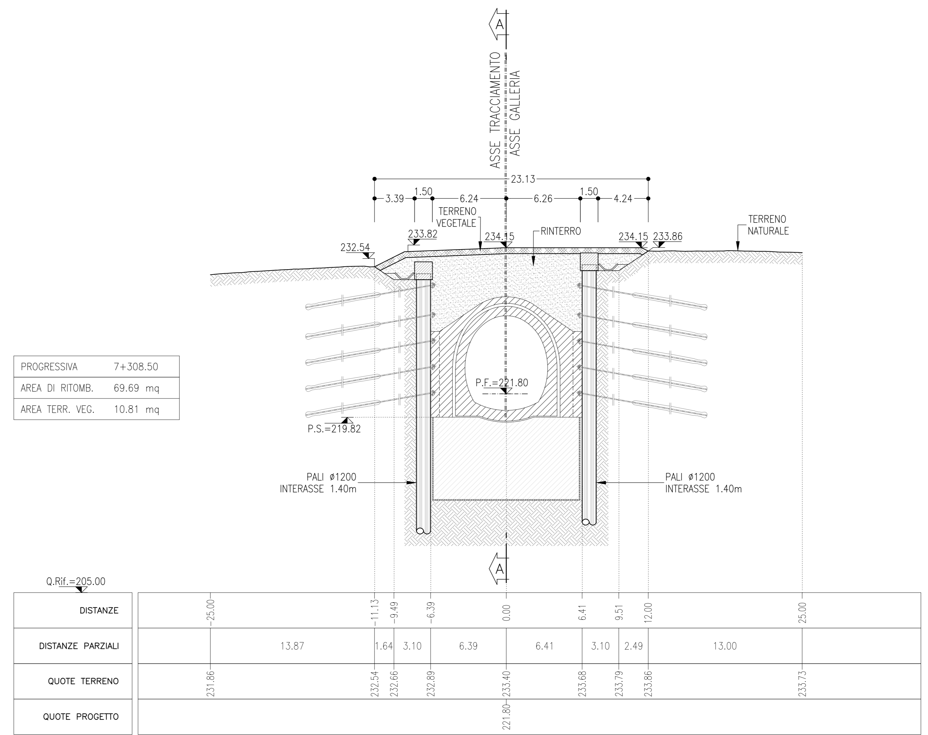
SEZIONE F-F SCALA 1:200 SEZIONE TRASVERSALE
