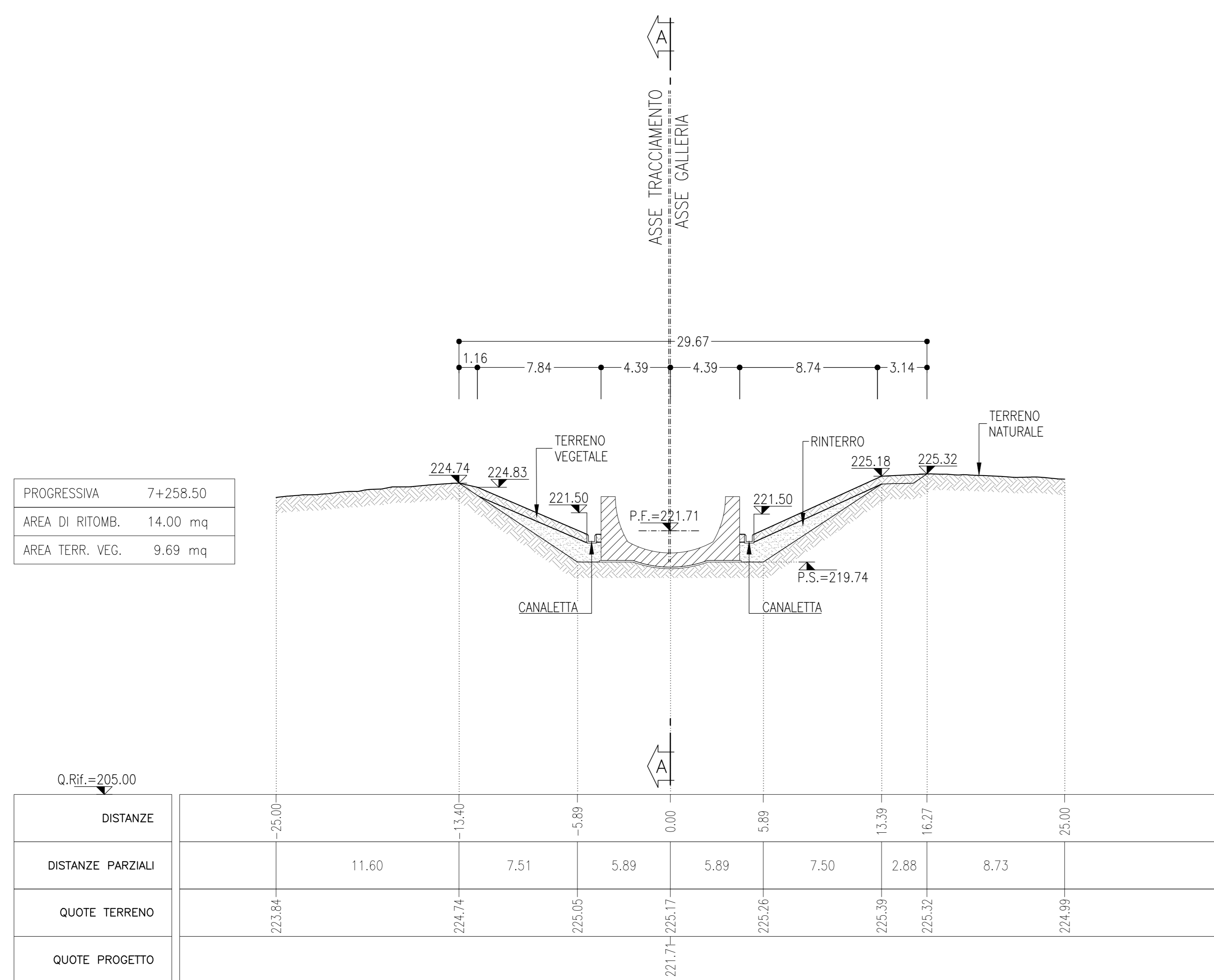
SEZIONE B-B SCALA 1:200 SEZIONE TRASVERSALE
