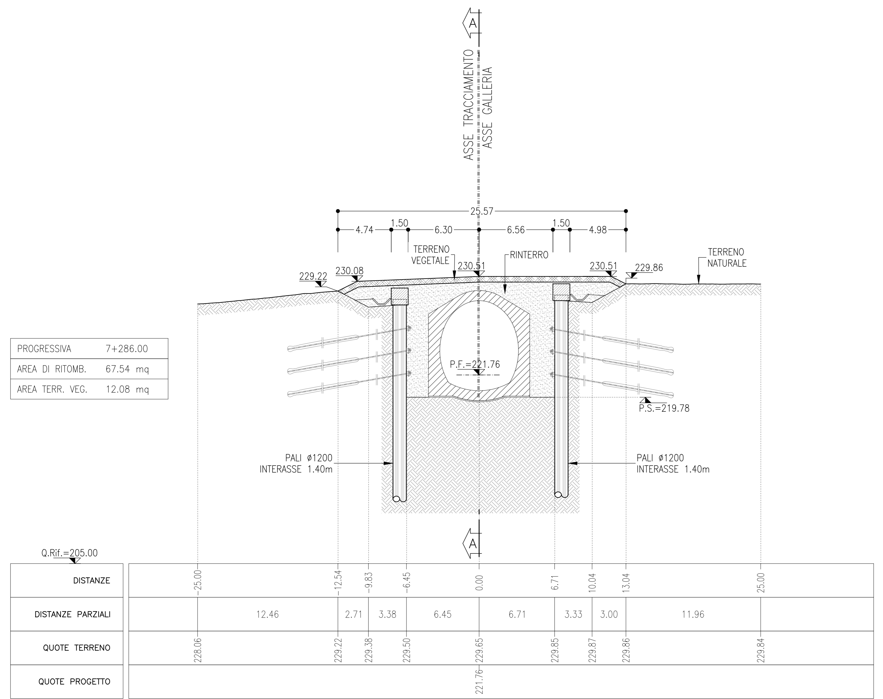
SEZIONE D-D SCALA 1:200 SEZIONE TRASVERSALE
