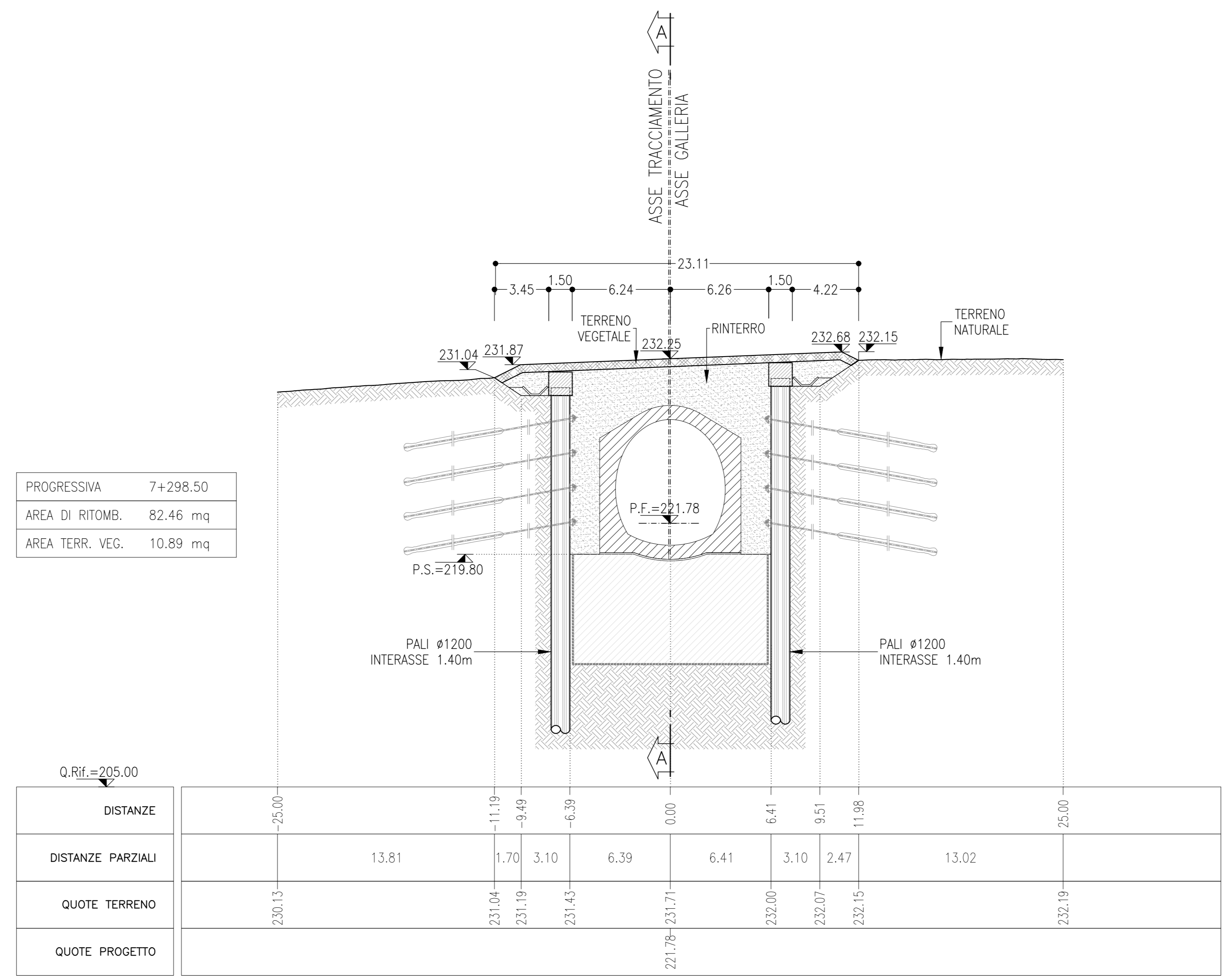
SEZIONE E-E SCALA 1:200 SEZIONE TRASVERSALE
