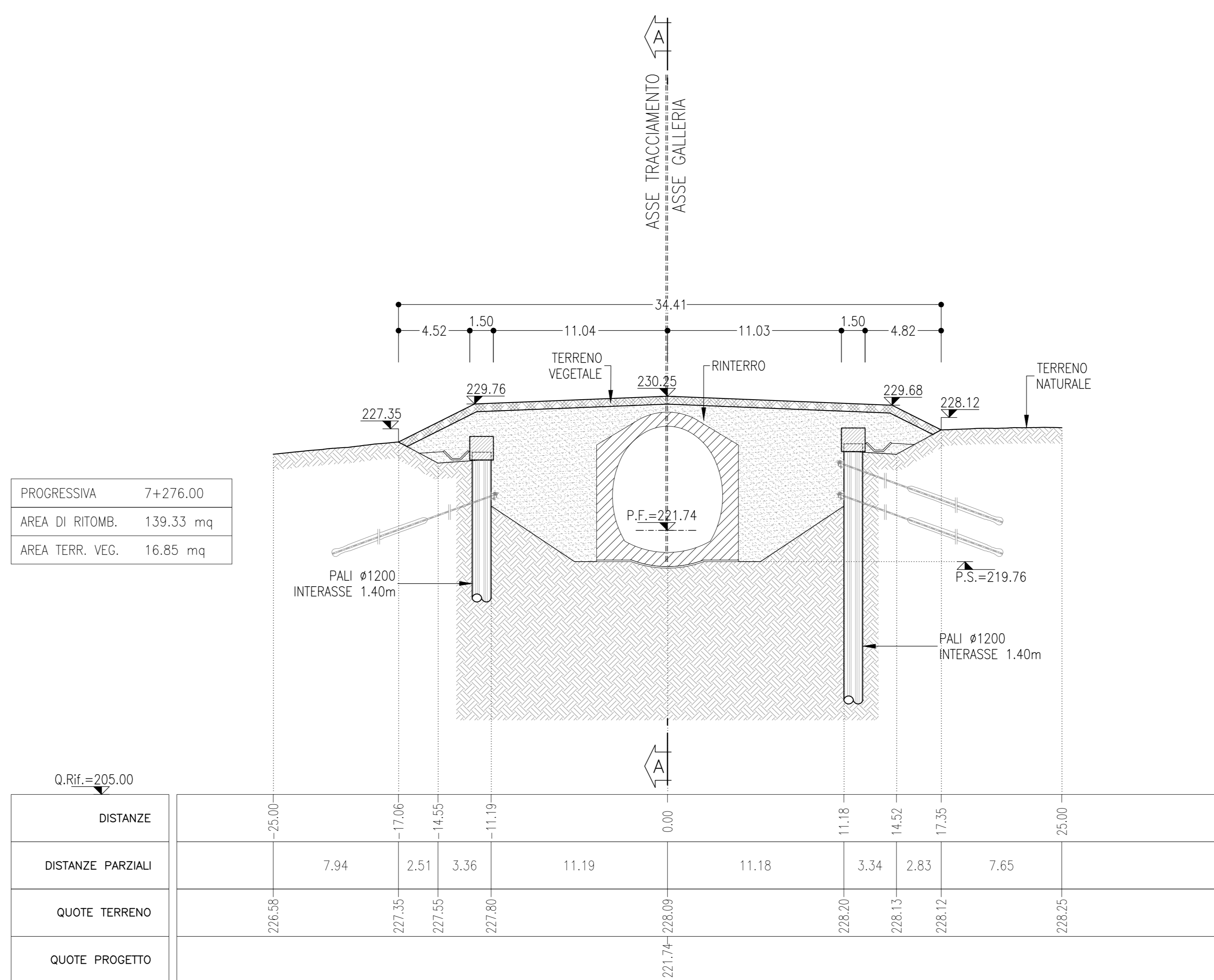
SEZIONE C-C SCALA 1:200 SEZIONE TRASVERSALE
