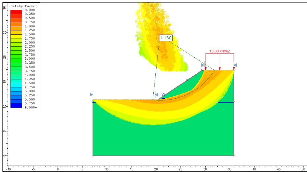
Figura 5. Analisi statica – Scarpare provvisorie –trincea H=6m – terreni incoerenti
