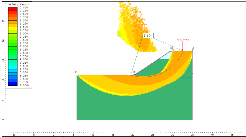
Figura 4. Analisi statica – Scarpare provvisorie –trincea H=6m – terreni coesivi
