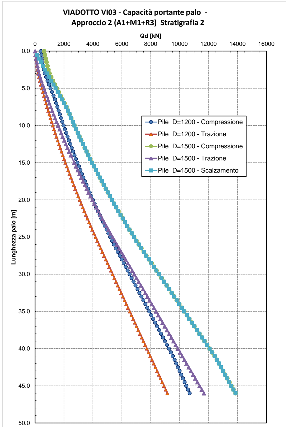
Figura 6 – Capacità portante palo Stratigrafia 2
