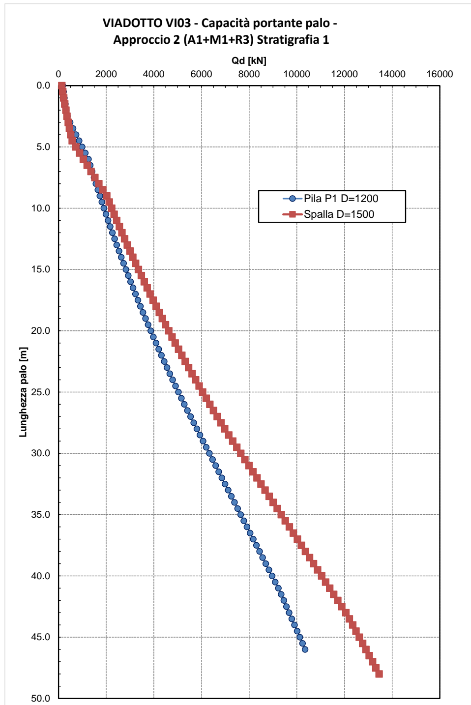
Figura 5 – Capacità portante palo Stratigrafia 1
