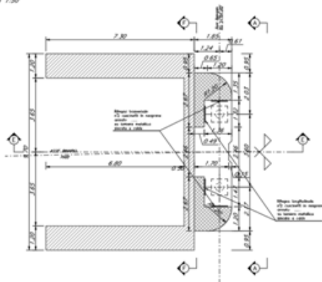
SEZIONE C-C Scala 1:50
