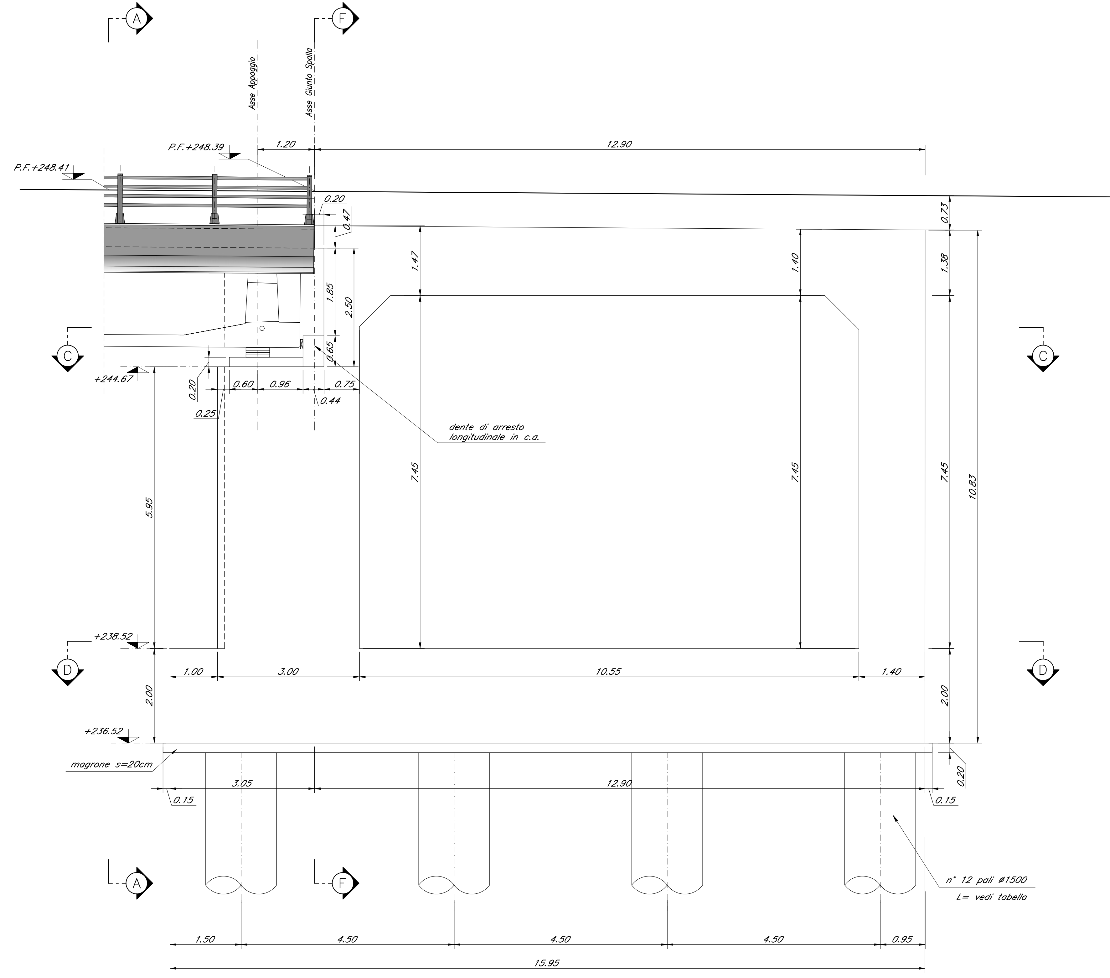
SEZIONE B-B Scala 1:50
