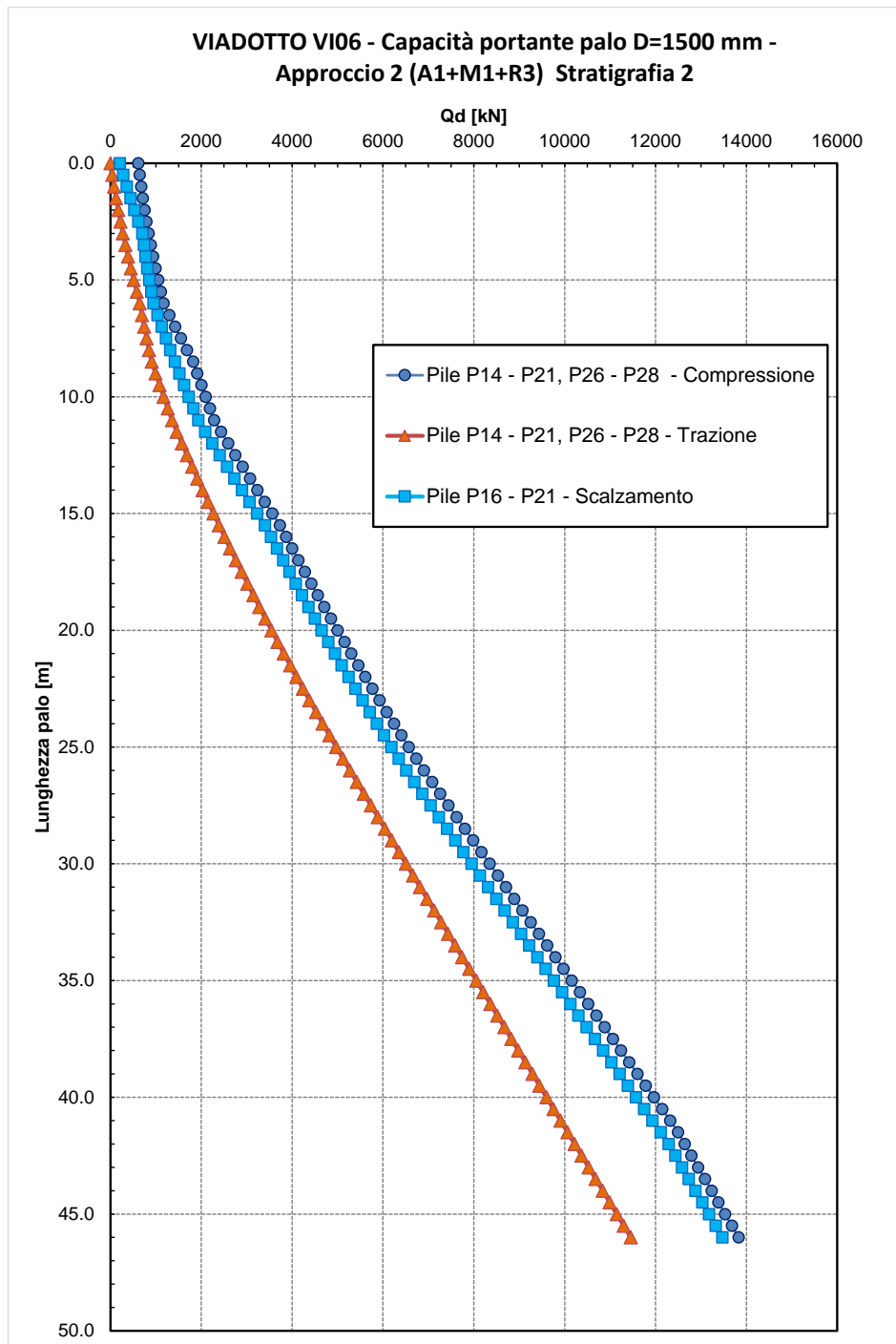
Figura 10 – Capacità portante pali - stratigrafia 2
