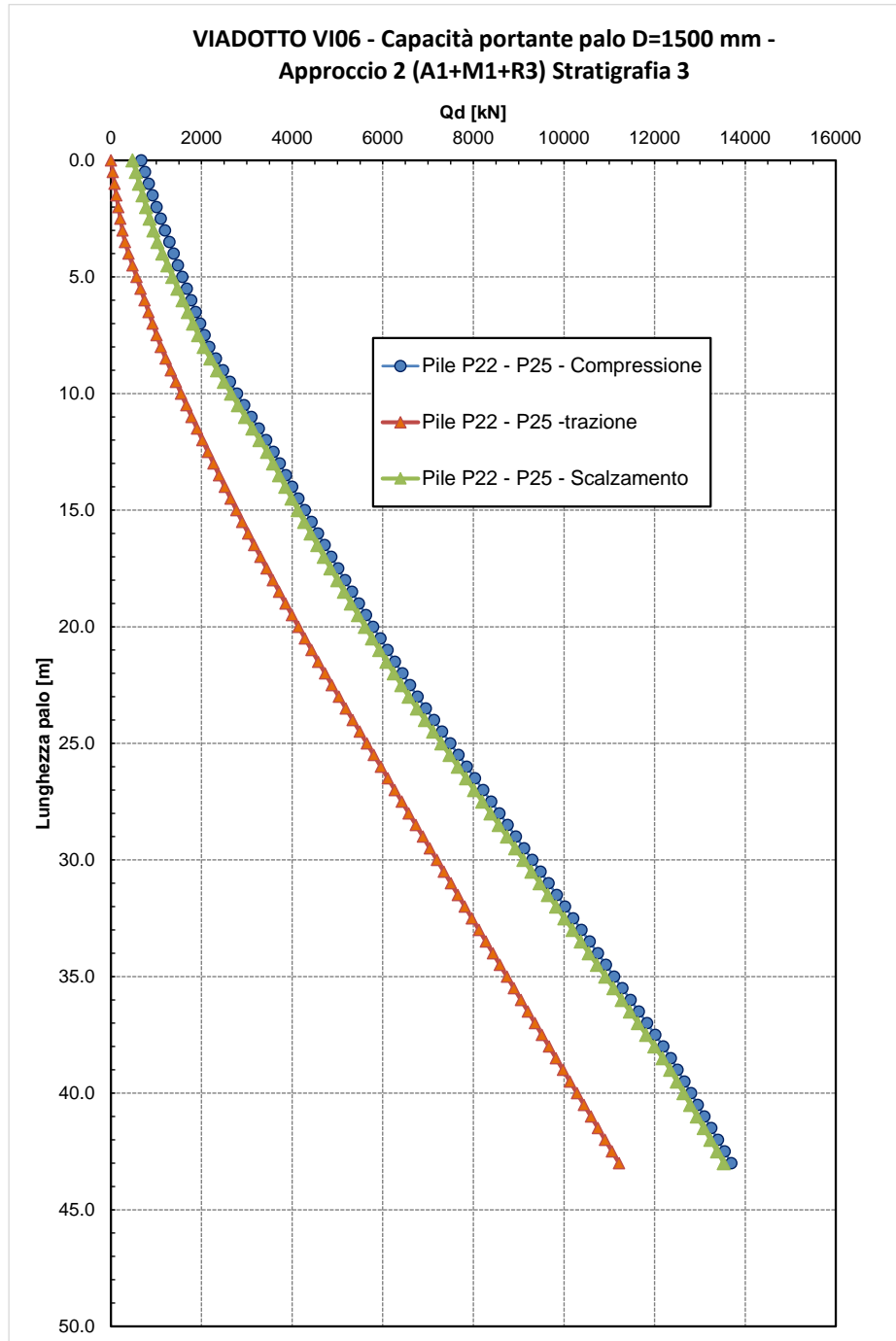
Figura 11 – Capacità portante pali - stratigrafia 3
