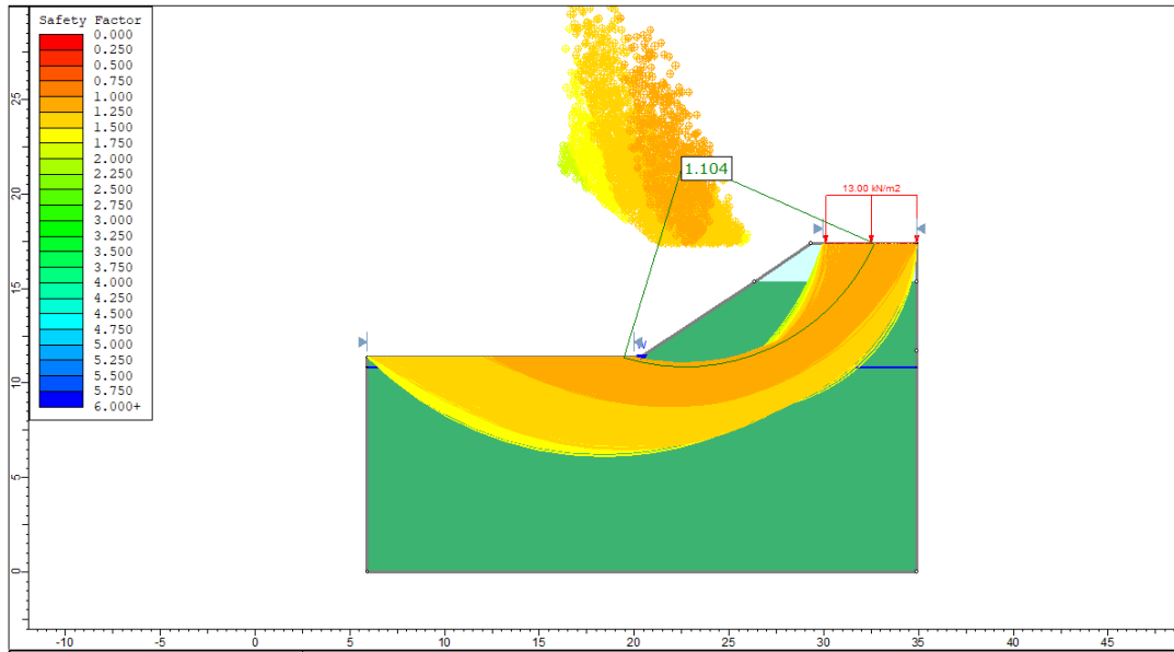
Figura 3. Analisi statica – Scarpate provvisorie –trincea H=6m – terreni coesivi
