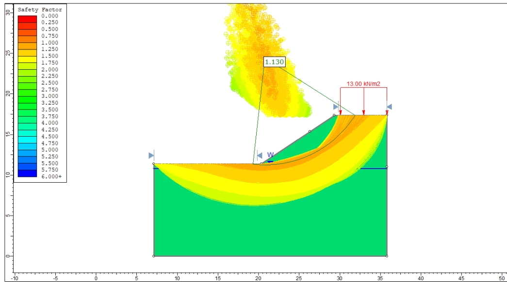
Figura 4. Analisi statica – Scarpate provvisorie –trincea H=6m – terreni incoerenti
