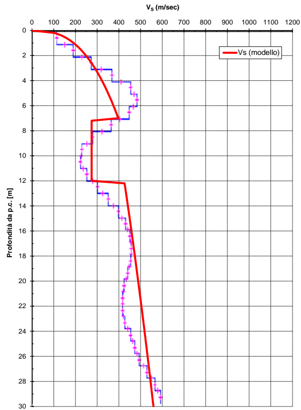
Figura 20. Velocità delle onde di taglio da prove geotecniche e legge di modello
