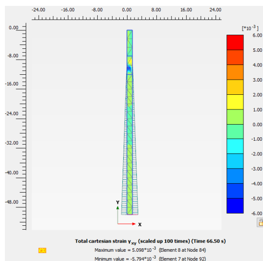
Figura 23. - Parametro \gamma_{07} che regola il decadimento del modulo a taglio con la deformazione tangenziale
