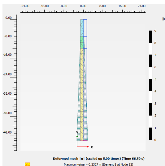
Figura 22. Spostamento massimo
