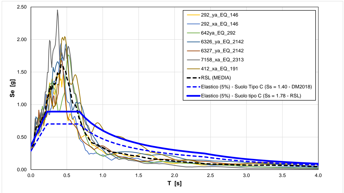
Figura 25. Spettri elastici
