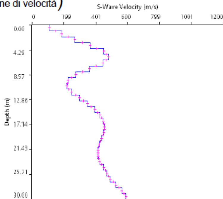
Figura 1 – Masw – VI10 (ex VI02)
