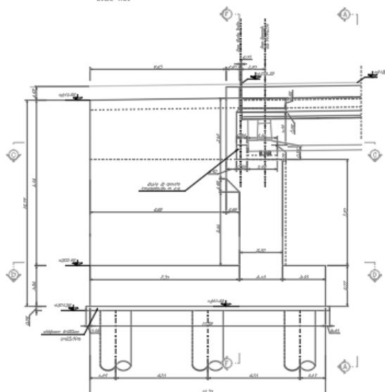
VISTA B-B Scala 1:50
