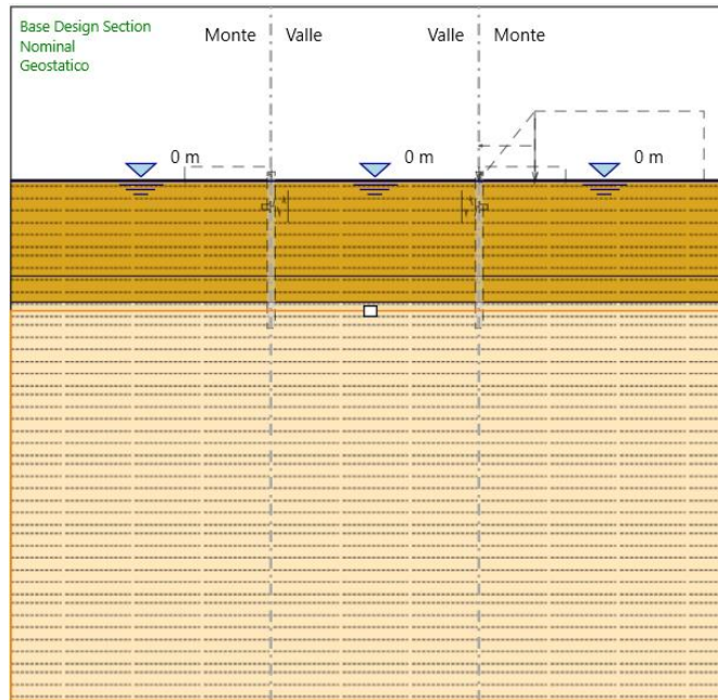
FASE 0: Generazione stato tensionale iniziale
