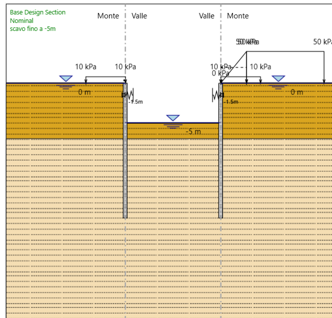
FASE 5: Scavo fino ad arrivare a 5 m da p.c.
