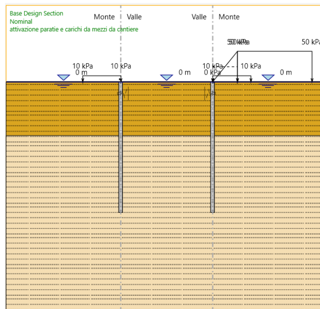
FASE 1: Installazione delle paratie di pali + attivazione carico di cantiere q_{acc}=10.0 kPa +attivazione carico trapezoidale che simula il terreno
