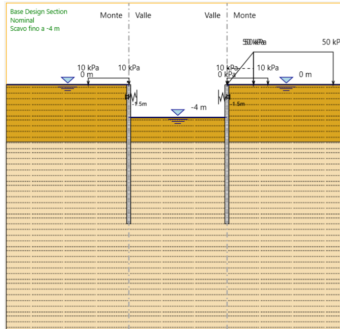
FASE 4: Scavo fino ad arrivare a 4m da p.c.
