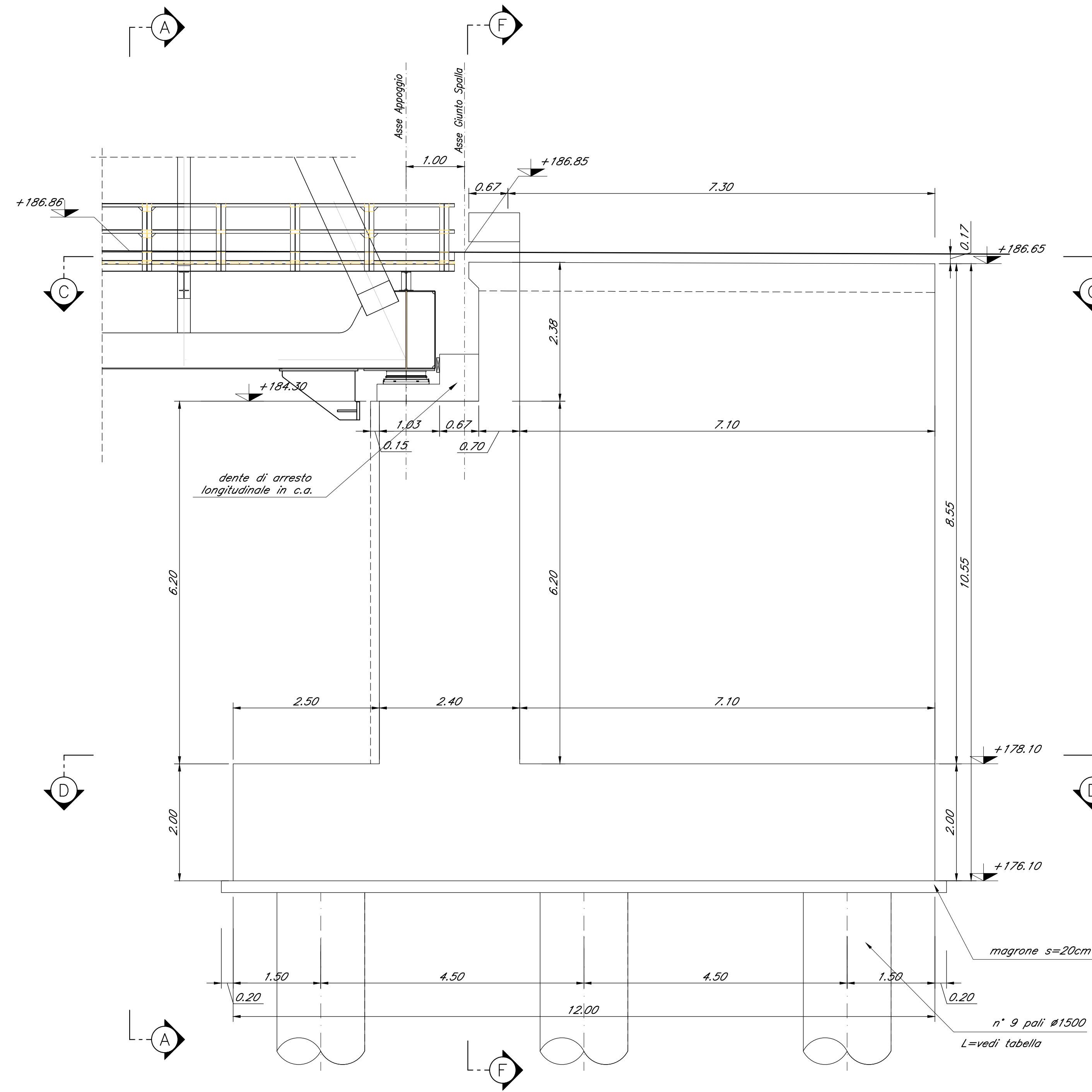
CARPENTERIA SPALLA B BINARIO PARI Scala 1:50
