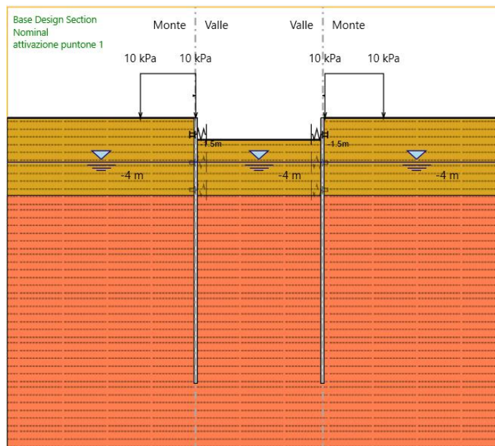
FASE 3: Installazione dei puntoni, con relative travi di ripartizione dei carichi, a 1.5 metro dalla testa della paratia
