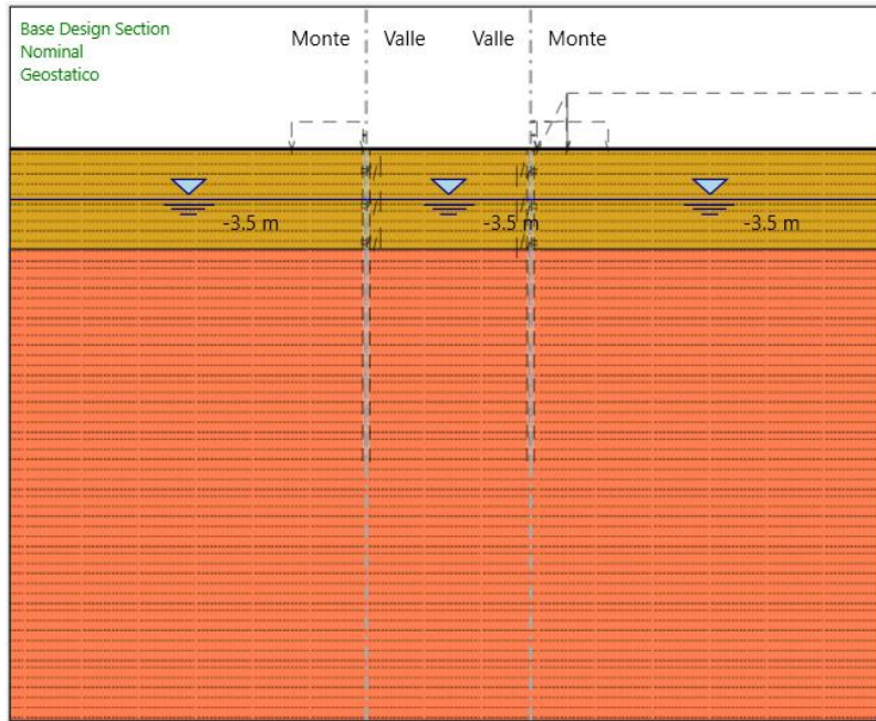
FASE 0: Generazione stato tensionale iniziale
