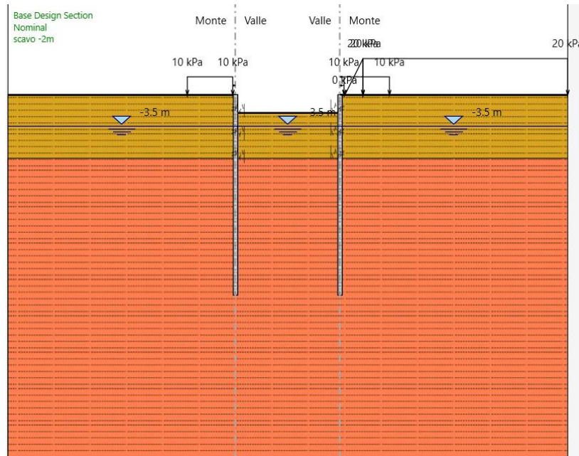
FASE 2: Scavo fino a arrivare a 2m dal p.c.
