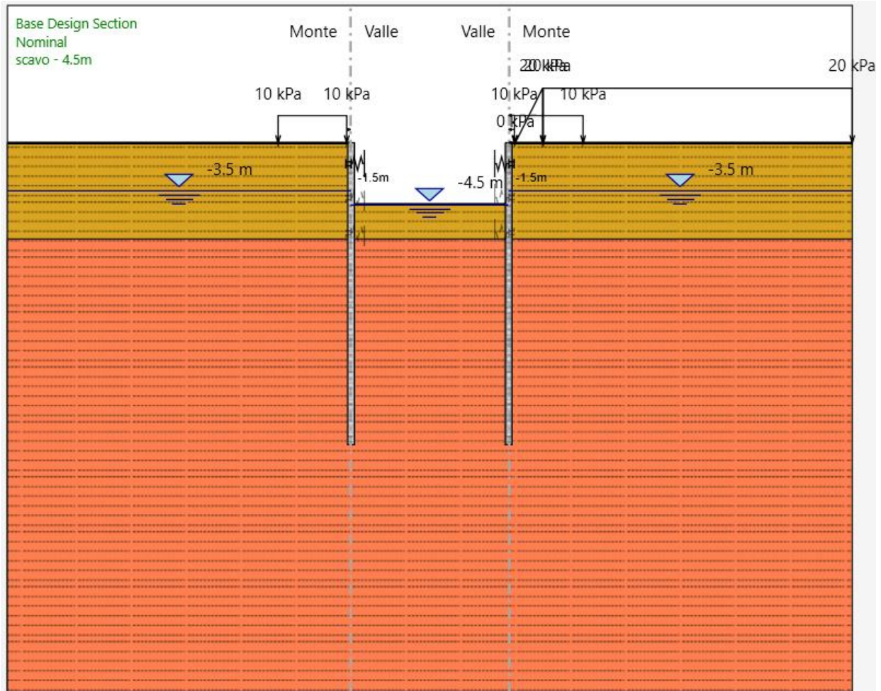
FASE 5: Scavo fino ad arrivare a 4.5m da p.c.
