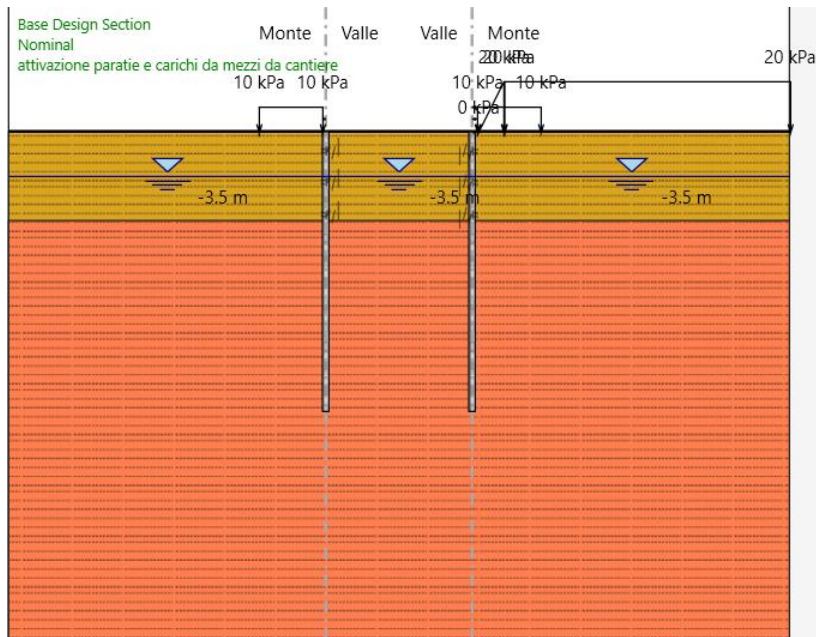
FASE 1: Installazione delle paratie di pali + attivazione carico di cantiere q_{acc}=10.0 \text{ kPa}
