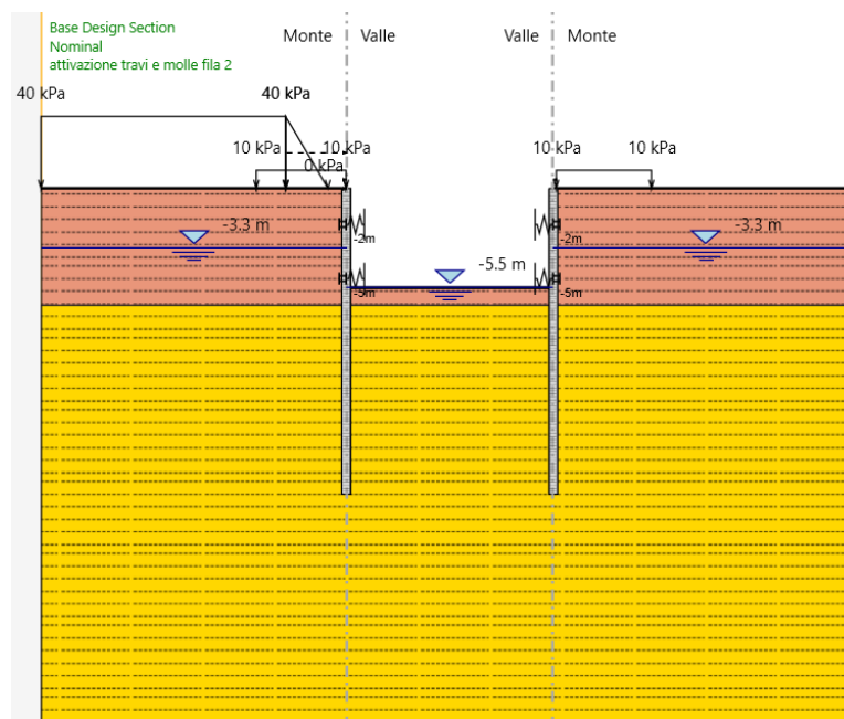
FASE 6: Installazione dei puntoni, con relative travi di ripartizione dei carichi, a 5 metri dalla testa della paratia
