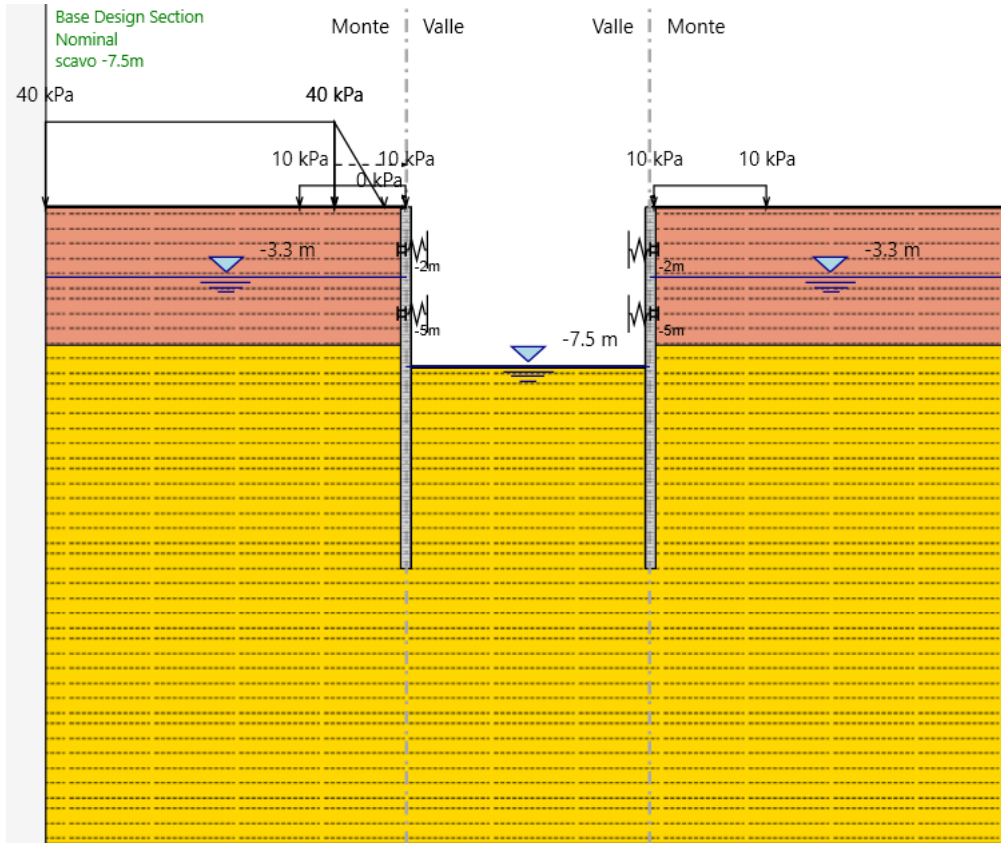
FASE 7: Scavo fino ad arrivare a 8m da p.c.
