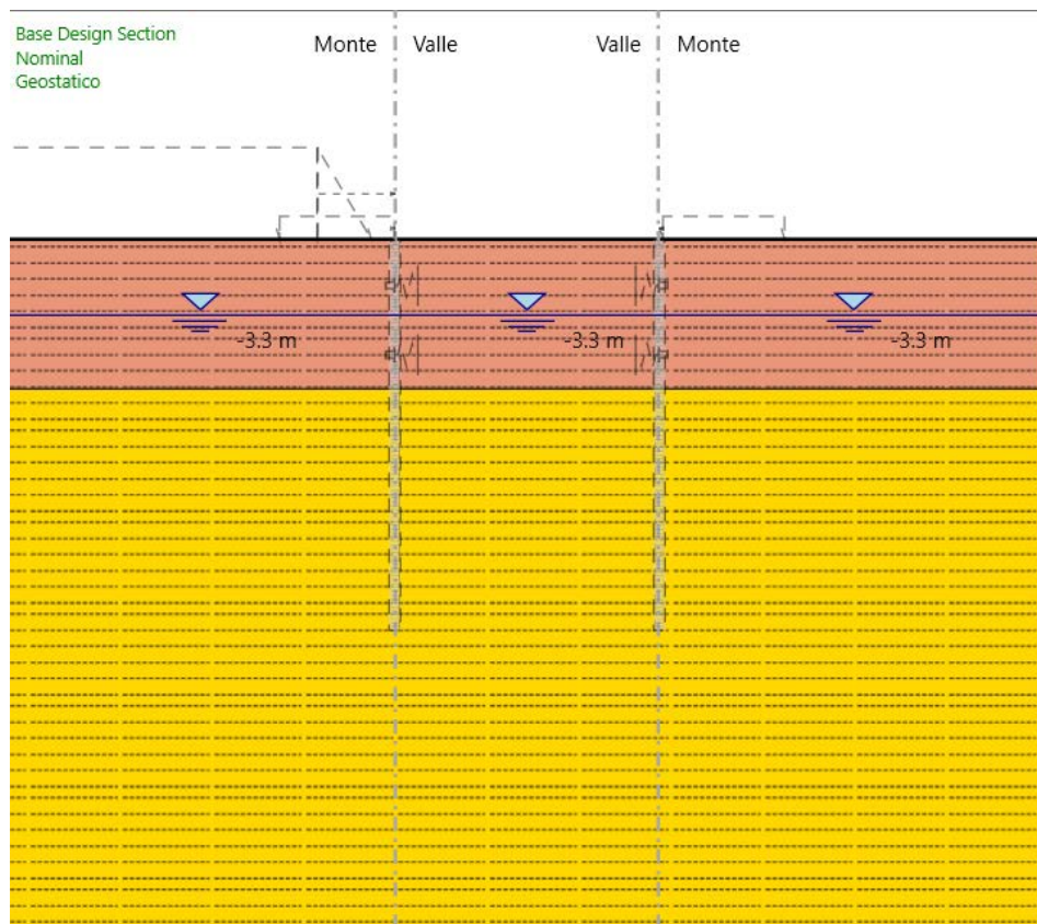
FASE 0: Generazione stato tensionale iniziale
