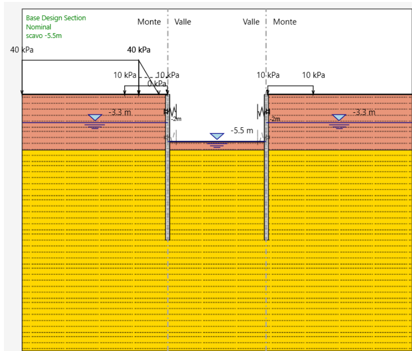
FASE 5: Scavo fino ad arrivare a 5.5m da p.c.
