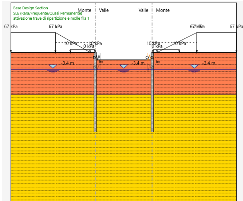
FASE 3: Installazione dei puntoni, con relative travi di ripartizione dei carichi, a 1.5 metri dalla testa della paratia
