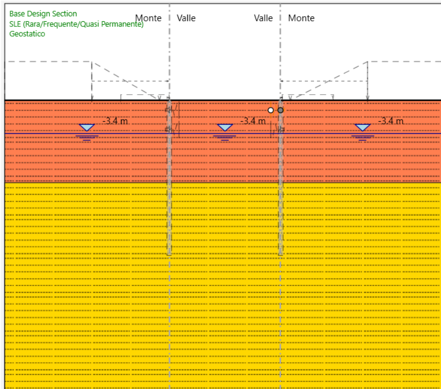
FASE 0: Generazione stato tensionale iniziale
