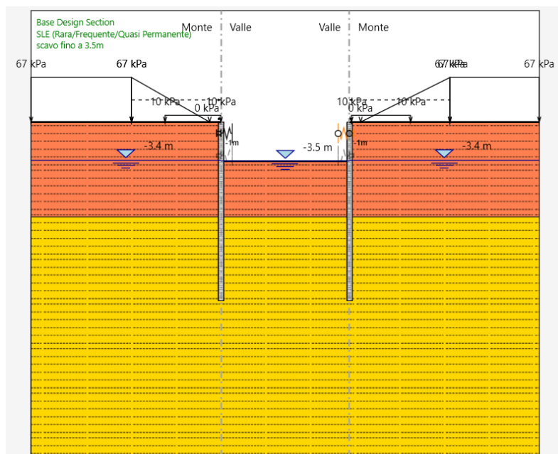
FASE 5: Scavo fino ad arrivare a 3.5 m da p.c.
