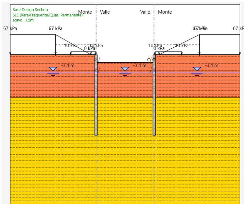
FASE 2: Scavo fino a arrivare a 1.5 m dal p.c.
