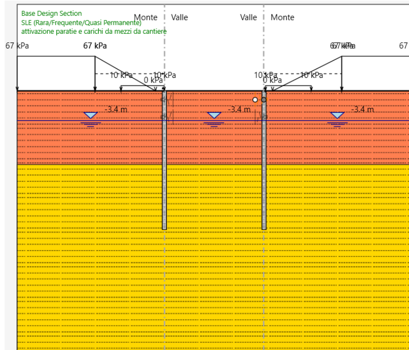
FASE 1: Installazione delle paratie di pali + attivazione carico di cantiere q_{acc}=10.0 kPa + attivazione carico trapezoidale che simula il p.c.
