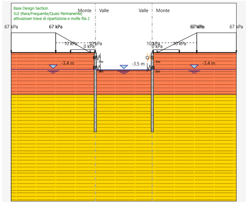
FASE 6: Installazione dei puntoni, con relative travi di ripartizione dei carichi, a 3.5 metri dalla testa della paratia
