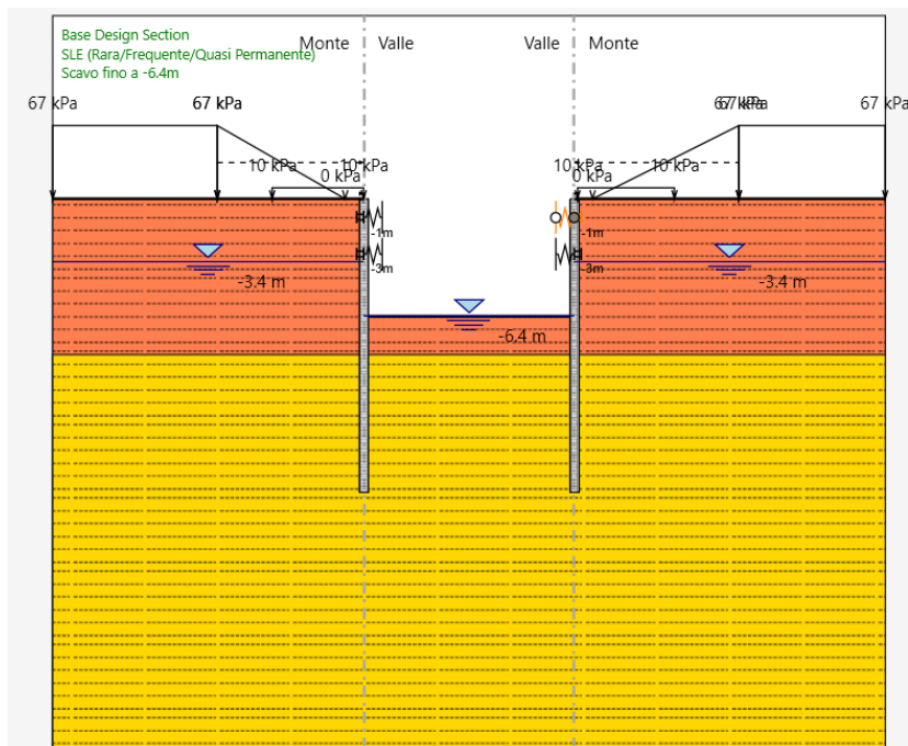
FASE 7: Scavo fino ad arrivare a 6.4 m da p.c.
