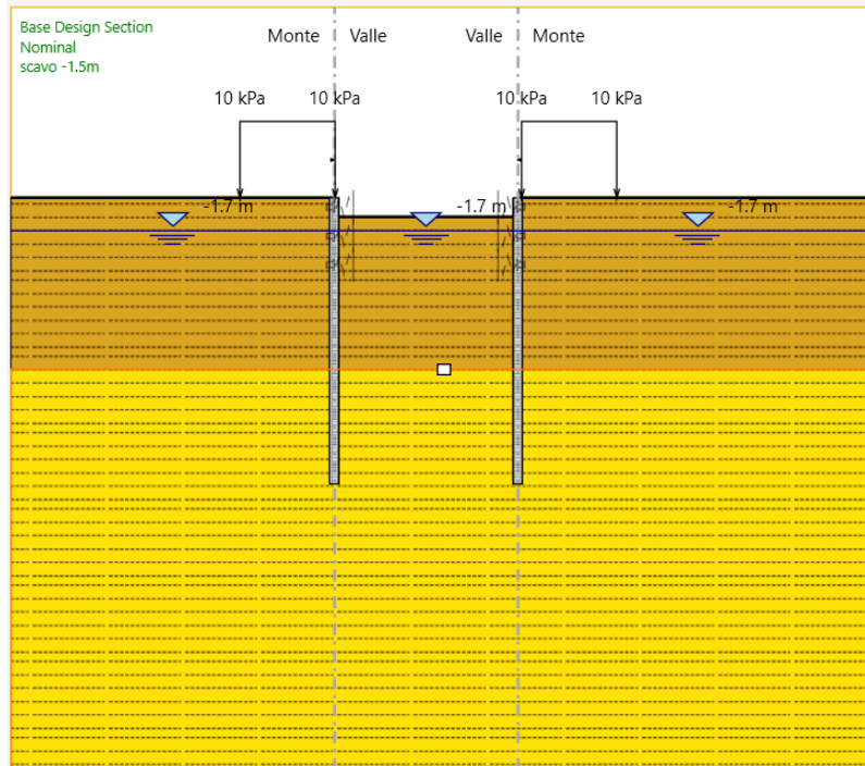
FASE 2: Scavo fino a arrivare a 1.5 m dal p.c.
