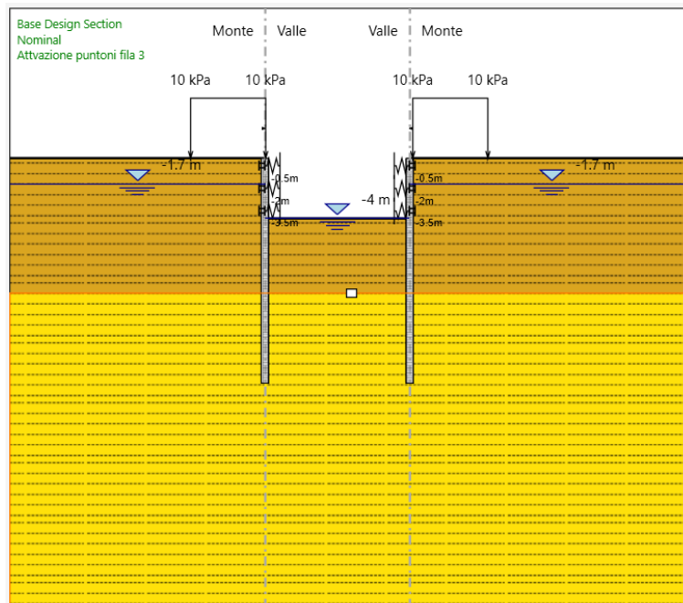
FASE 6: Scavo fino ad arrivare a 4m da p.c.
