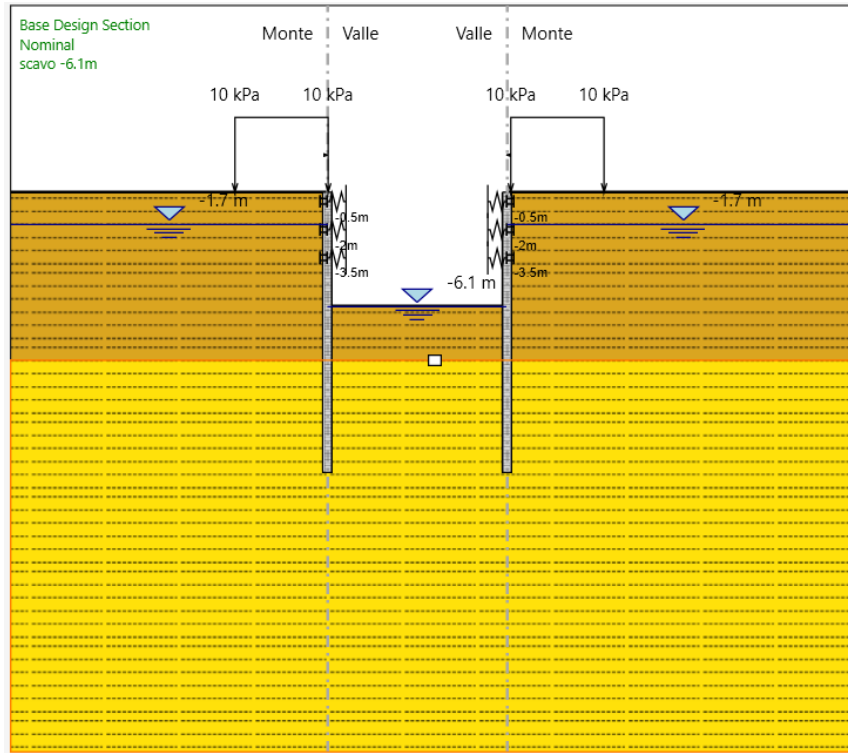
FASE 8: Scavo fino ad arrivare a 6.1 m da p.c.
