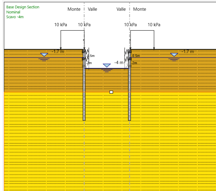
FASE 6: Scavo fino ad arrivare a 4m da p.c.
