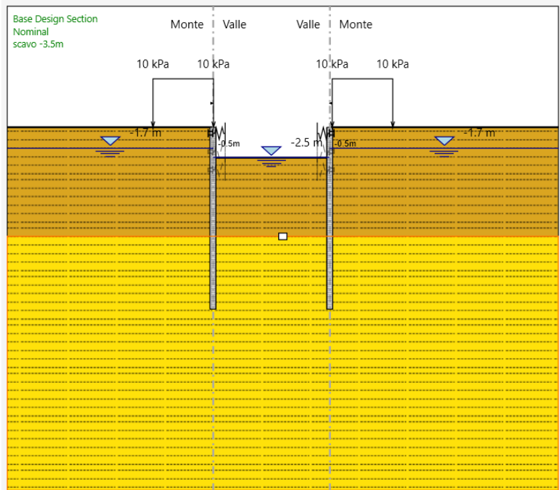
FASE 4: Scavo fino ad arrivare a 2.5m da p.c.
