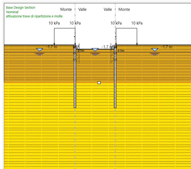
FASE 3: Installazione dei puntoni, con relative travi di ripartizione dei carichi, a 0.5 metri dalla testa della paratia
