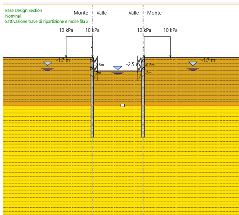
FASE 5: Installazione dei puntoni, con relative travi di ripartizione dei carichi, a 2 metri dalla testa della paratia
