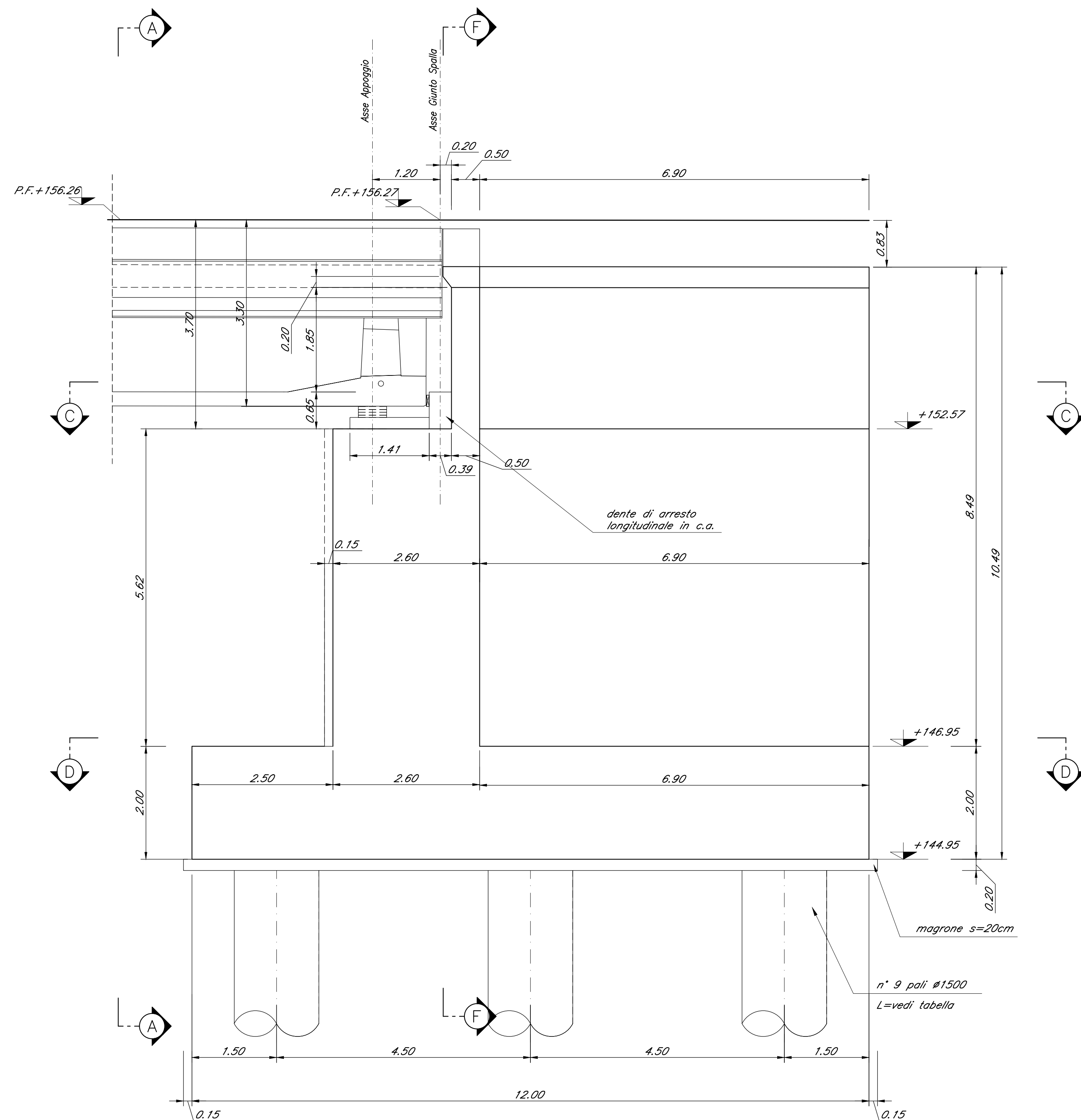
SEZIONE E-E Scala 1:50
