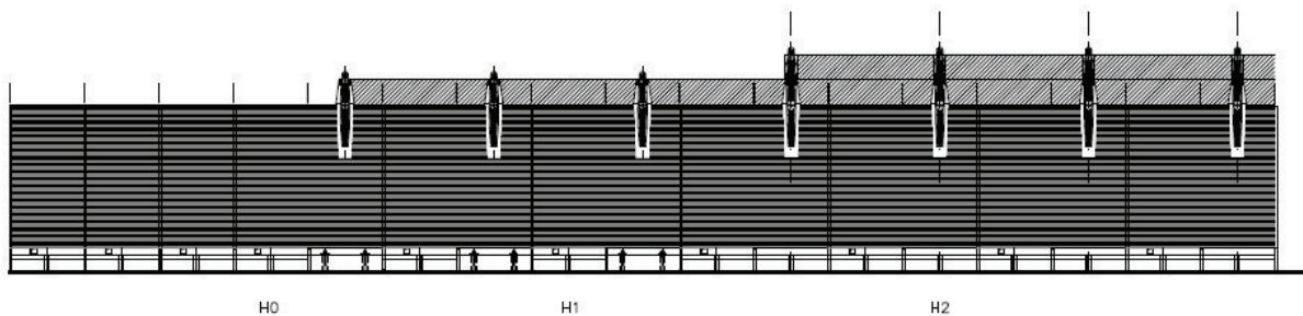
Sezioni-tipo dei moduli di barriera antirumore previsti nello Studio Acustico
