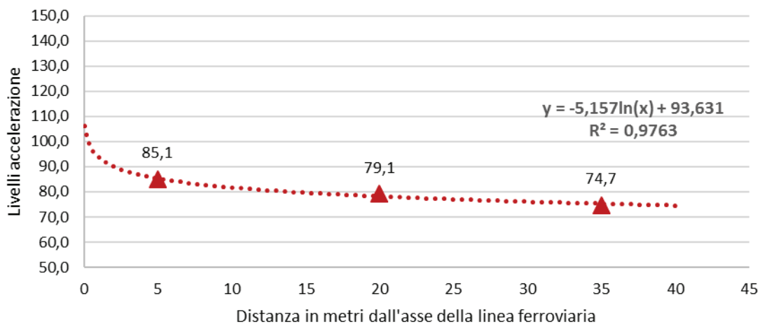
Figura 5 Curva di attenuazione del Leq_{te} in funzione della distanza dal binario, ricavata dai rilievi lungo l'asse Z, in corrispondenza della Terna 1 (5 metri), della Terna 2 (20 metri) e della Terna 3 (35 metri).
