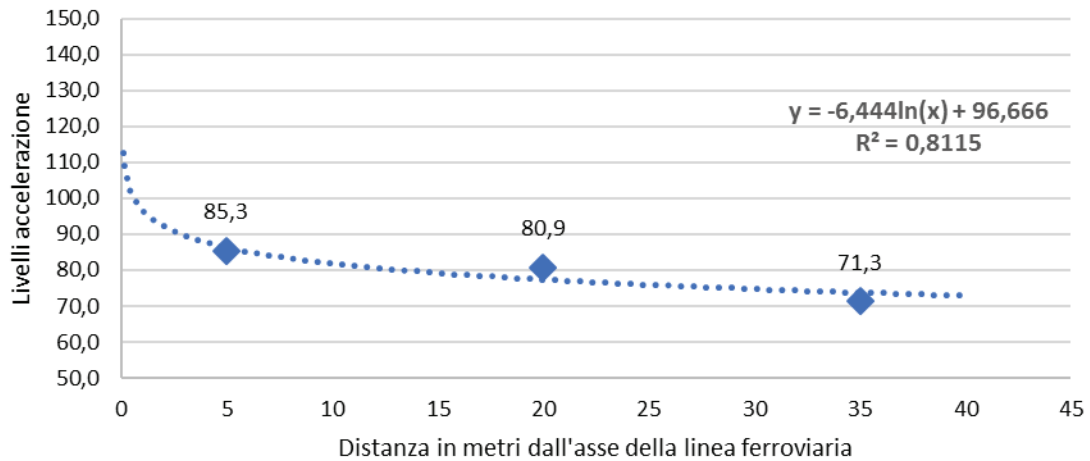
Figura 3 Curva di attenuazione del Leq,te in funzione della distanza dal binario, ricavata dai rilievi lungo l'asse X, in corrispondenza della Terna 1 (5 metri), della Terna 2 (20 metri) e della Terna 3 (35 metri).
