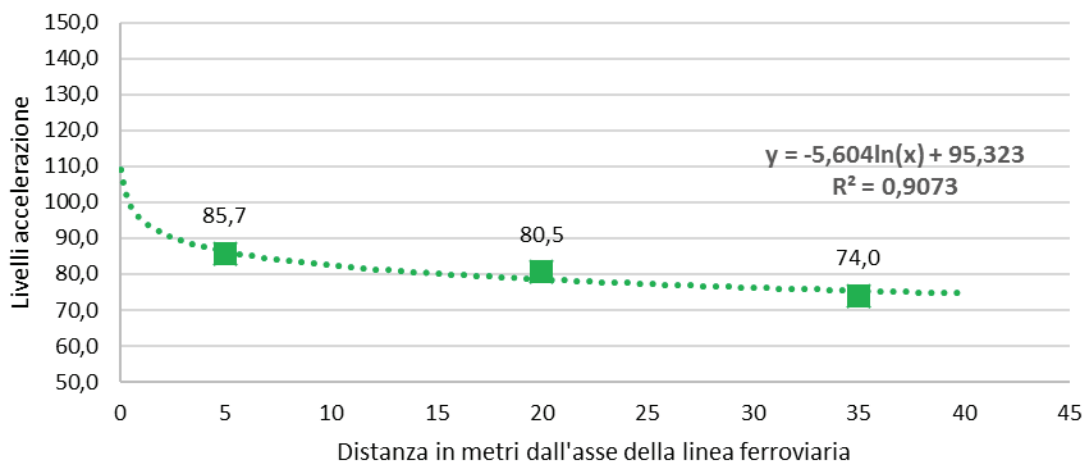
Figura 4 Curva di attenuazione del Leq_{te} in funzione della distanza dal binario, ricavata dai rilievi lungo l'asse Y, in corrispondenza della Terna 1 (5 metri), della Terna 2 (20 metri) e della Terna 3 (35 metri).
