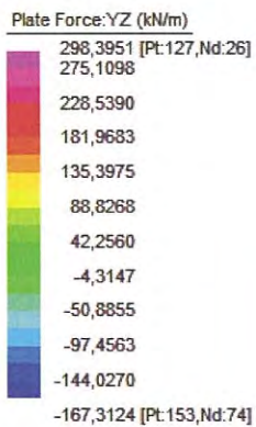
Figura 16 – Diagramma taglio piano verticale combinazione SLU
