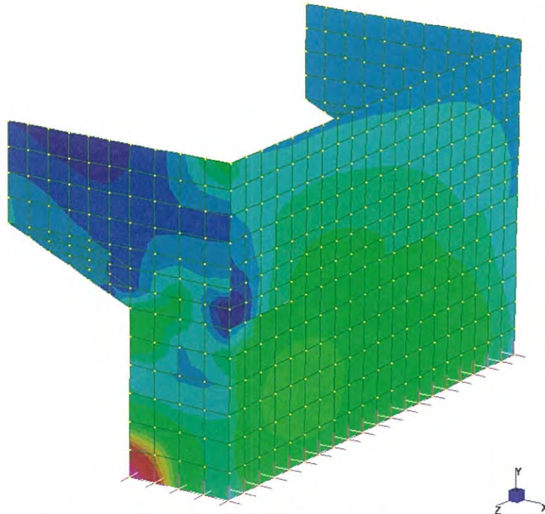
Figura 16 – Diagramma taglio piano verticale combinazione SLU
