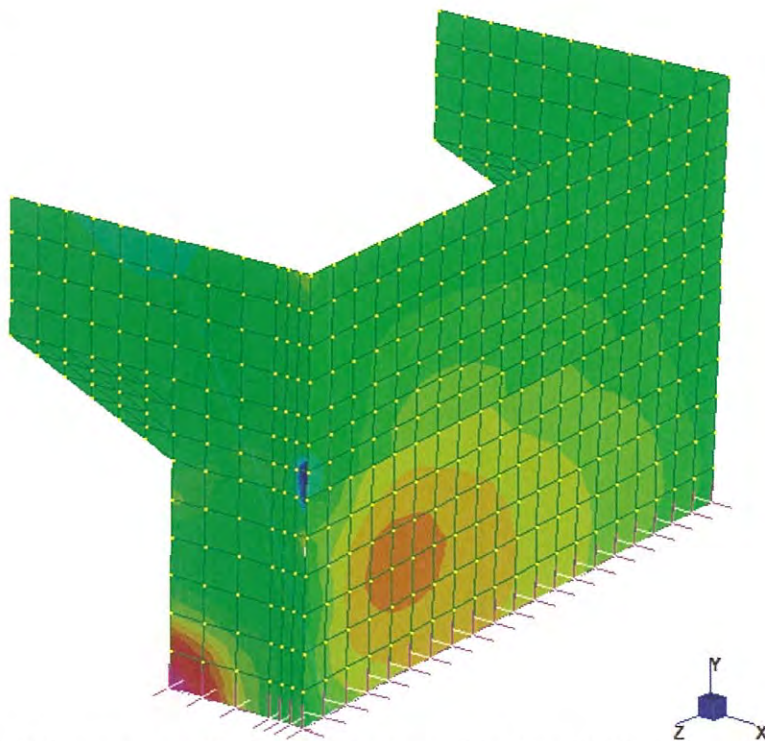
Figura 17 – Diagramma taglio piano verticale combinazione SLV
