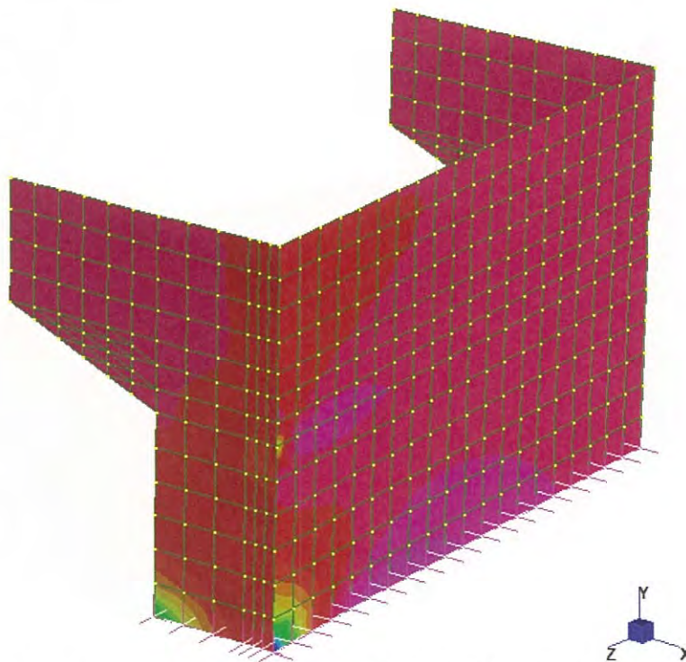
Figura 12 – Diagramma momento flettente piano verticale combinazione SLV
