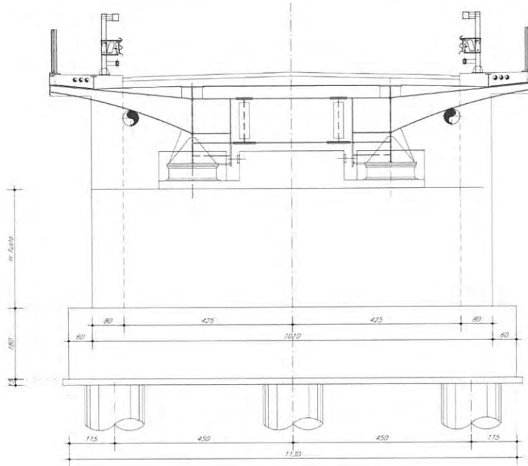
Figura 1 - Vista frontale
