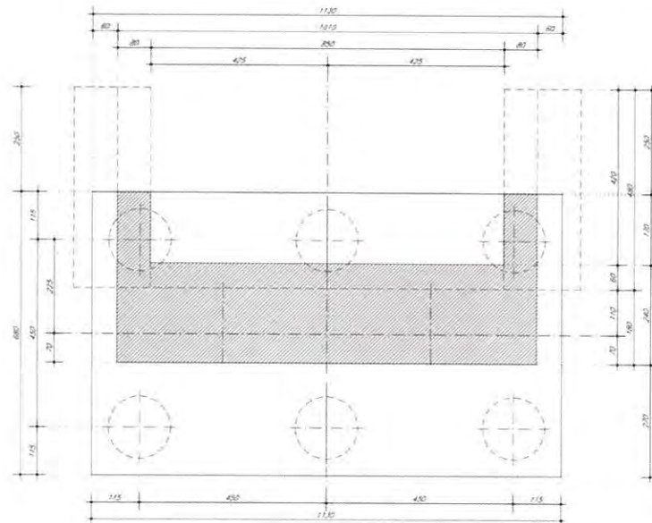
Figura 3 – Pianta fondazione e spiccato elevazione
